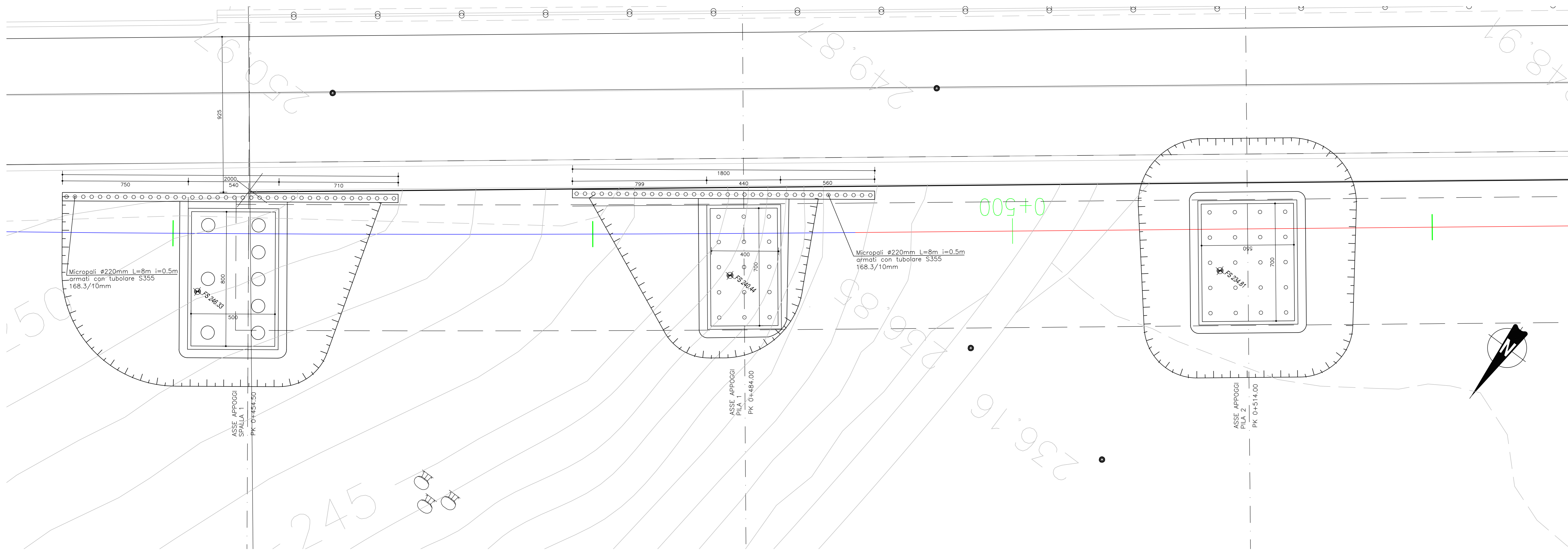
PIANTA STRALCIO 1 SCALA 1:100
