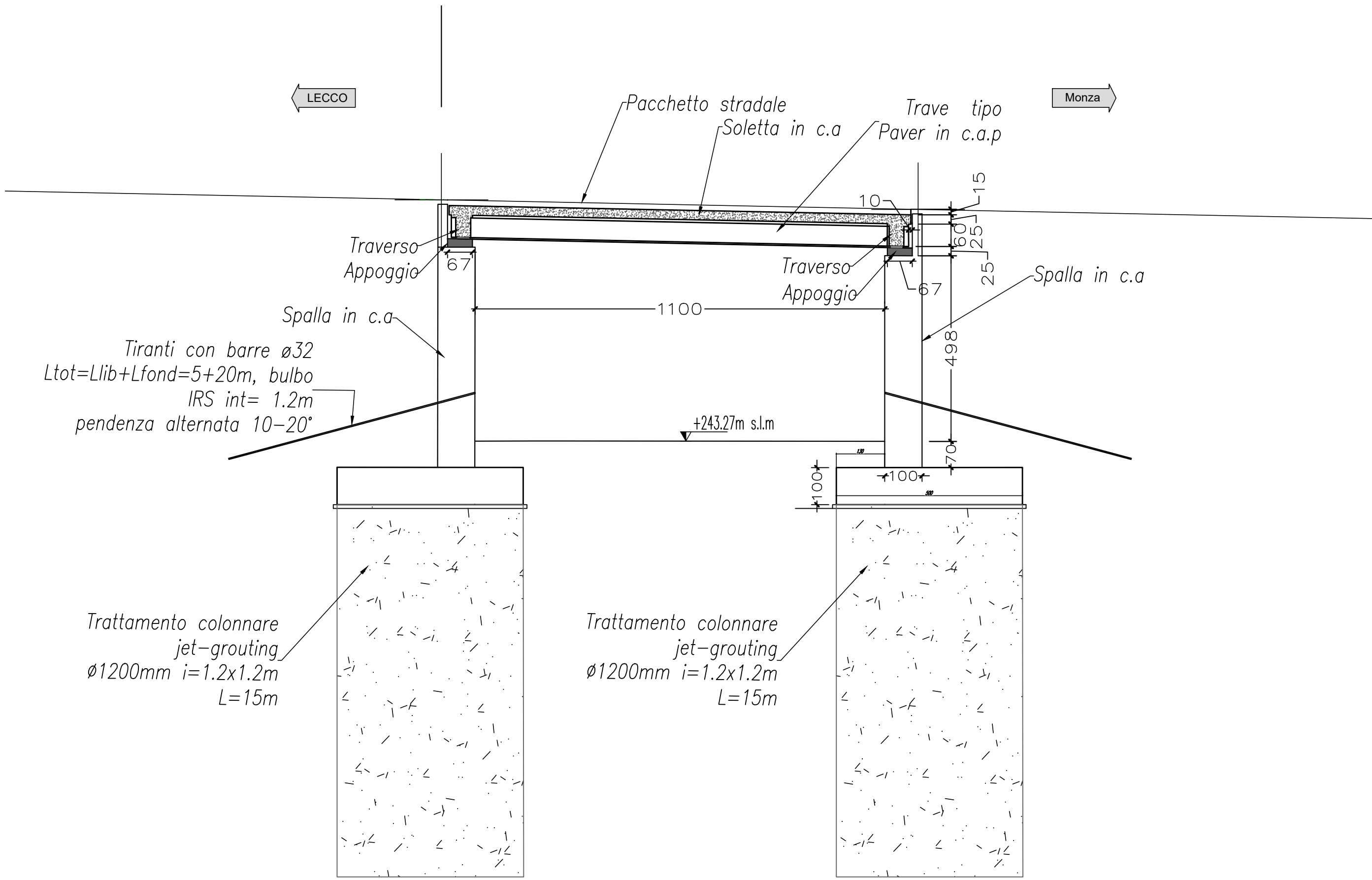
SEZIONE TRASVERSALE B-B' Scala 1:100
