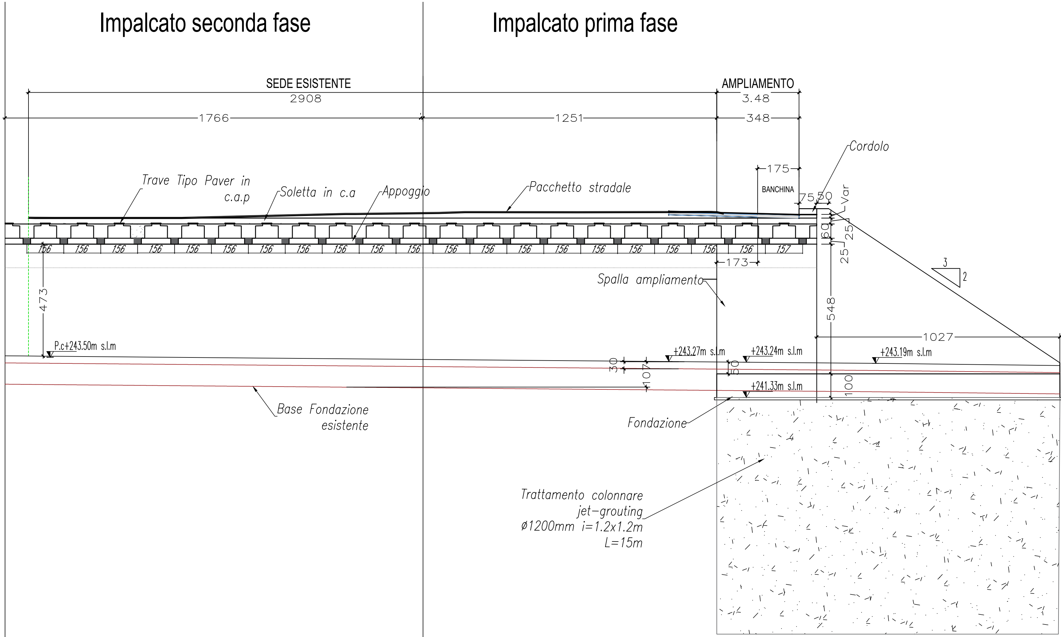
SEZIONE LONGITUDINALE A-A' SCALA 1:100
