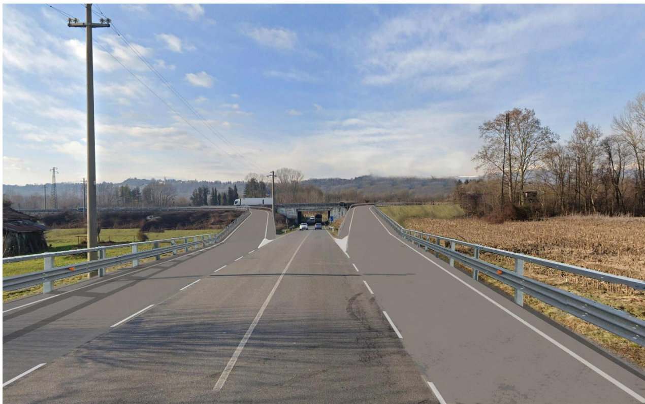
Figura 20: Vista da via Giuseppe Verdi verso i nuovi svincoli – FOTOSIMULAZIONE
