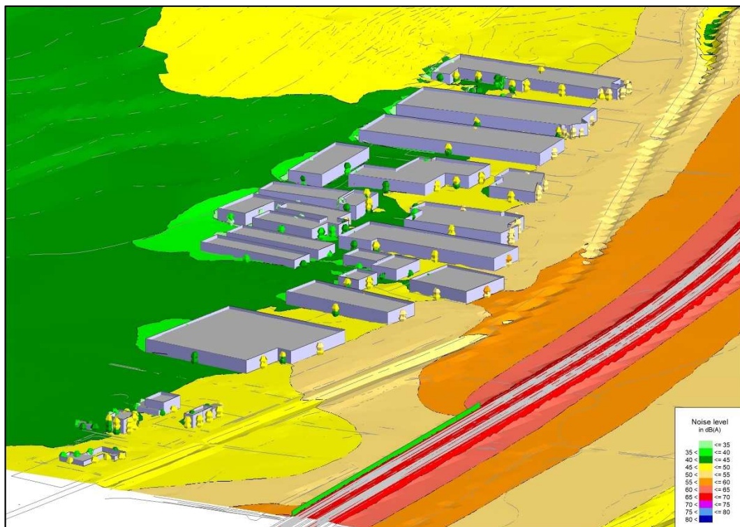
Figura 5.8.C – Vista 3D mappa impatto mitigato notturno (Leq 22-6) area fine lotto
