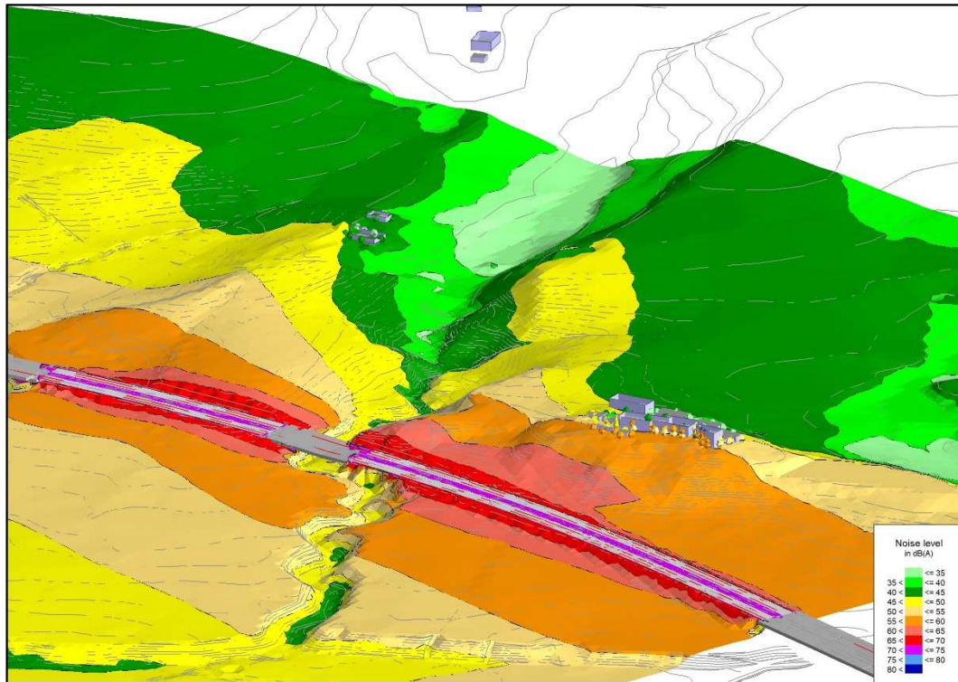
Figura 5.6.A – Vista 3D mappa impatto notturno (Leq 22-6) area Cascina Spià
