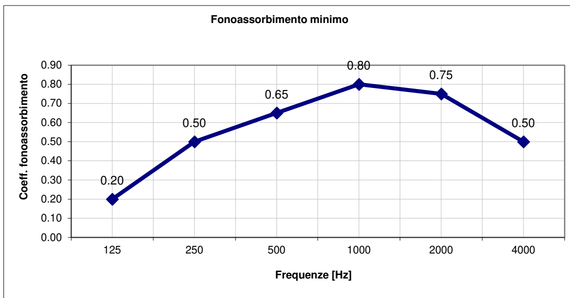
Figura 5.7.A – Curva di fonoassorbimento minimo dei pannelli fonoassorbenti
