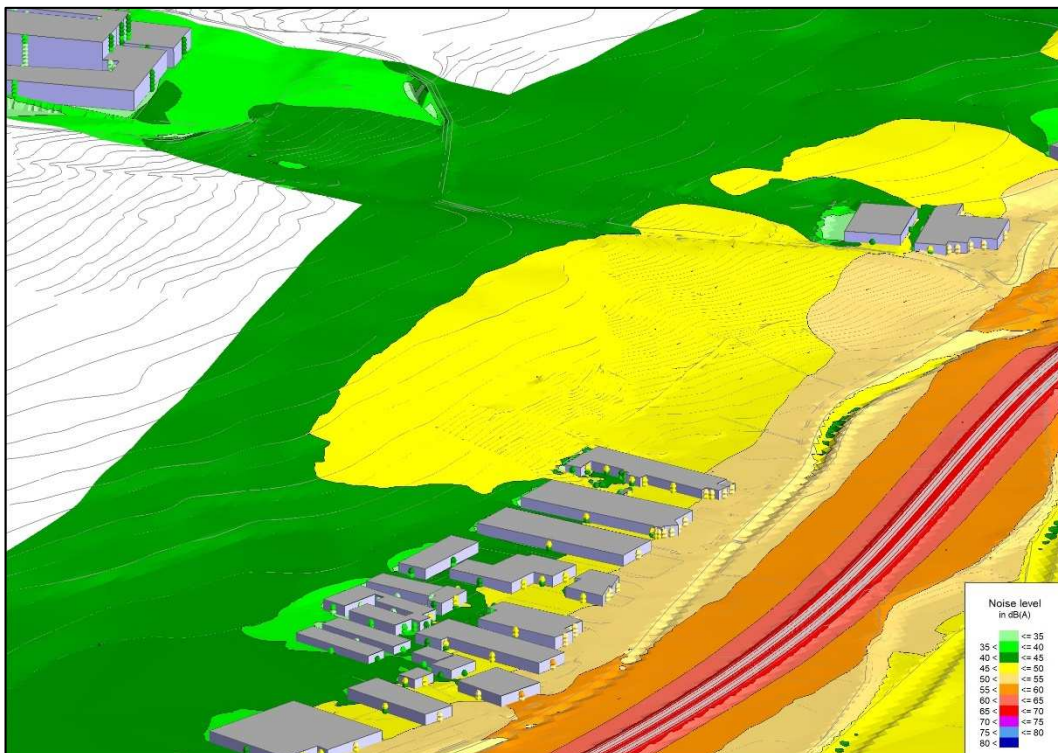
Figura 5.8.E – Vista 3D mappa impatto mitigato notturno (Leq 22-6) area Ospedale di Alba-Bra
