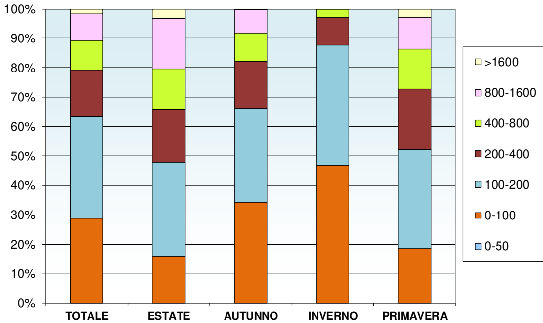
Figura 3.K Altezza di rimescolamento
