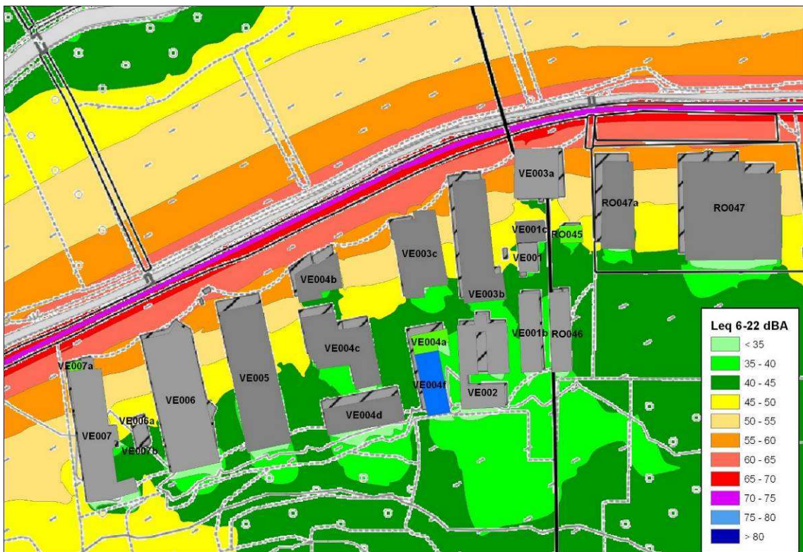
Figura. 4.7.B – Mappatura acustica viabilità di cantiere aree industriale Verduno-Roddi
