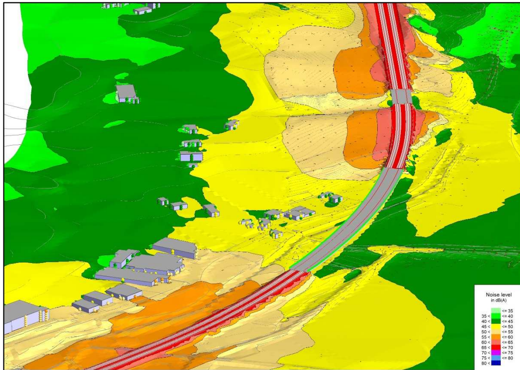
Figura 5.8.B – Vista 3D mappa impatto mitigato notturno (Leq 22-6) area viadotto Verduno
