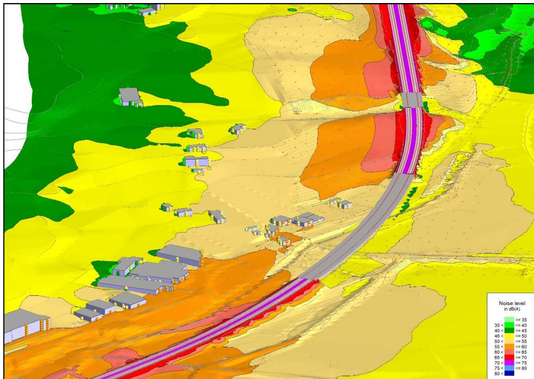
Figura 5.6.B – Vista 3D mappa impatto notturno (Leq 22-6) area viadotto Verduno
