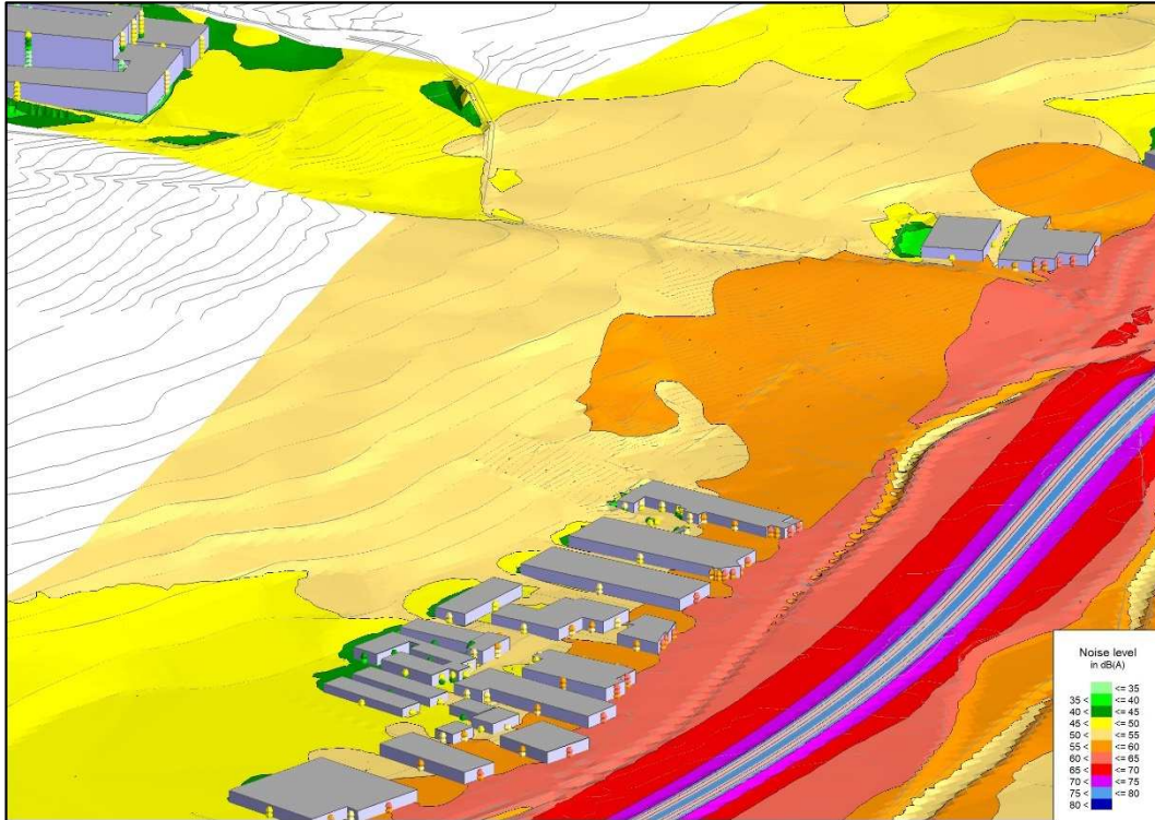
Figura 5.8.D – Vista 3D mappa impatto mitigato diurno (Leq 6-22) area Ospedale di Alba-Bra
