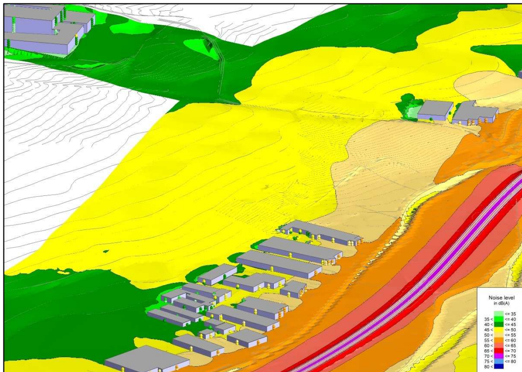
Figura 5.6.E – Vista 3D mappa impatto notturno (Leq 22-6) area Ospedale di Alba-Bra
