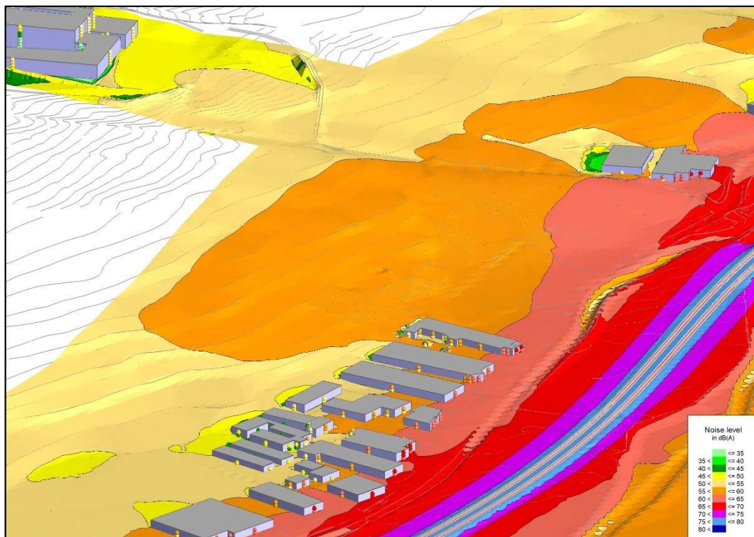
Figura 5.6.D – Vista 3D mappa impatto diurno (Leq 6-22) area Ospedale di Alba-Bra
