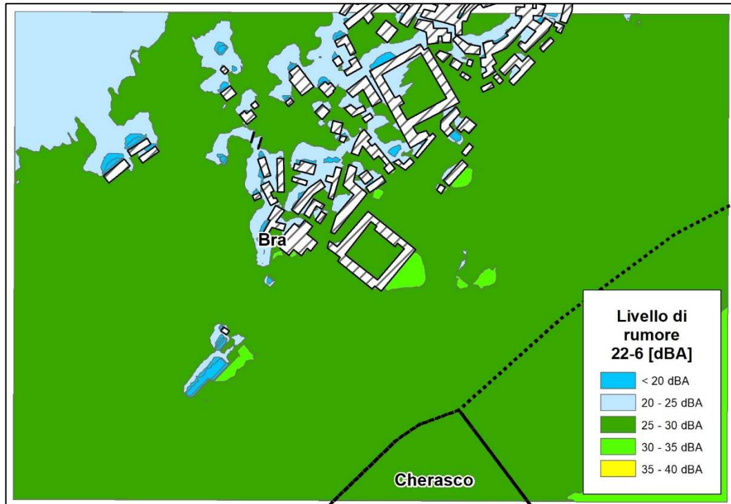
Figura 5.8.G – Esposizione acustica del Castello Reale di Pollenzo – Periodo notturno
