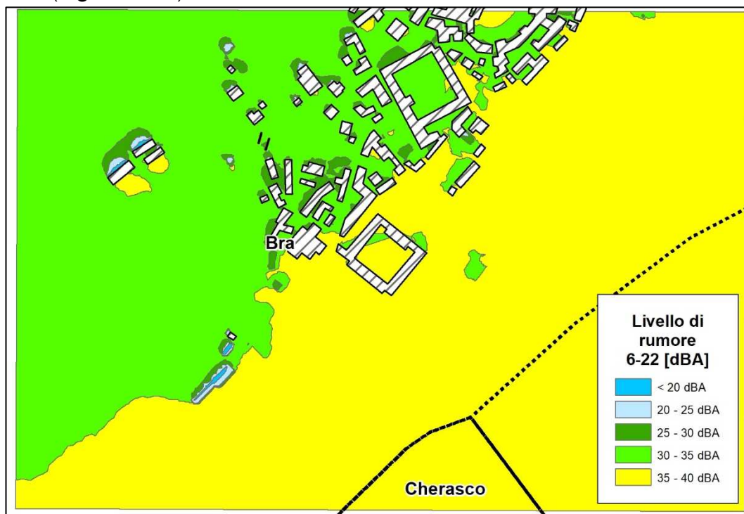
Figura 5.8.F – Esposizione acustica del Castello Reale di Pollenzo – Periodo diurno
