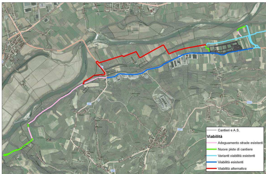
Figura. 4.4.A – Viabilità di cantiere
