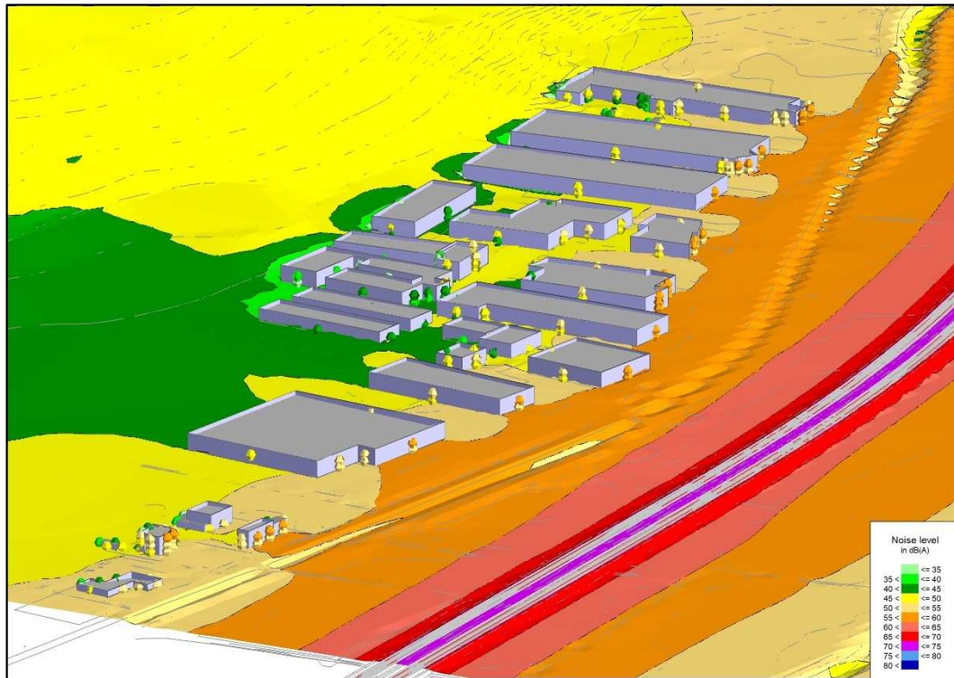
Figura 5.6.C – Vista 3D mappa impatto notturno (Leq 22-6) area fine lotto
