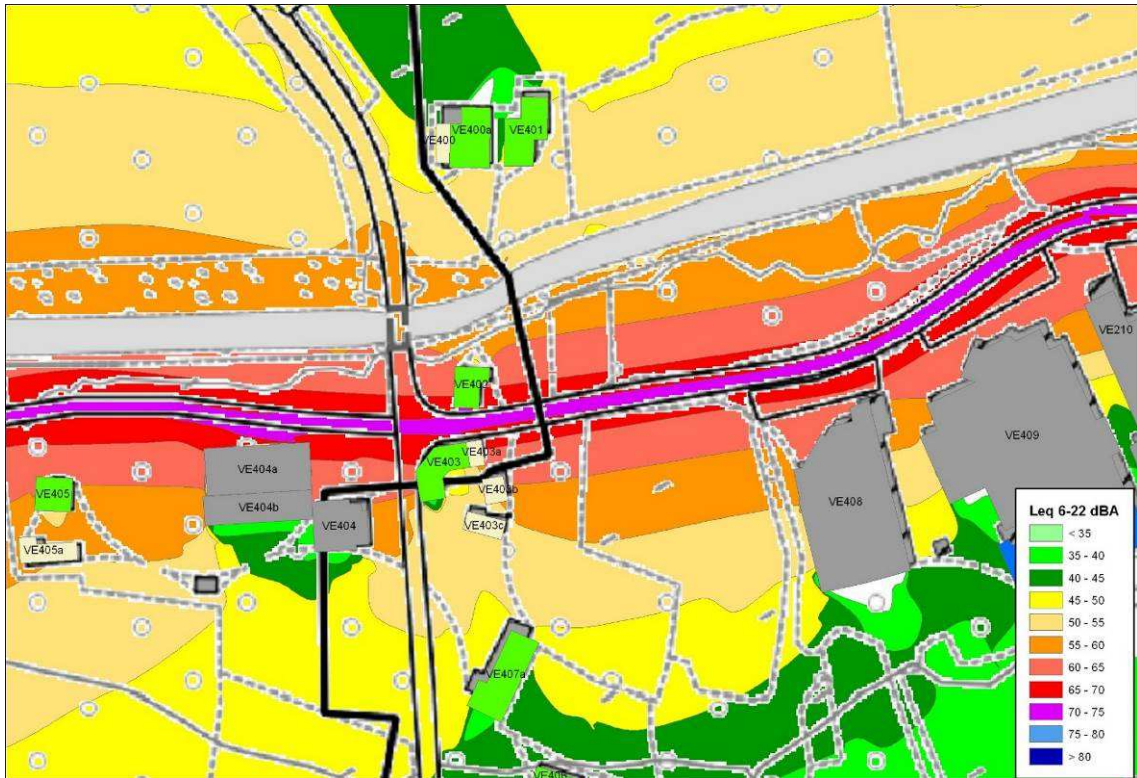
Figura. 4.7.A – Mappatura acustica viabilità di cantiere area La Morra-Verduno
