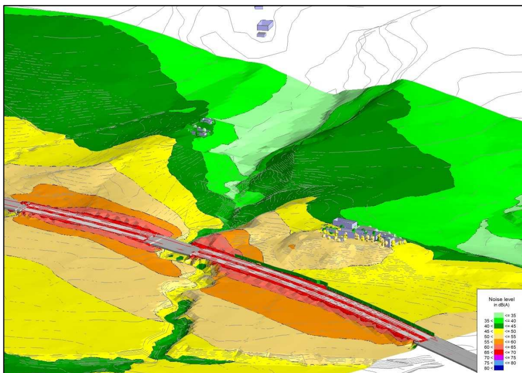
Figura 5.8.A – Vista 3D mappa impatto mitigato notturno (Leq 22-6) area Cascina Spià
