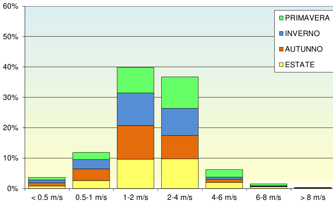
Figura 3.L Classi di velocità del vento
