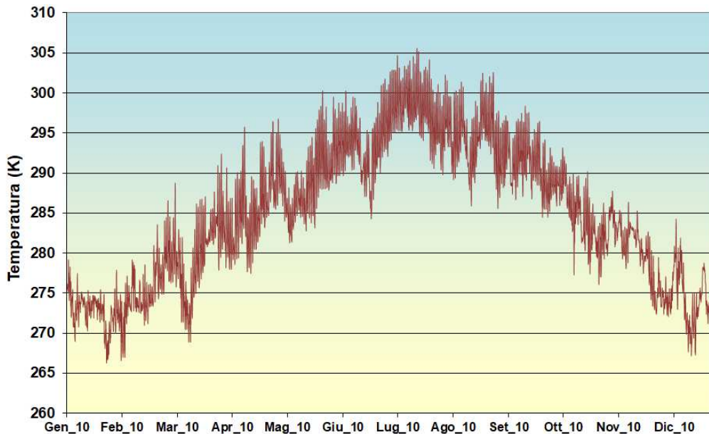
Figura 3.I Andamento della temperatura oraria in gradi Kelvin
