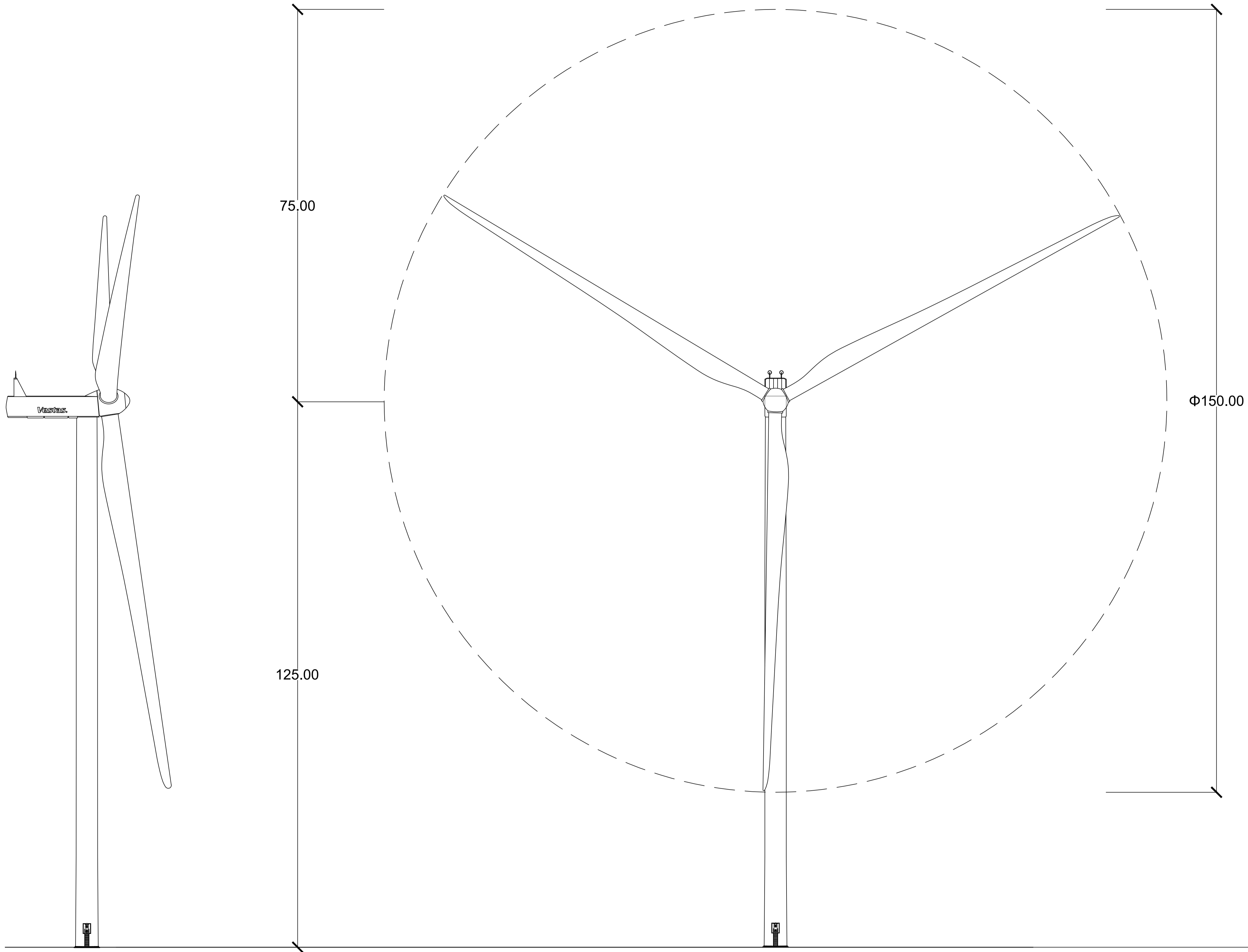
VISTA FRONTALE - SCALA 1:400
