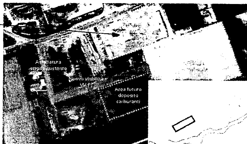
Figura 3-25 Area deposito carburanti e accessi.
