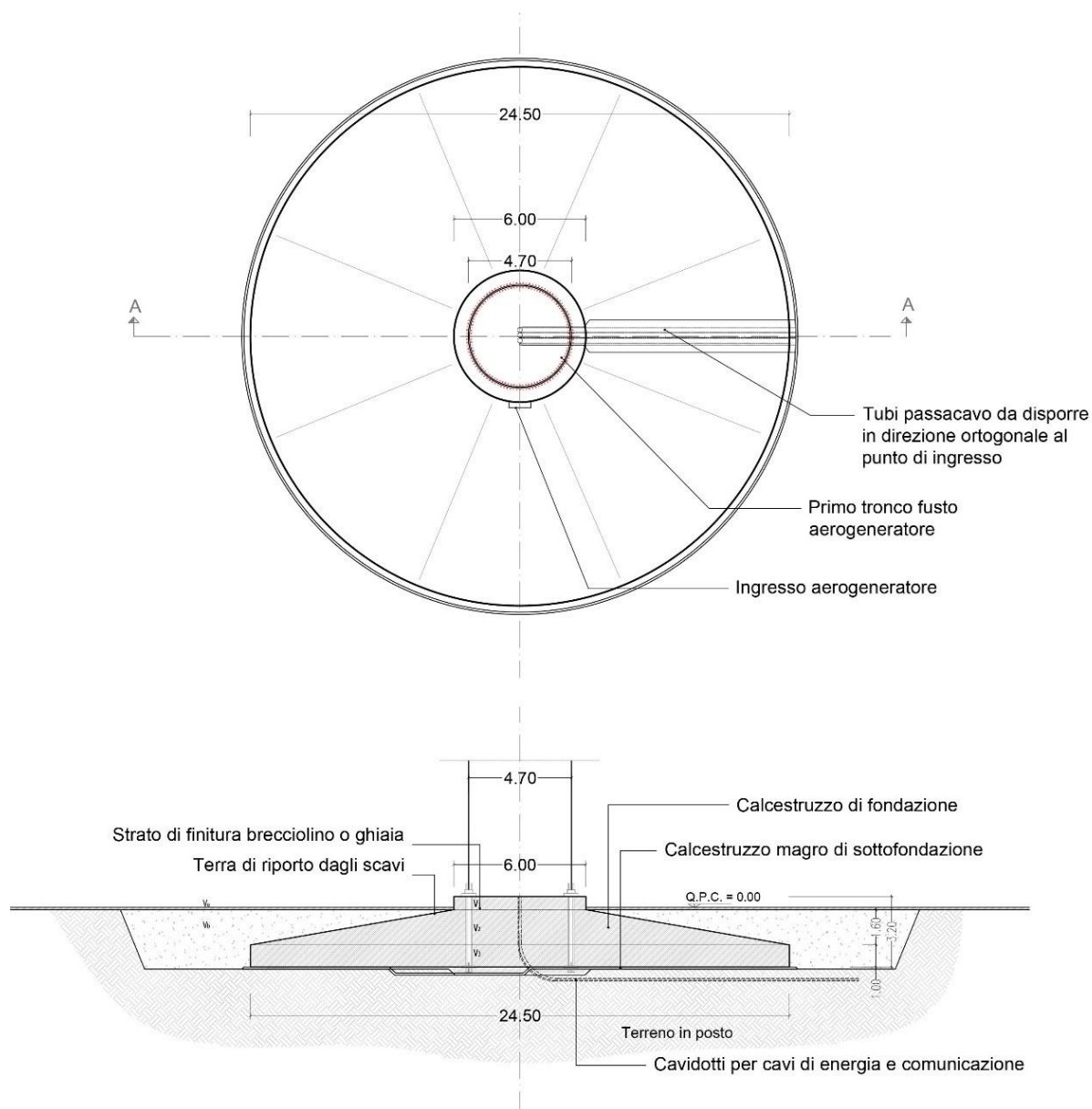
Figura 1 – Pianta e vista della fondazione tipo dell'aerogeneratore
