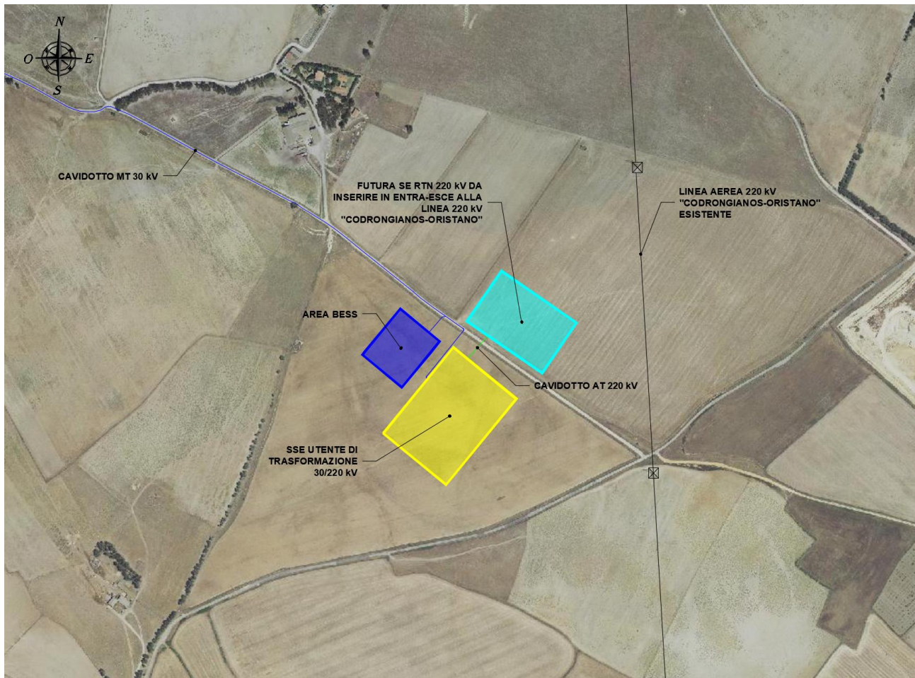
Figura 2.1 - Connessione Produttore Sorgenja Renewables S.r.l.
