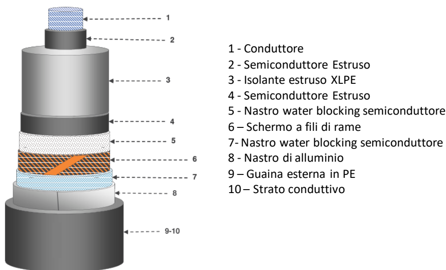
Figura 3.1 - Cavo AT 220 kV tipo ARE4H1H5E 220 kV
