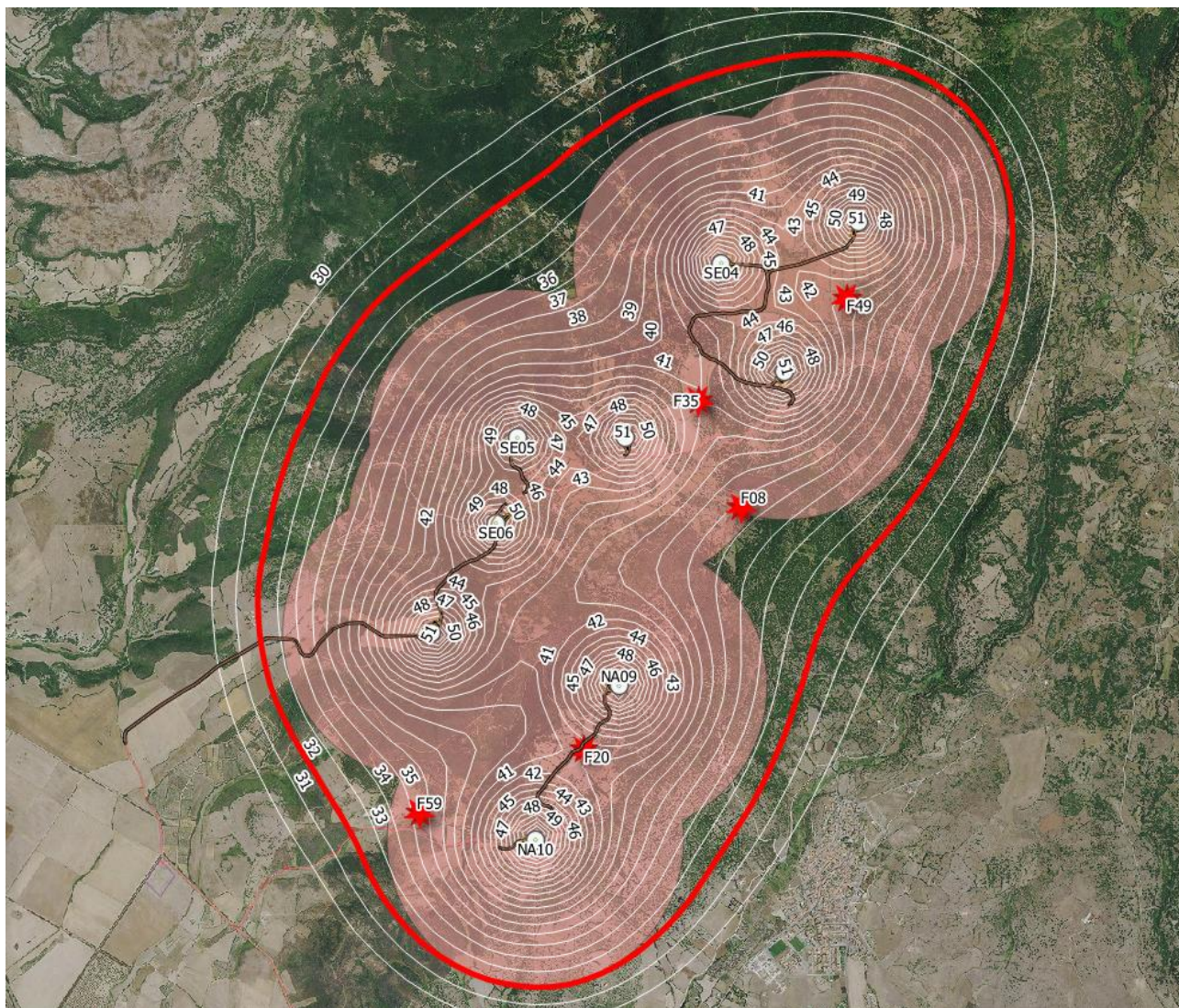
Figura 2.5 – Campo sonoro generato dall'impianto. In rosso l'isofonica dei 32 dBA, attestata ad una distanza indicativa di 1.000 m dalle postazioni eoliche in progetto
