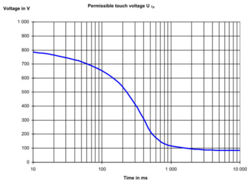
Figura 7.1: Massima tensione ammissibile (CEI EN 50522, Fig.4).
