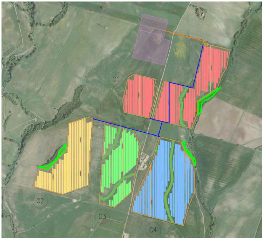
Figura 3.1: Layout di progetto
