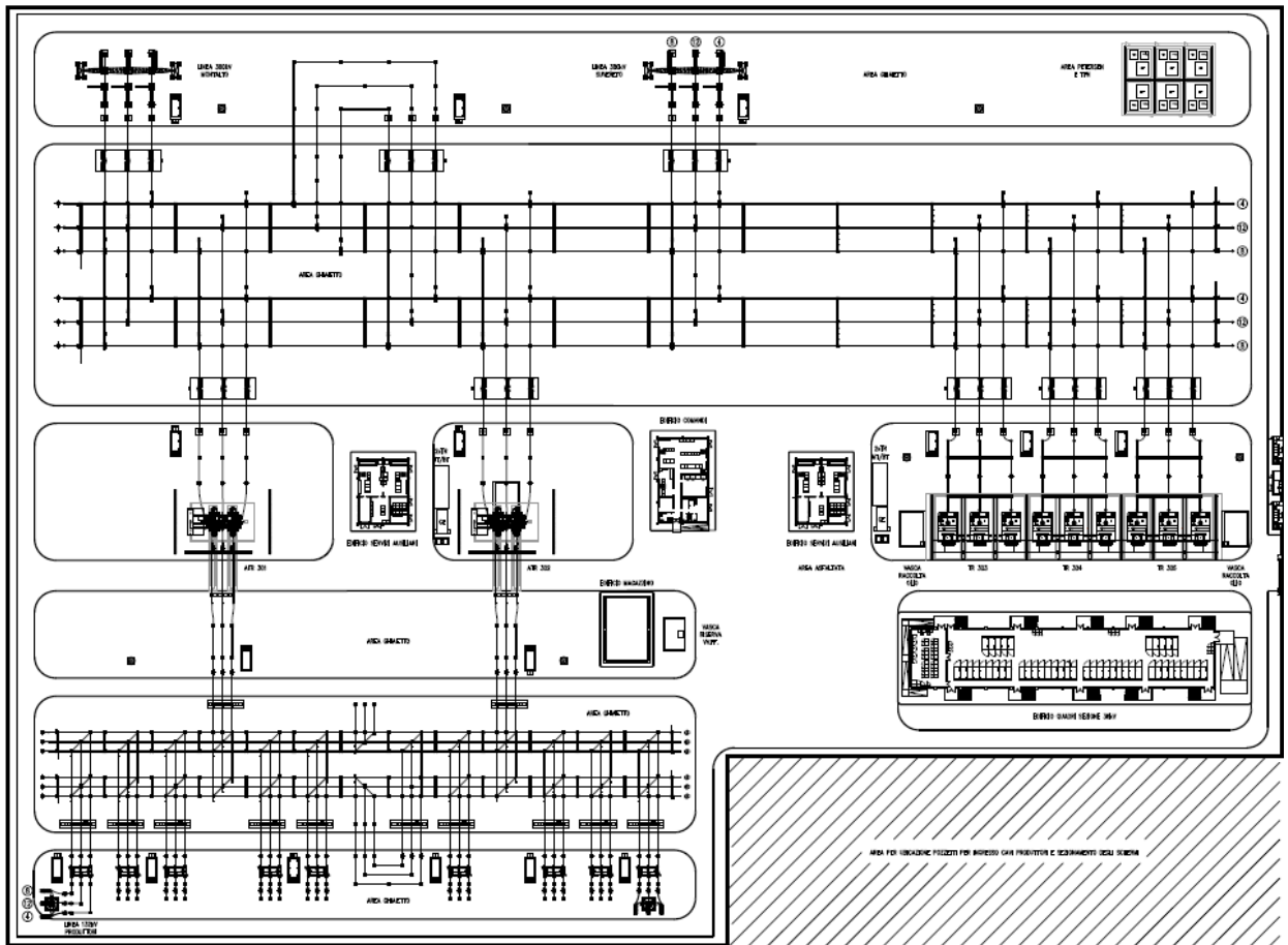
Figura 2.7: Planimetria reparto AT nuova SE 380/132/36 kV Manciano
