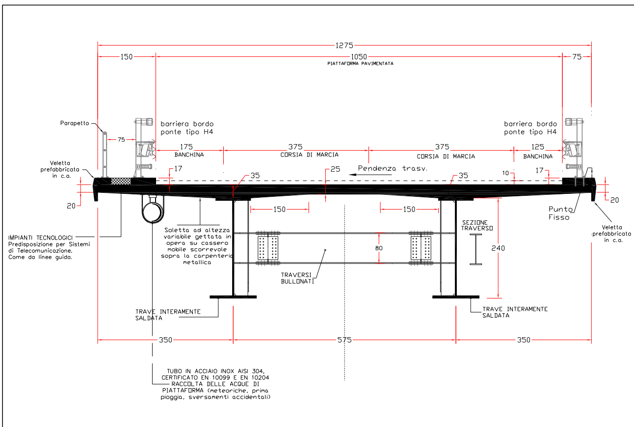
Sezione trasversale d'impalcato.
