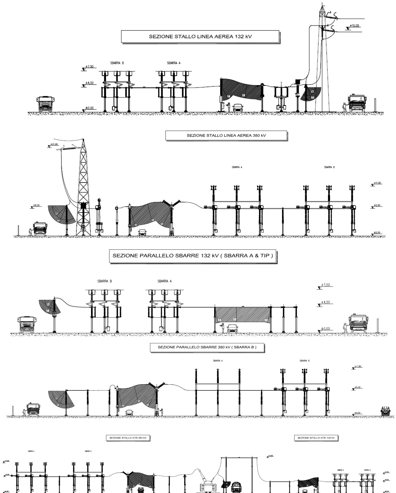
Figura 4 – Sezioni degli stalli linea e delle sbarre delle due sezioni 380 e 132 kV di una tipica stazione Terna
