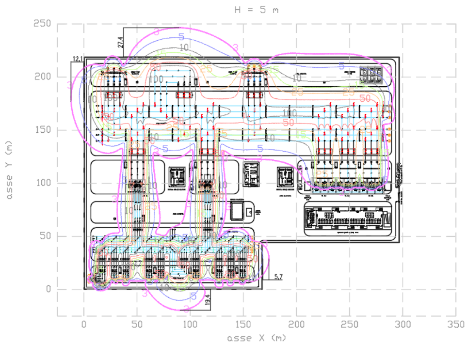
Figura 8 – Livelli di campo magnetico a 5 m dal piano della stazione
