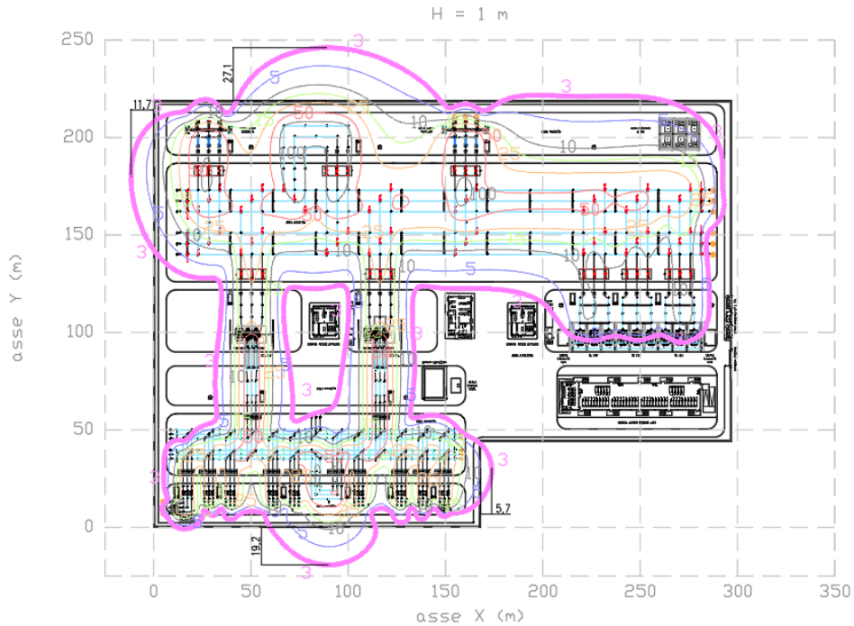
Figura 7 – Livelli di campo magnetico a 1 m dal piano della stazione
