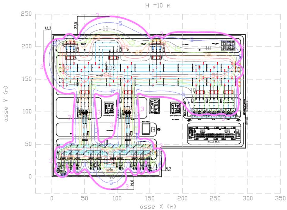
Figura 9 – Livelli di campo magnetico a 8 m dal piano della stazione
