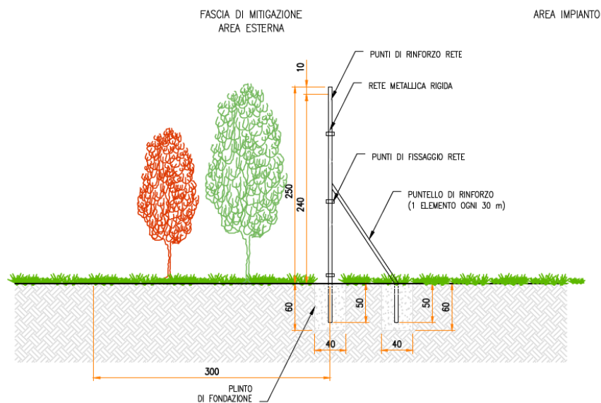
Figura 3.3: Particolari recinzione
