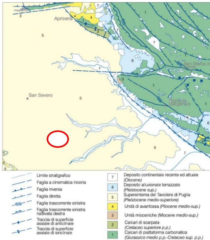
Figura 3:4 schema tettonico
