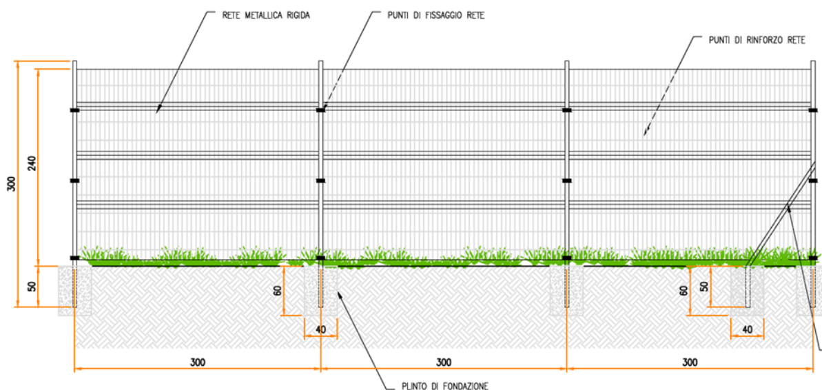
Figura 2.8: Particolare recinzione
