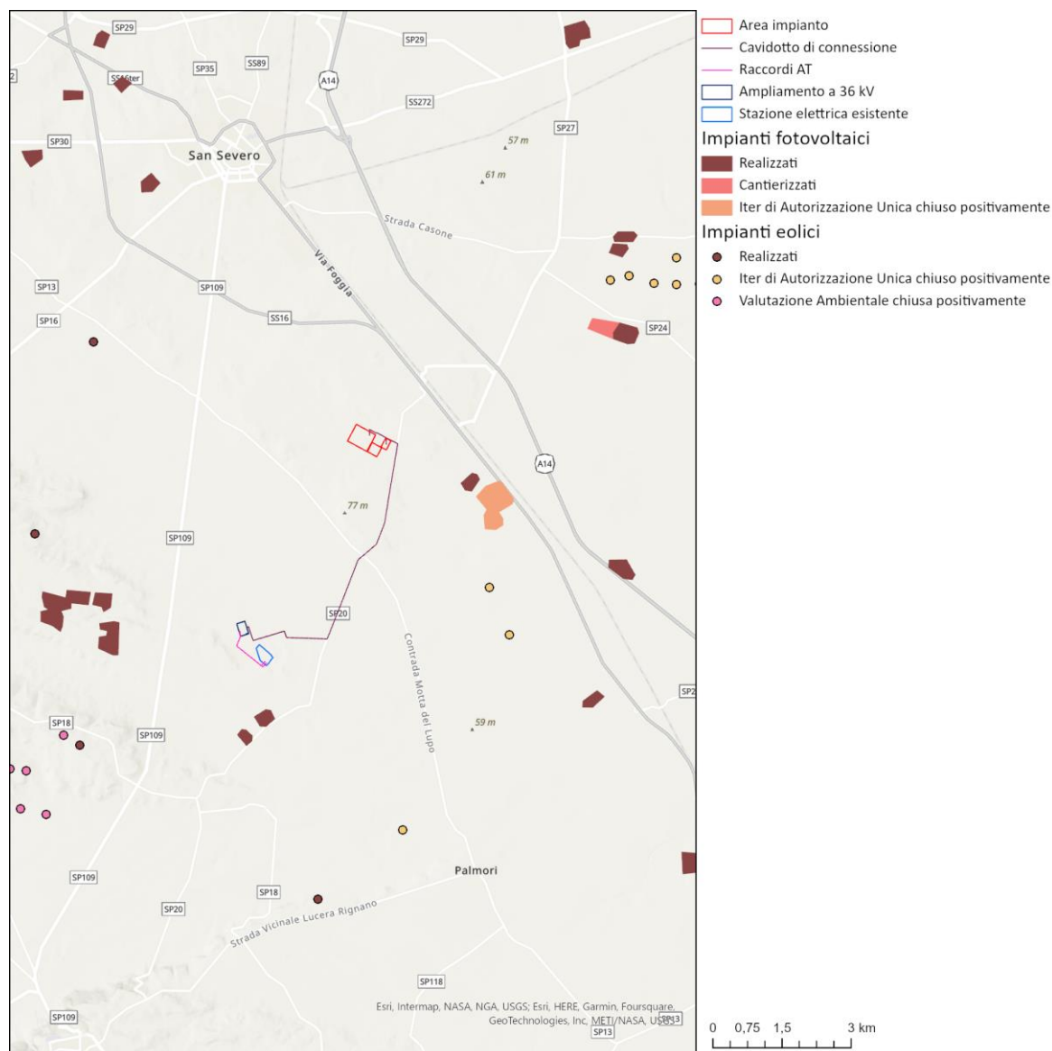
Figura 11.1: Impianto in progetto (in blu) e impianti fotovoltaici/eolici presenti nell'area oggetto di studio – Elaborazione Montana S.p.A.
