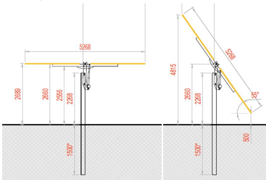
Figura 4.3: Particolare strutture di sostegno moduli
