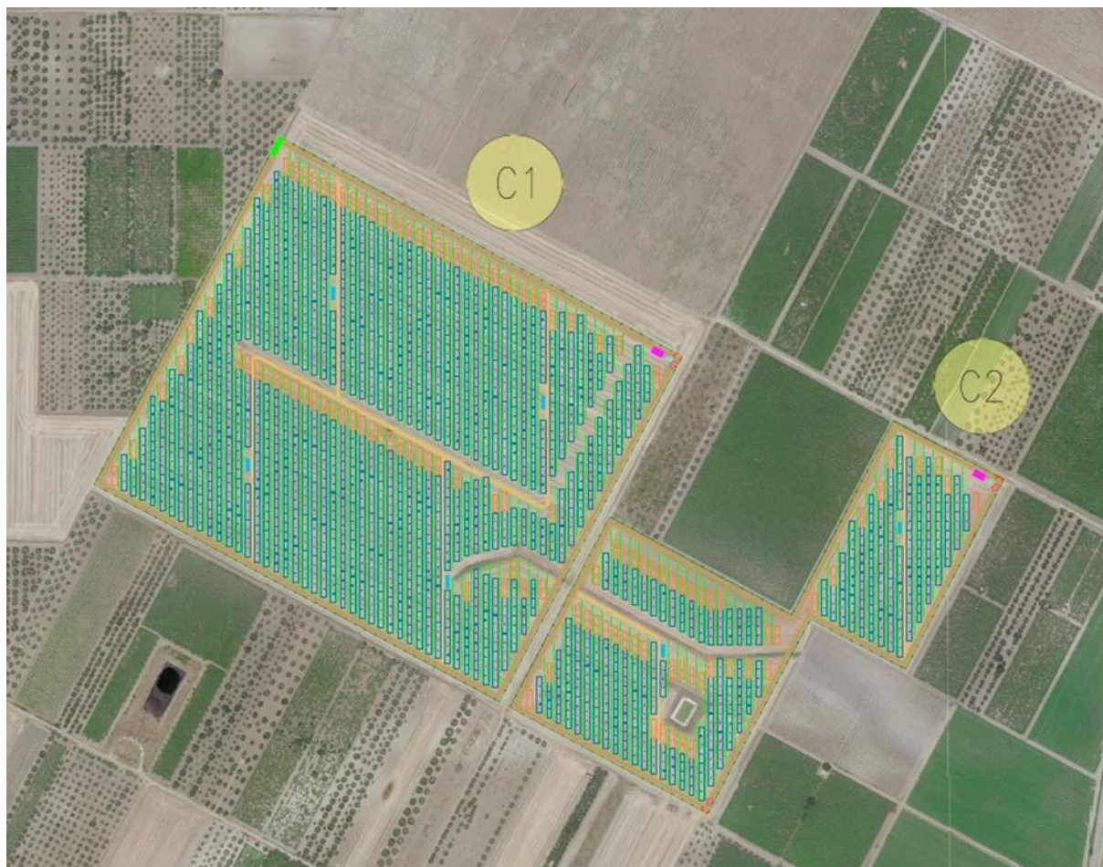
Figura 4.2: layout di impianto
