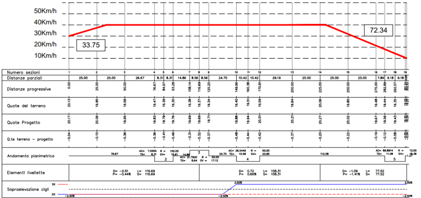
Diagramma velocità planimetrica – Ricucitura n.24
