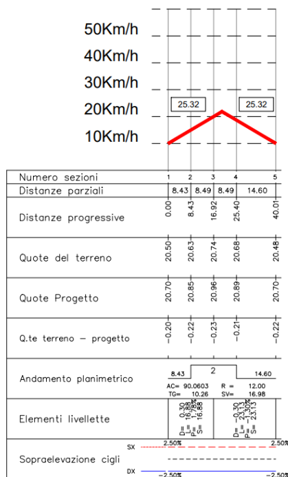
Diagramma velocità planimetrica – Ricucitura n.25
