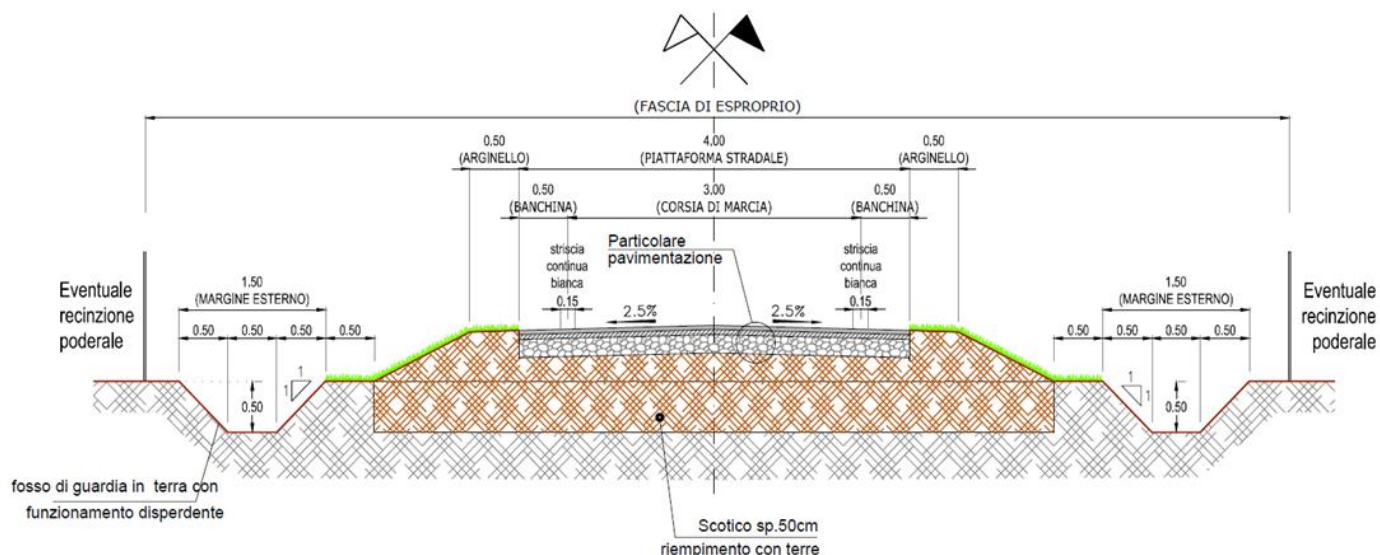
Figura 6.2 – Sezione tipo ricuciture: configurazione a schiena
