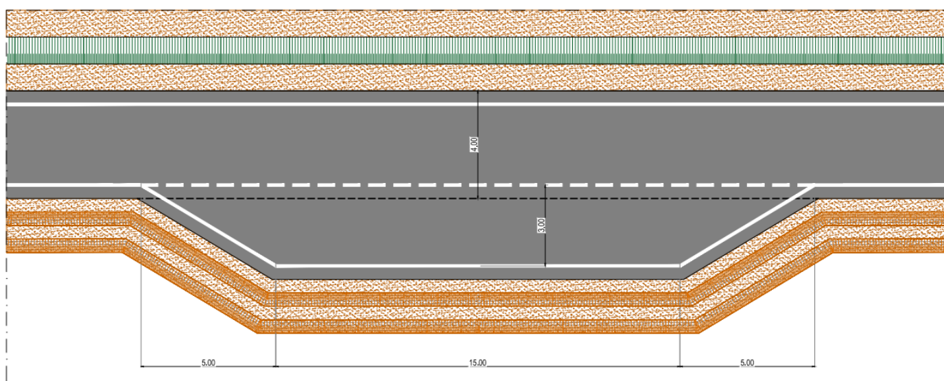
Figura 6.5 – Piazzole di precedenza
