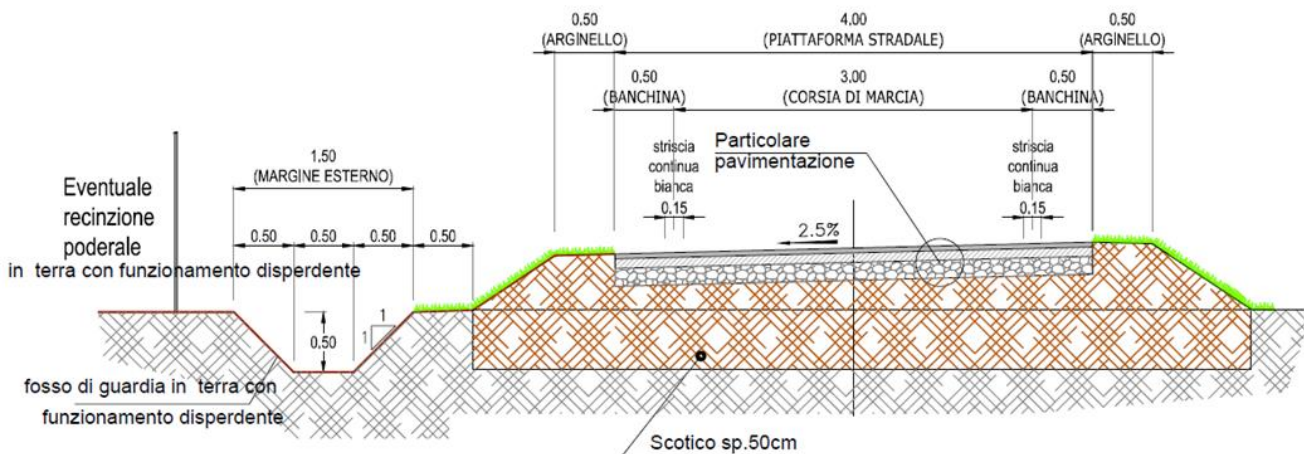
Figura 6.3 – Sezione tipo ricuciture: configurazione a tetto parallelo al rilevato stradale
