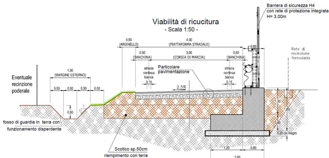
Figura 6.4 – Sezione tipo: configurazione a tetto parallela alla ferrovia con barriere di sicurezza
