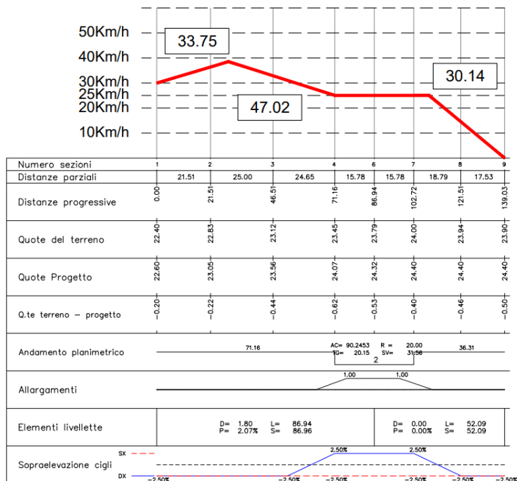
Diagramma velocità planimetrica – Ricucitura n.23
