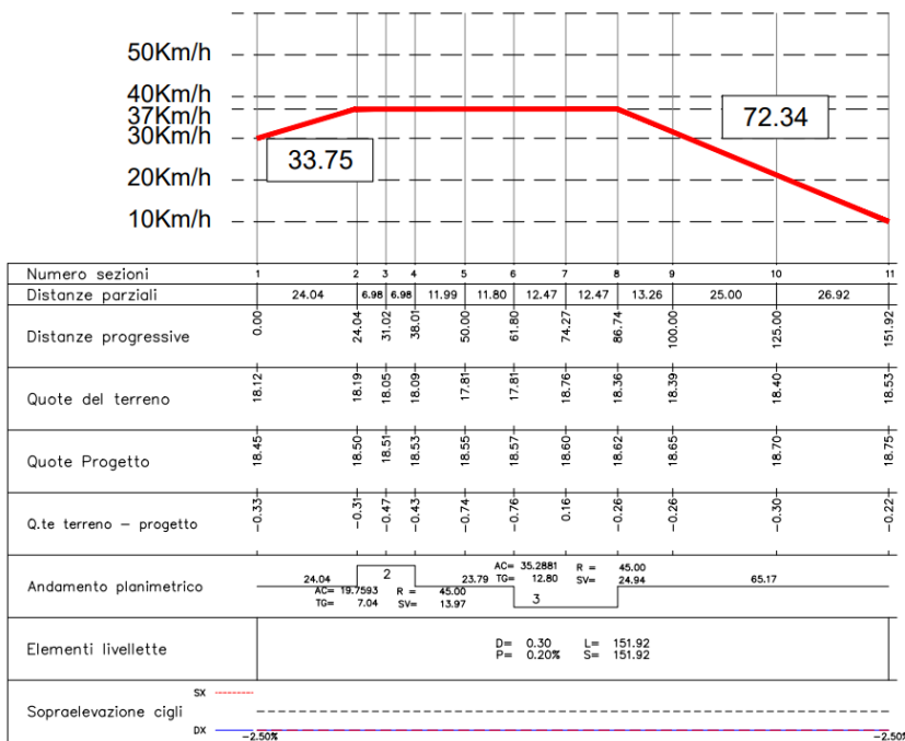
Diagramma velocità planimetrica – Ricucitura n.22
