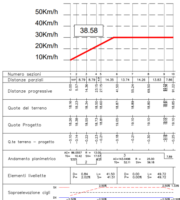
Diagramma velocità planimetrica – Ricucitura n.26
