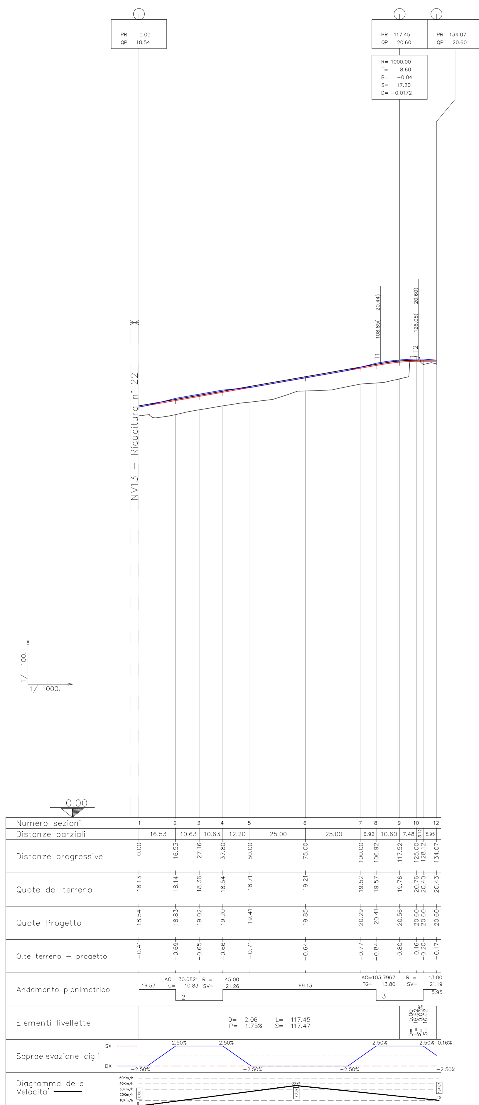
PROFILO LONGITUDINALE RICUCITURA N. 21
