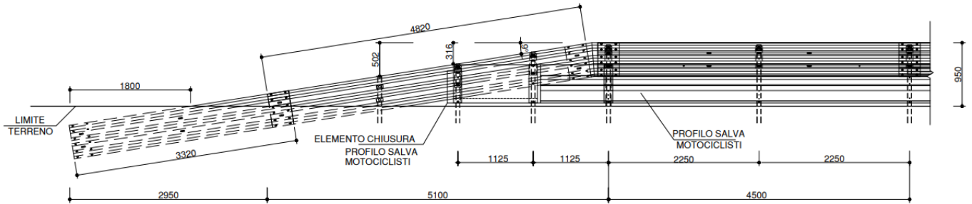
Figura 11.6 – Terminale interrato. Vista laterale
