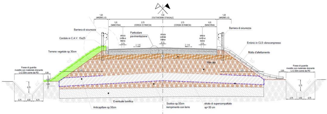
Figura 6.1 – Sezione trasversale tipologica
