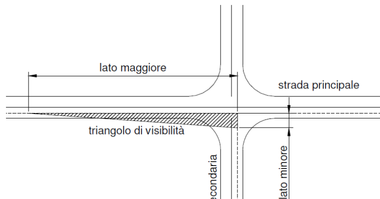
Figura 14.1 – Schematizzazione dei triangoli di visibilità
