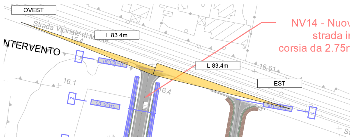
Figura 14.2 – Triangolo di visibilità all'intersezione fra la NV14 e la Strada vicinale Monte
