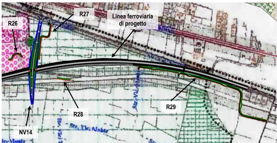
Figura 4.2 – Inquadramento funzionale su PRG
