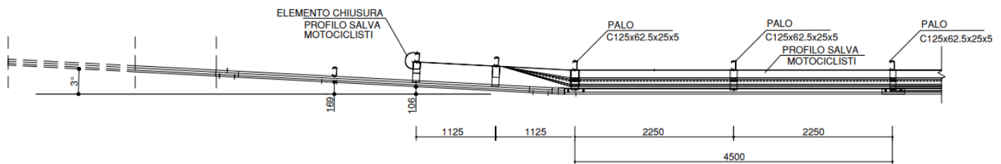
Figura 11.7 – Terminale interrato. Vista dall'alto
