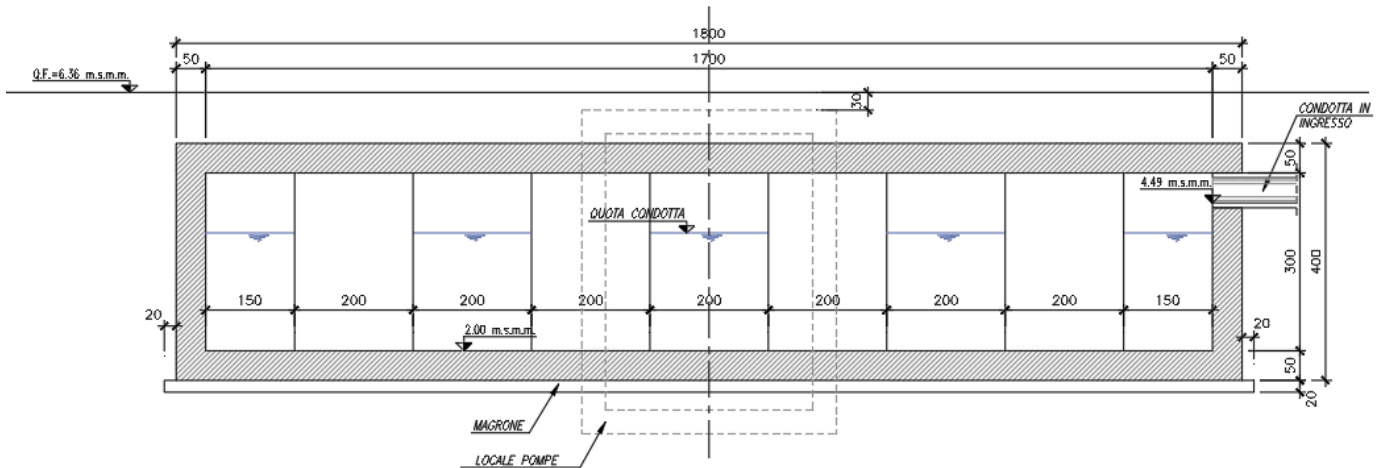
Figura 2 – Sezione trasversale e caratteristiche vasca
