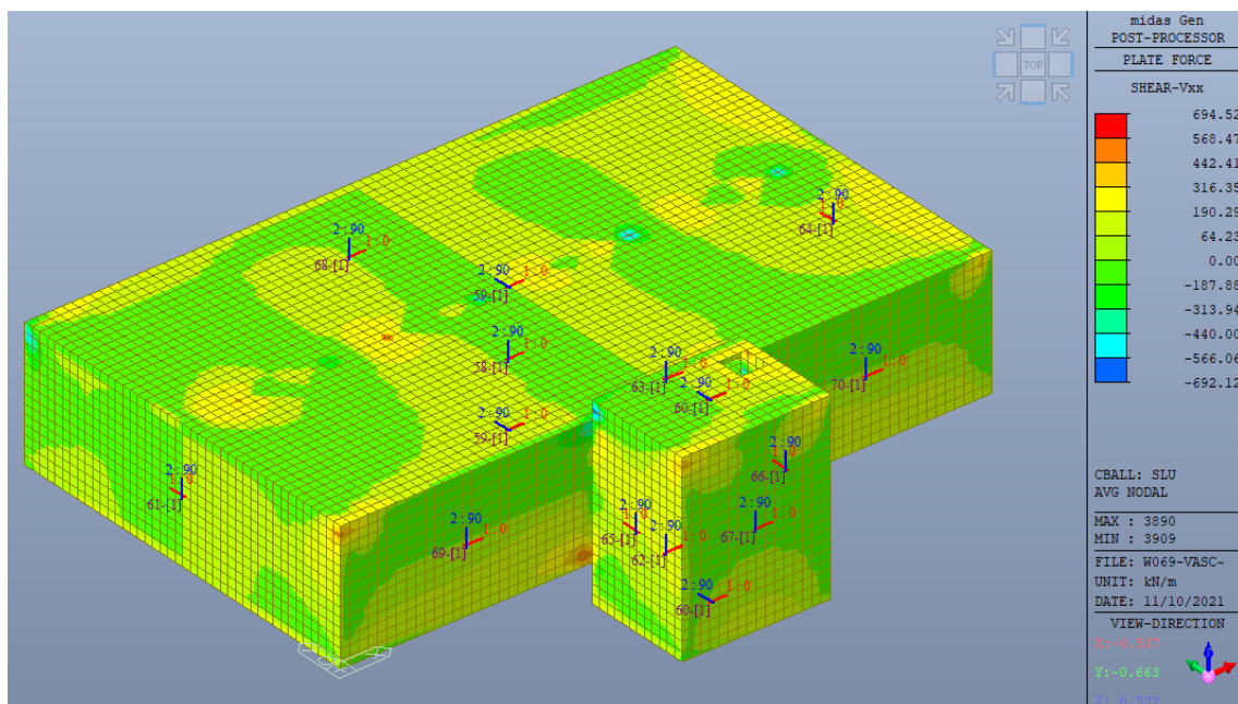
Figura 7 – Diagramma involuppo del taglio (SLV)
