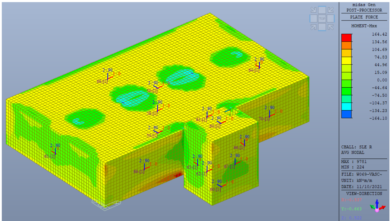
Figura 9 – Diagramma involuppo del momento flettente (SLE)
