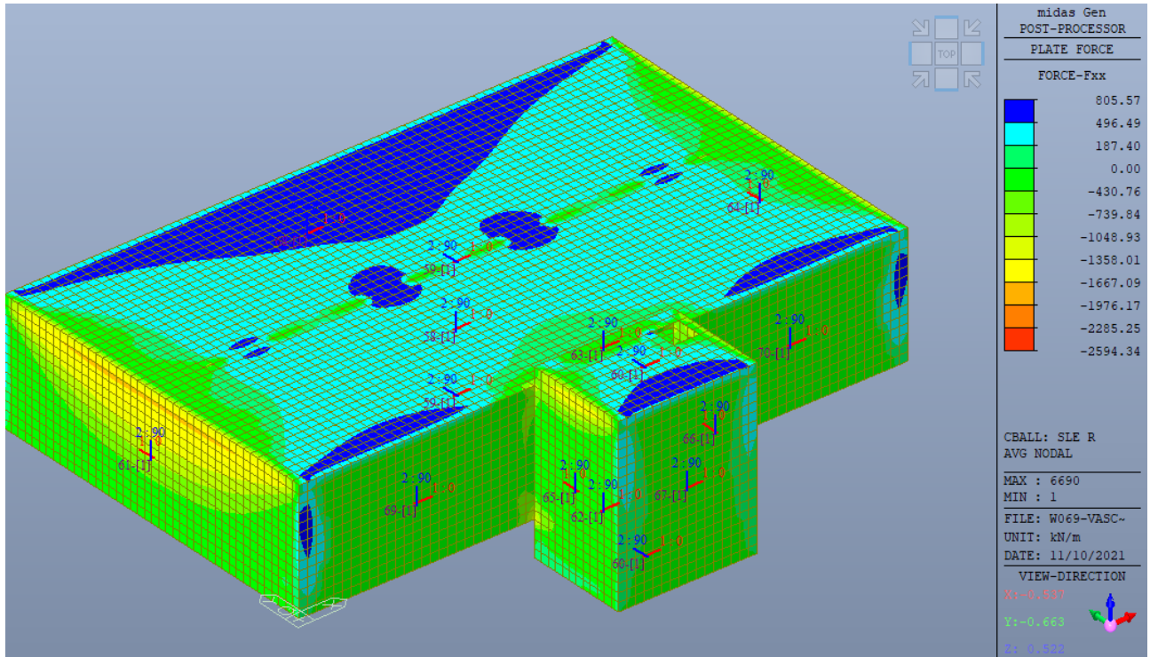
Figura 11 – Diagramma involuppo dello sforzo normale (SLE)
