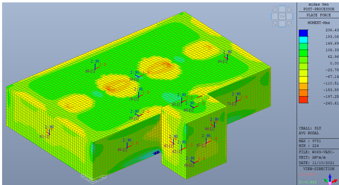
Figura 6 – Diagramma involuppo del momento flettente (SLV)
