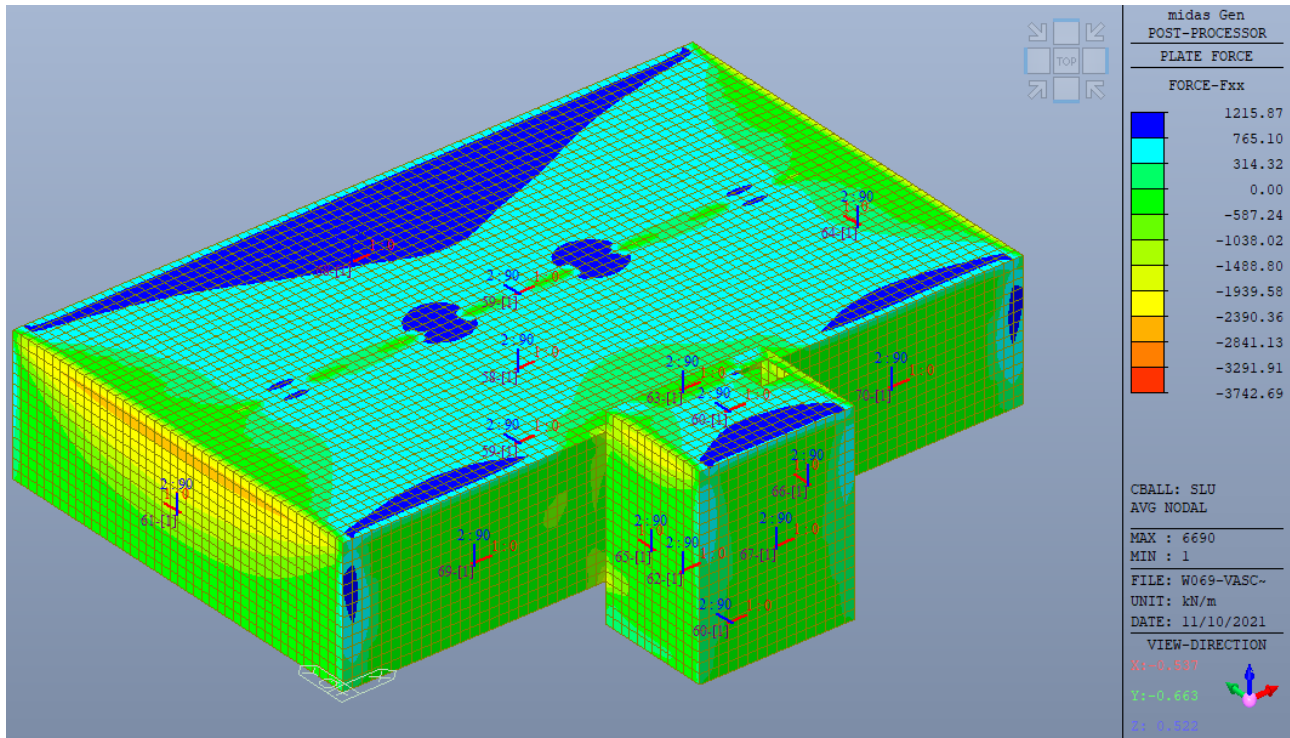
Figura 8 – Diagramma involuppo dello sforzo normale (SLV)
