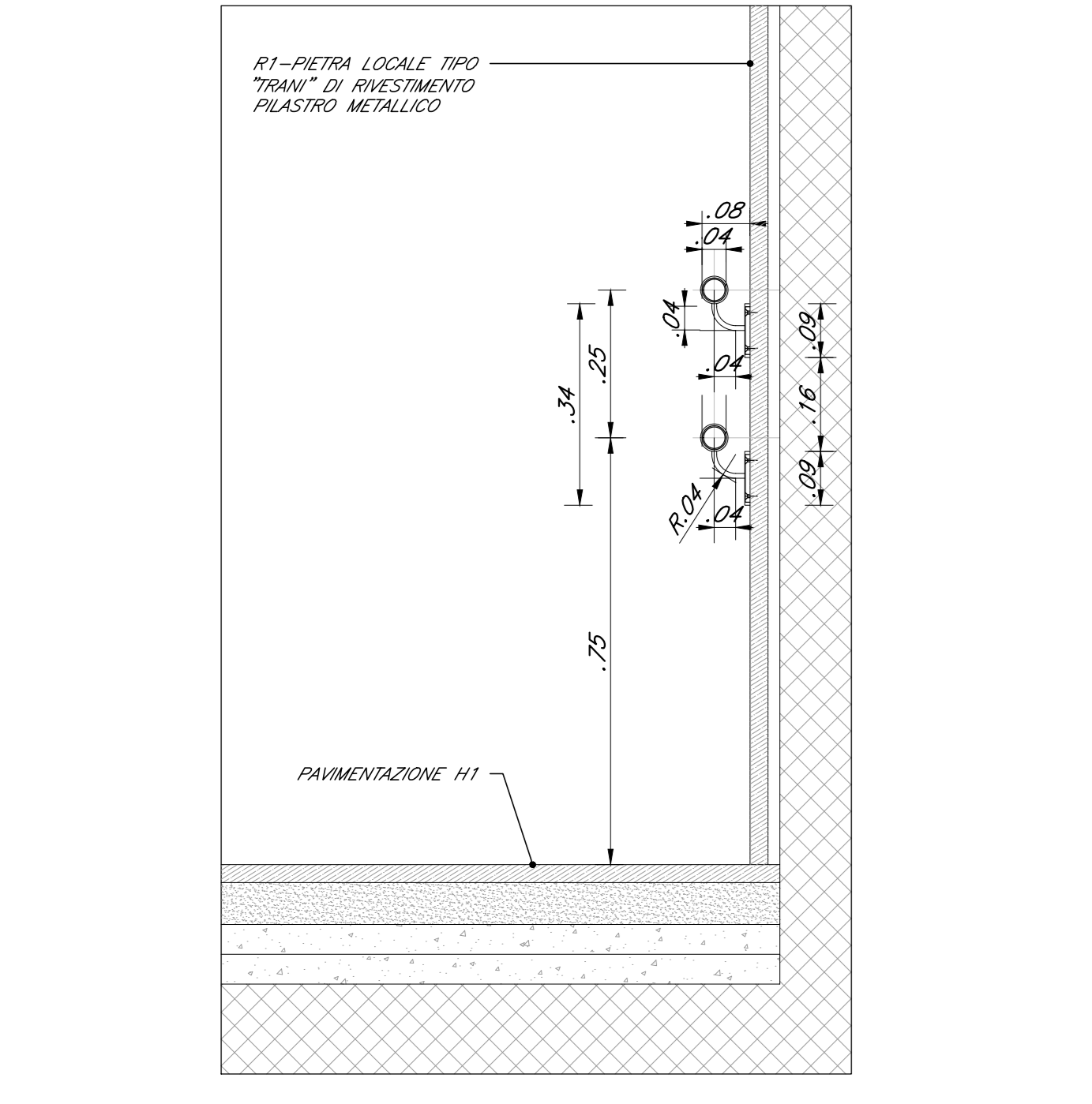
DETTAGLIO L7 CORRIDORO RAMPE E SCALE IN DOPPI TUBOLARI Ø40mm IN ACCIAIO INOX SCALA 1:10
