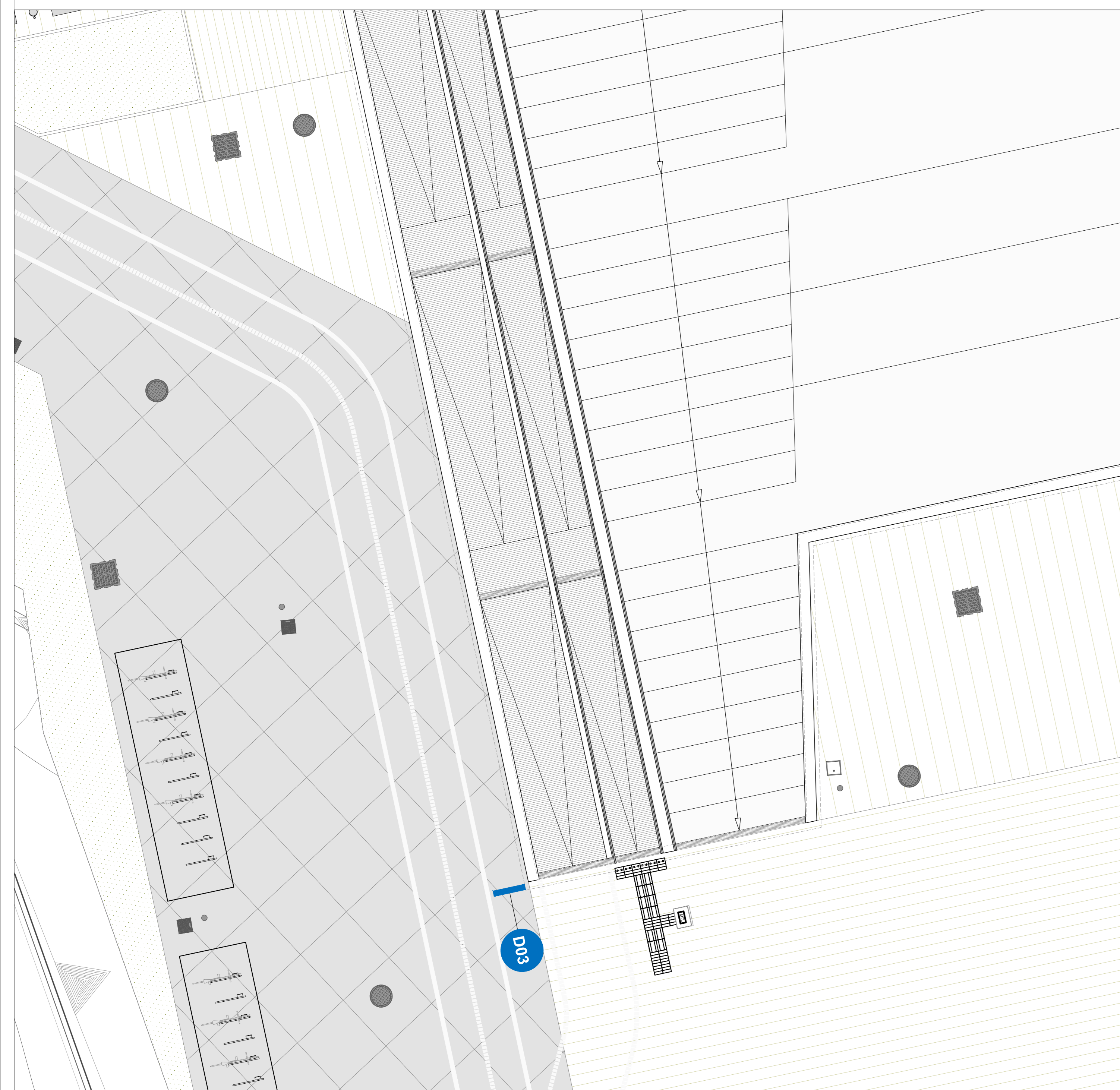
RAMPA CICLOPEDONALE SUD - OVEST SCALA 1:100
