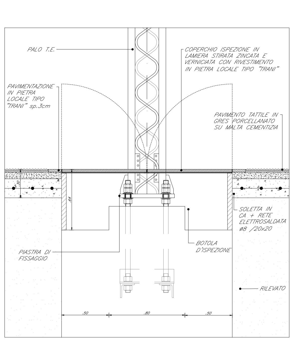
DETTAGLIO 6 PARTICOLARE PALO T.E. CON CHIUSINO D'ISPEZIONE SCALA 1/20
