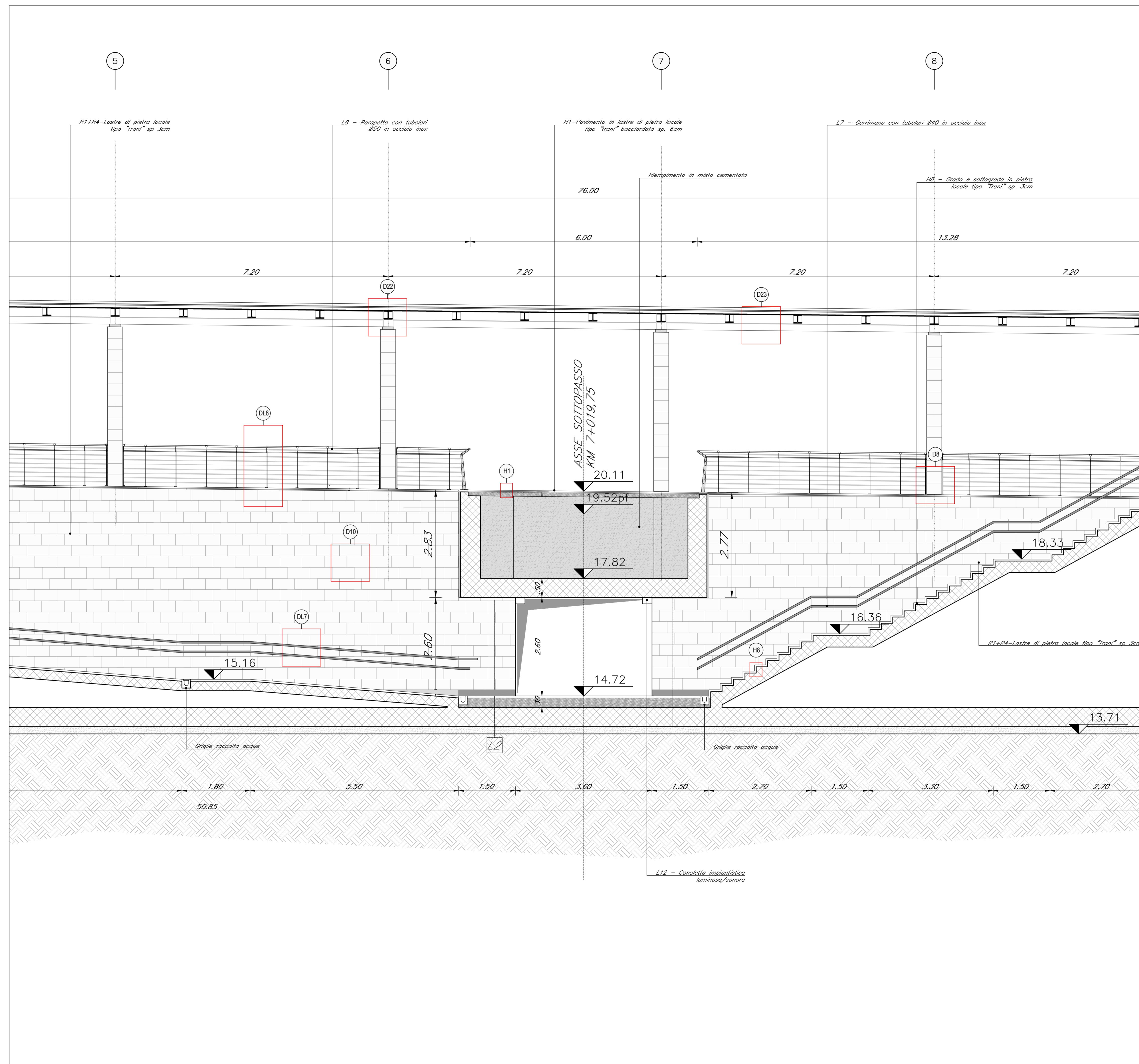
STRALCIO SEZIONE 4-4 SCALA 1:50
