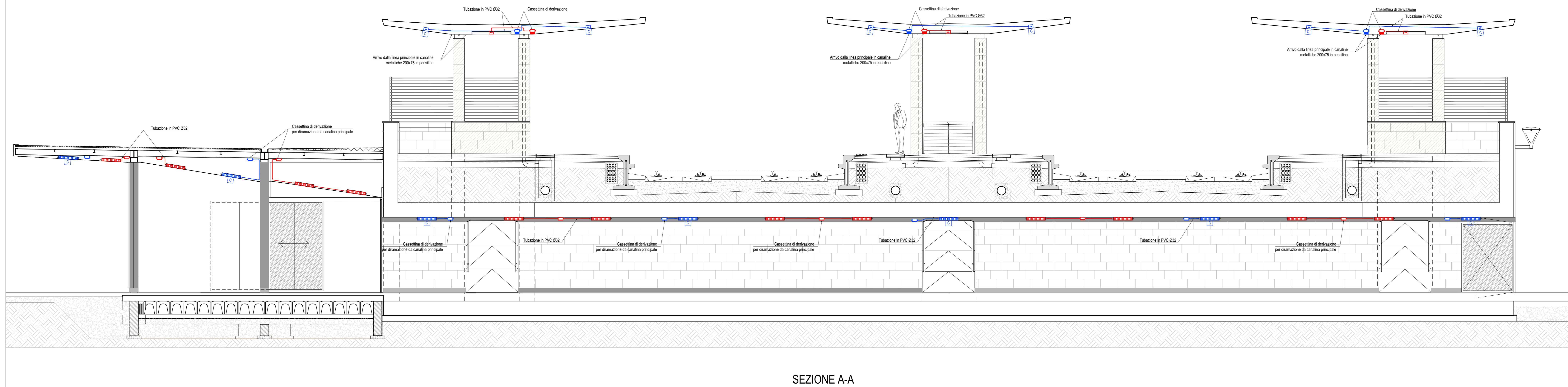
SEZIONE A-A
