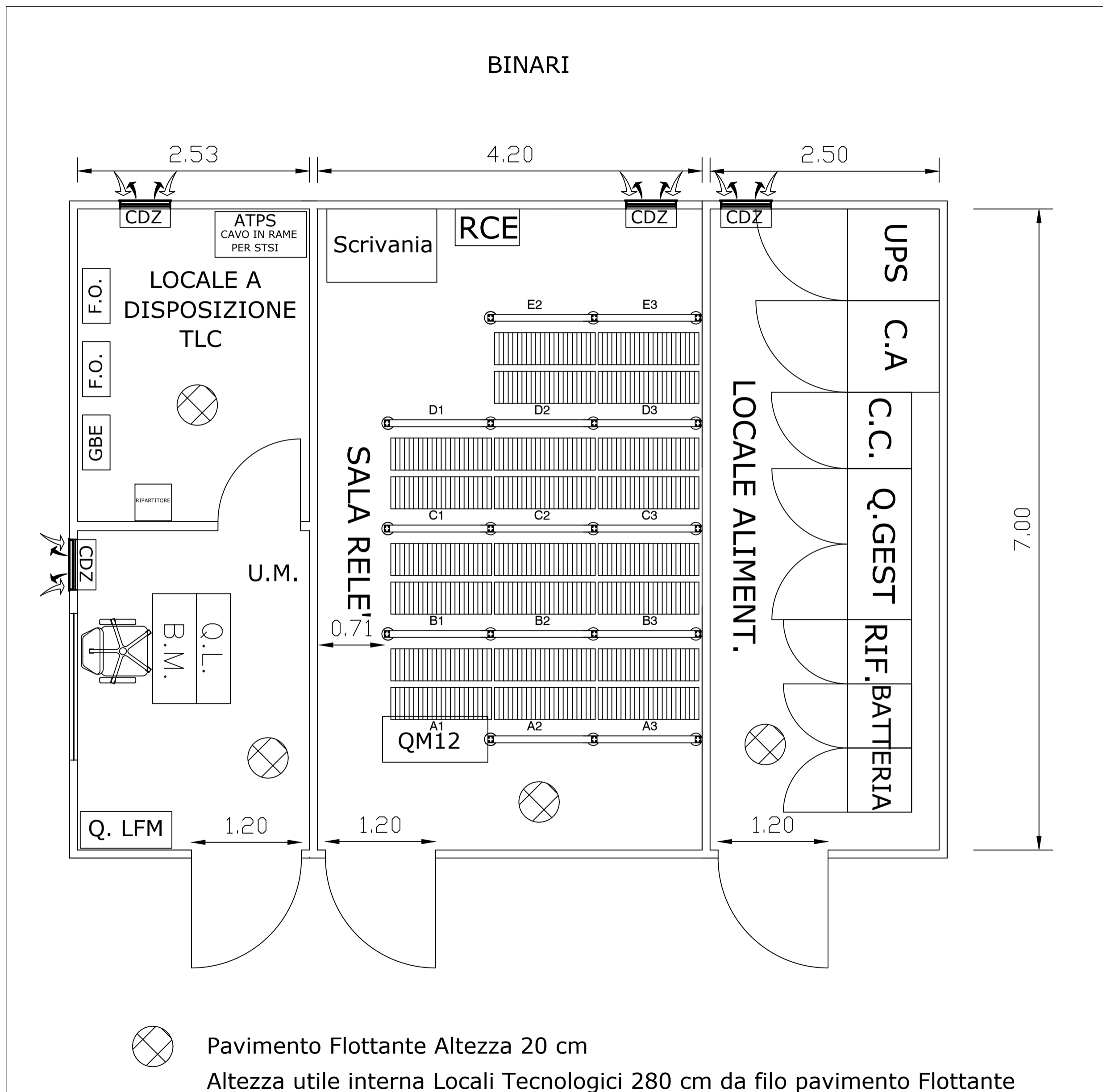
PIANTA DEI LOCALI - SCALA 1:50
