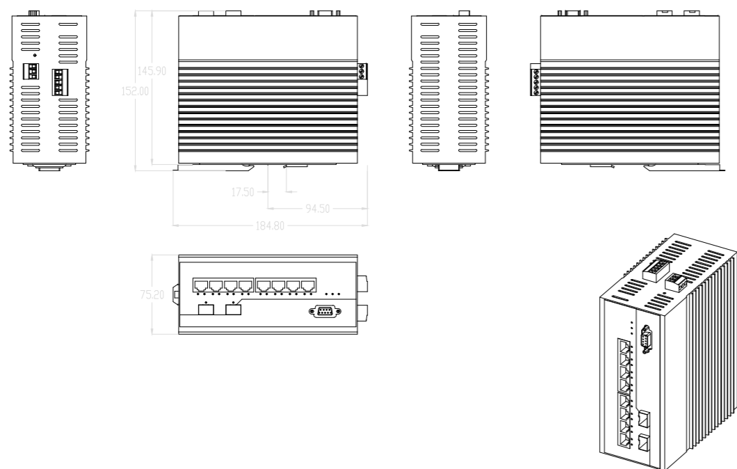
SWITCH 8 porte PoE + 2 SPF
