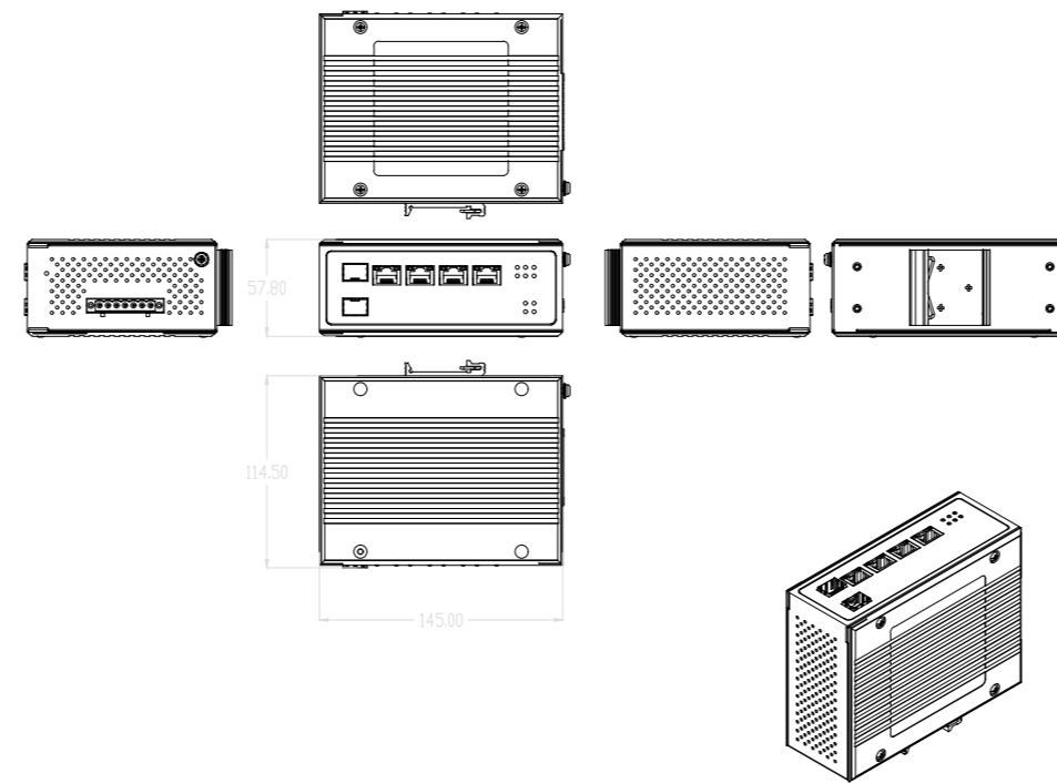
SWITCH 4 porte PoE + 2 SPF
