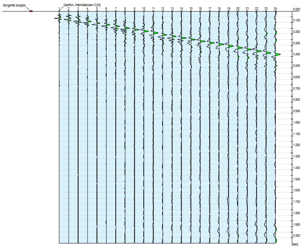
Analisi spettrale
