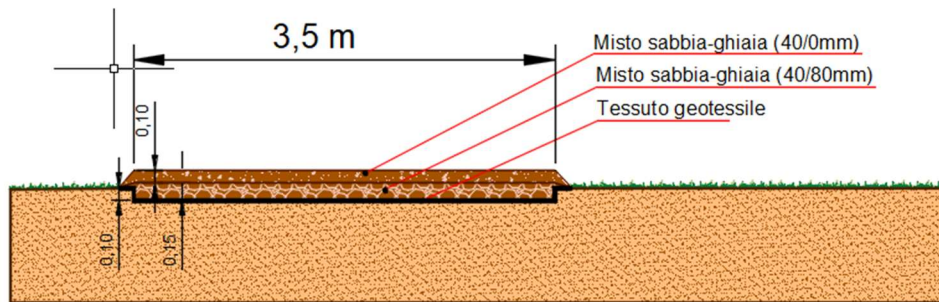
Figura 5. Esempio di stratigrafia stradelli
