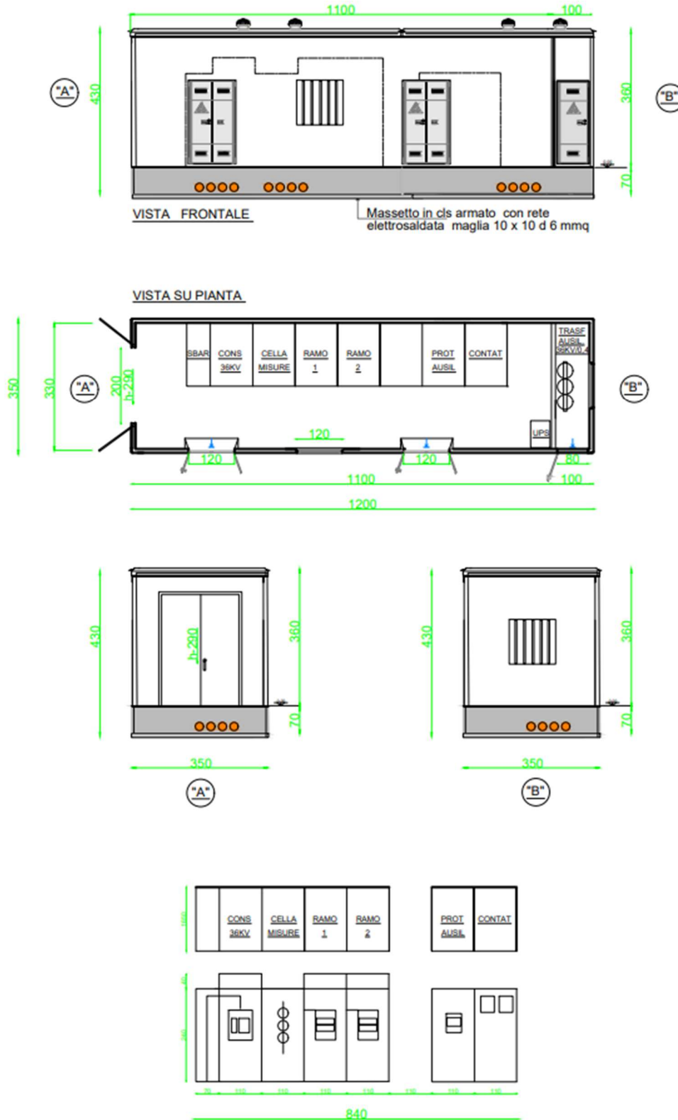
Figura 16. Viste planimetriche e in prospettiva della cabina di smistamento
