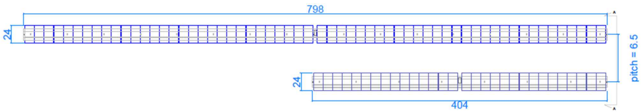
Figura 6. Vista in pianta dei tracker fotovoltaici previsti a progetto (il tracker da 60 moduli è rappresentato parzialmente, per questioni di impaginazione)
