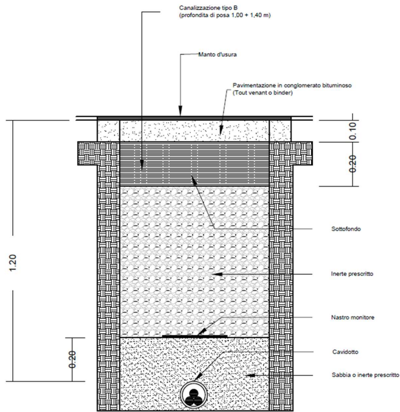
Figura 3. Sezioni tipiche di scavo per cavidotto AT in singola terna su strada asfaltata pubblica
