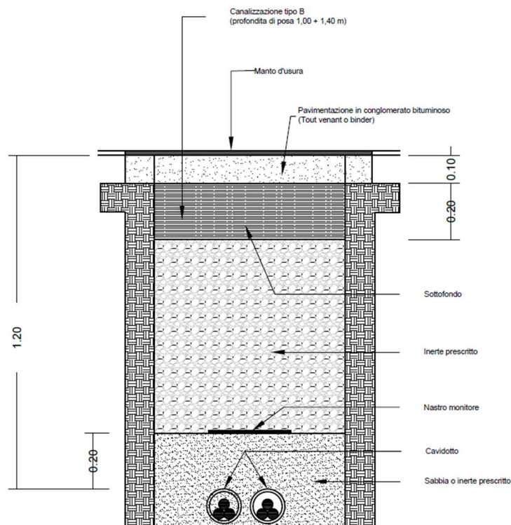
Figura 4. Sezioni tipiche di scavo per cavidotto AT in doppia terna su strada asfaltata pubblica
