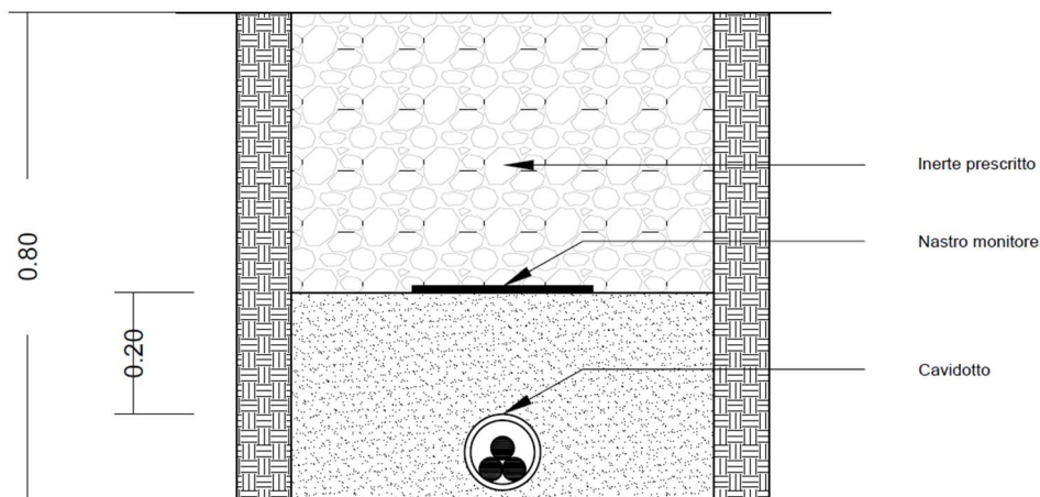
Figura 2. Sezioni tipiche di scavo per cavidotto AT in singola terna su strada sterrata o terreno agricolo
