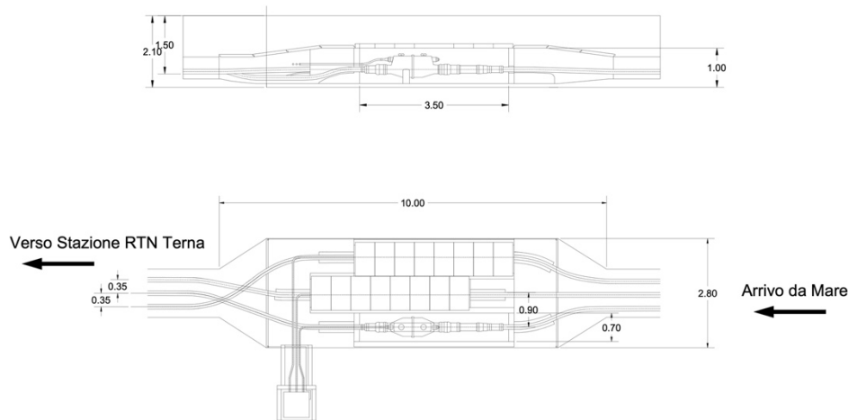
Particolare vasca
