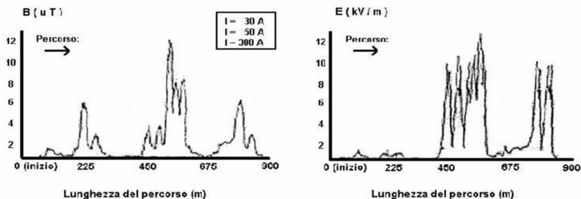
Fig. 2- Risultati della misura dei campi elettrici e magnetici effettuate lungo le vie interne della sezione a 380 kV della stazione riportata in fig. 1
