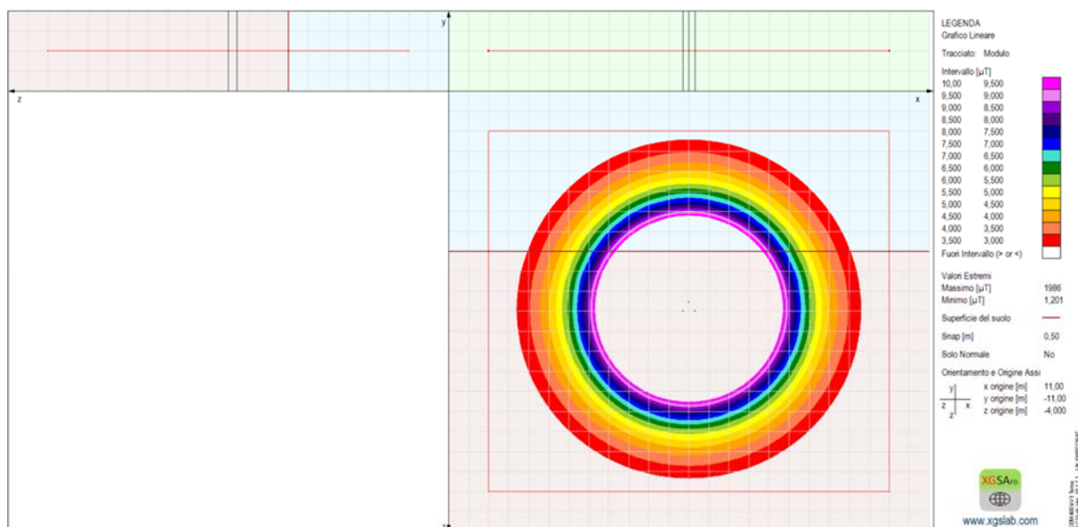
Calcolo Induzione Magnetica sulla sezione del cavo AAT da 1200 mm 2
