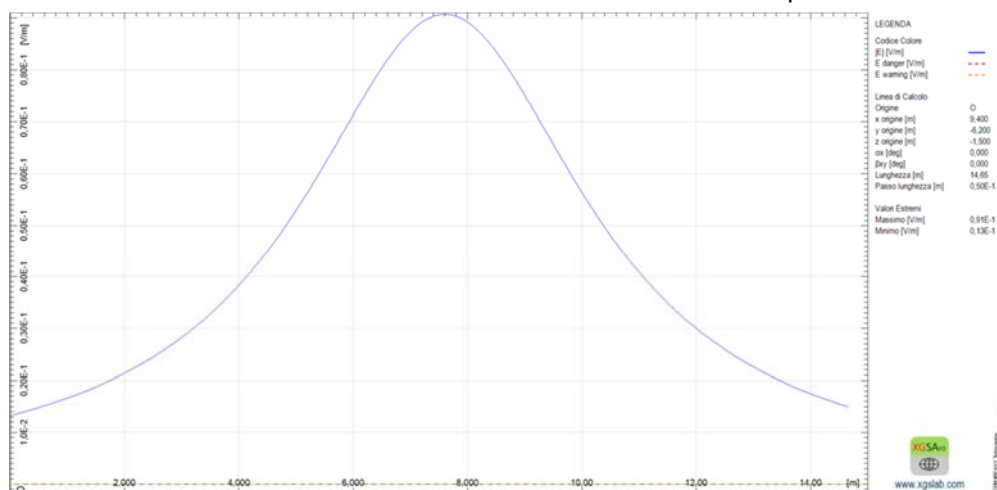
Profilo Campo Elettrico ad altezza a 1,5 m
