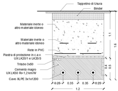
Sezione Scavo tipo cavidotto AAT
