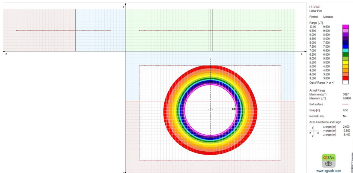
Calcolo Induzione Magnetica sulla sezione del cavo AAT da 2500 mm 2
