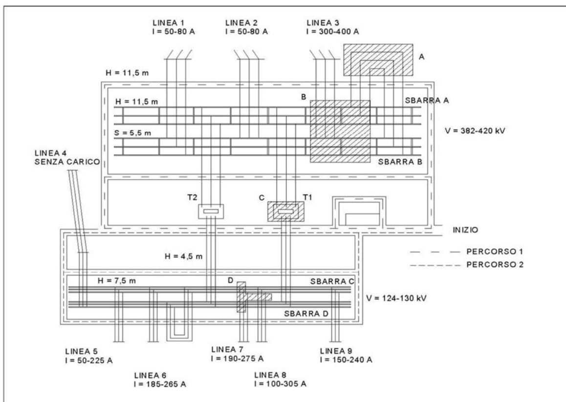
Fig 1 - Pianta di una tipica stazione 380/132 kV con l'indicazione delle principali distanze fase-fase (S) e fase-terra (H) e delle variazioni delle tensioni e delle correnti durante le fasi di misurazioni di campo elettrico e magnetico.
