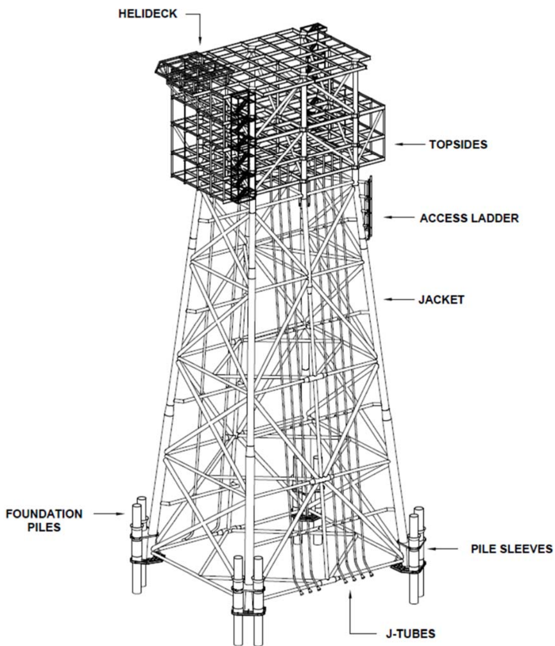
Struttura Piattaforma
