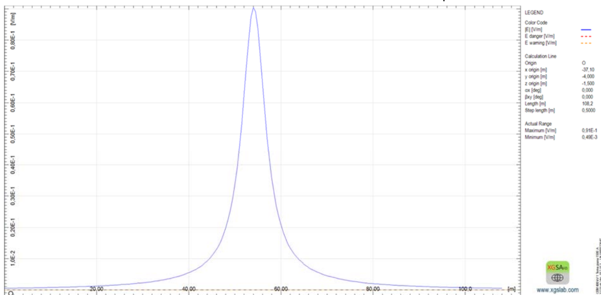
Profilo Campo Elettrico ad altezza a 1,5 m
