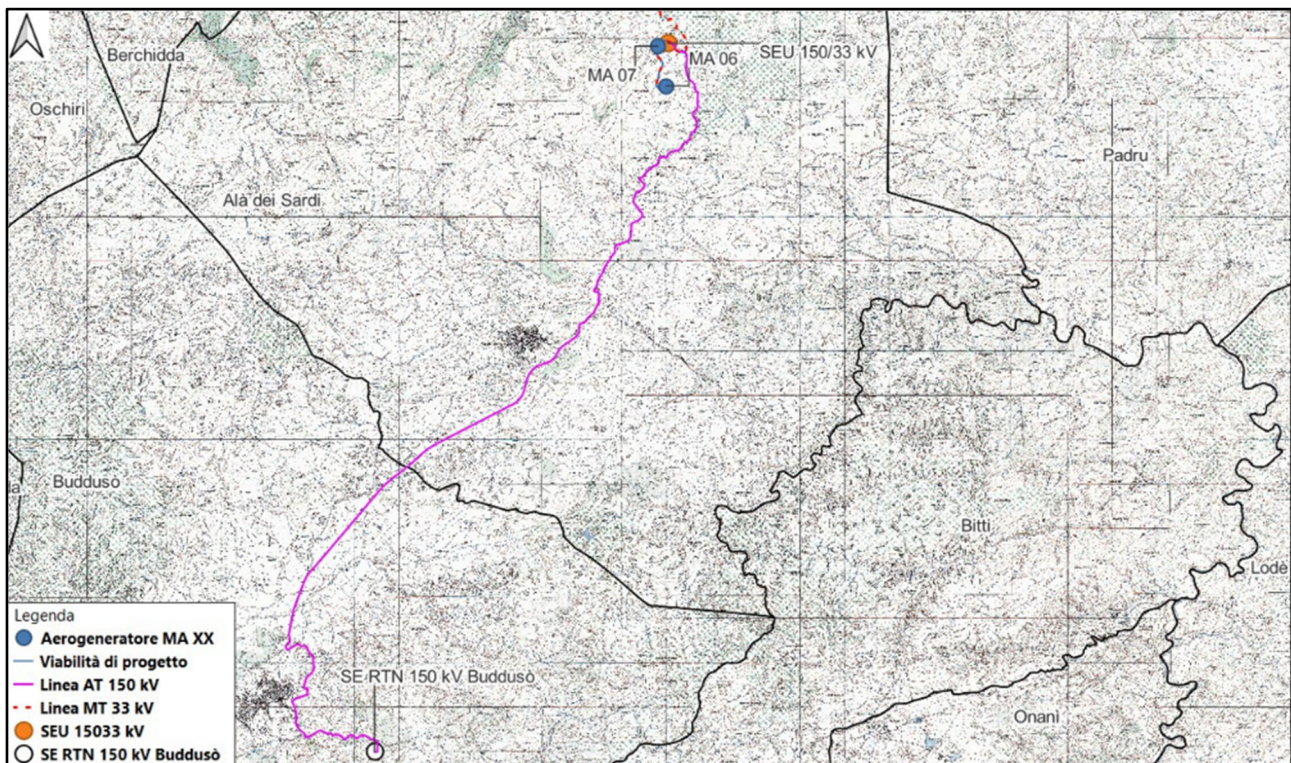
Figura 3.2: Soluzione di connessione a 150 kV in corrispondenza della stazione elettrica RTN Terna 150 kV Buddusò (di futura realizzazione)
