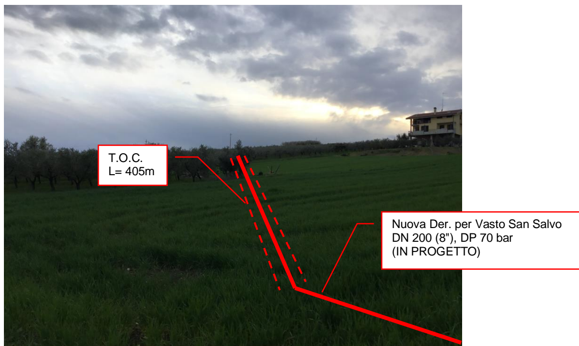
Foto n.17 – Km 6+000 - Metanodotto in progetto con vista T.O.C.
