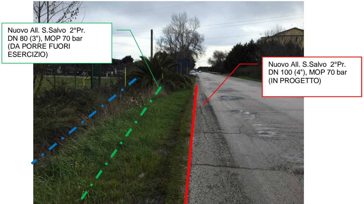
Foto n.31 – Km 8+700 - Panoramica metanodotti su S.P. 197 via Trignina (CH)
