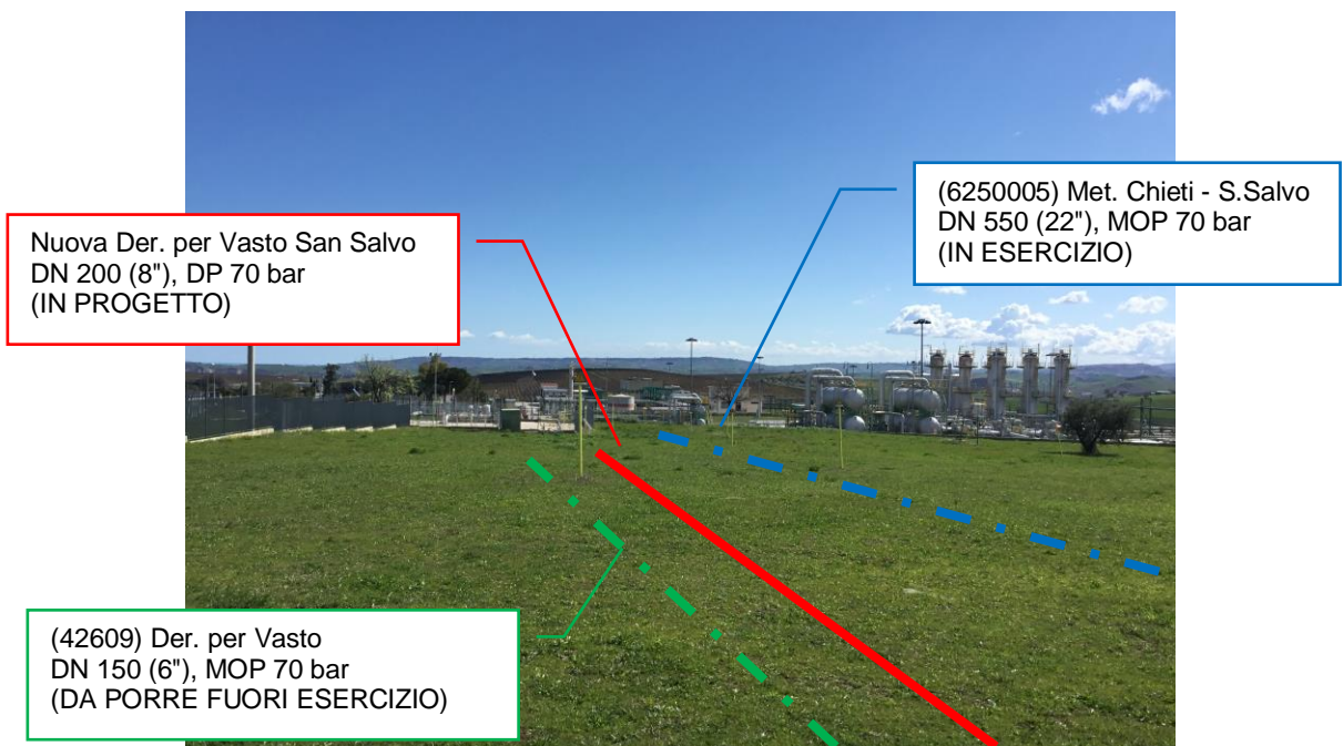
Foto n.2 – Km 0+060 - Panoramica metanodotti esistenti, da porre fuori esercizio e in progetto
