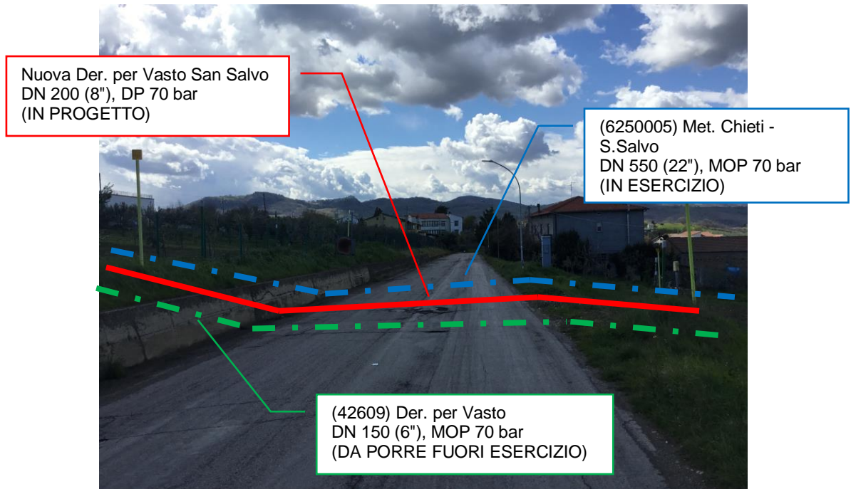
Foto n.4 – Km 0+163 - Attraversamento metanodotti su S.P. 187 (S.P. Trignina)
