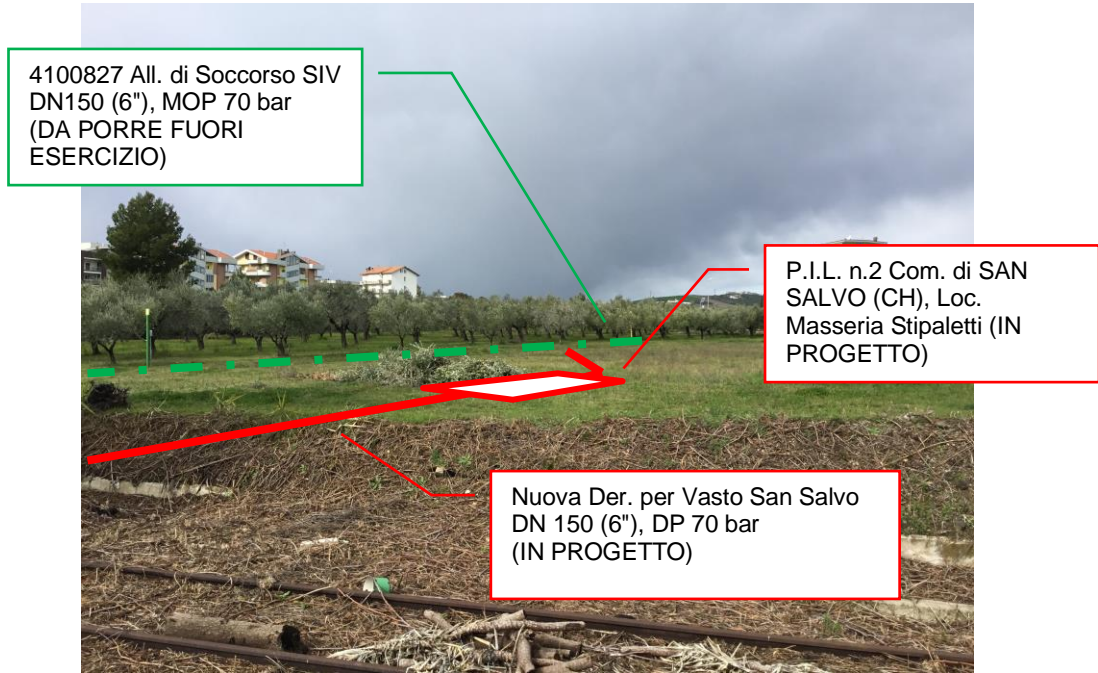
Foto n.21 – Km 7+195 - Met. in progetto con vista impianto PIL n.2 in progetto e met. da porre fuori esercizio
