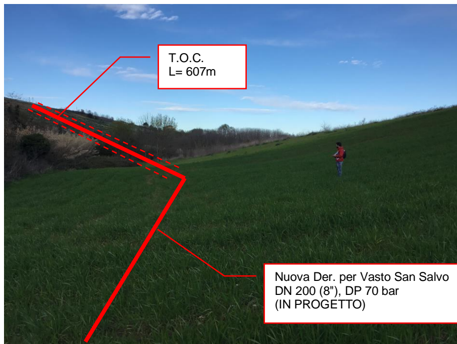
Foto n.16 – Km 4+845 - Metanodotto in progetto con vista T.O.C.
