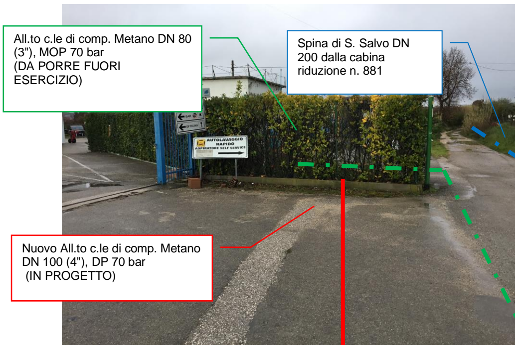
Foto n.30 – Km 8+700 - Vista metanodotti presso area di distribuzione metano
