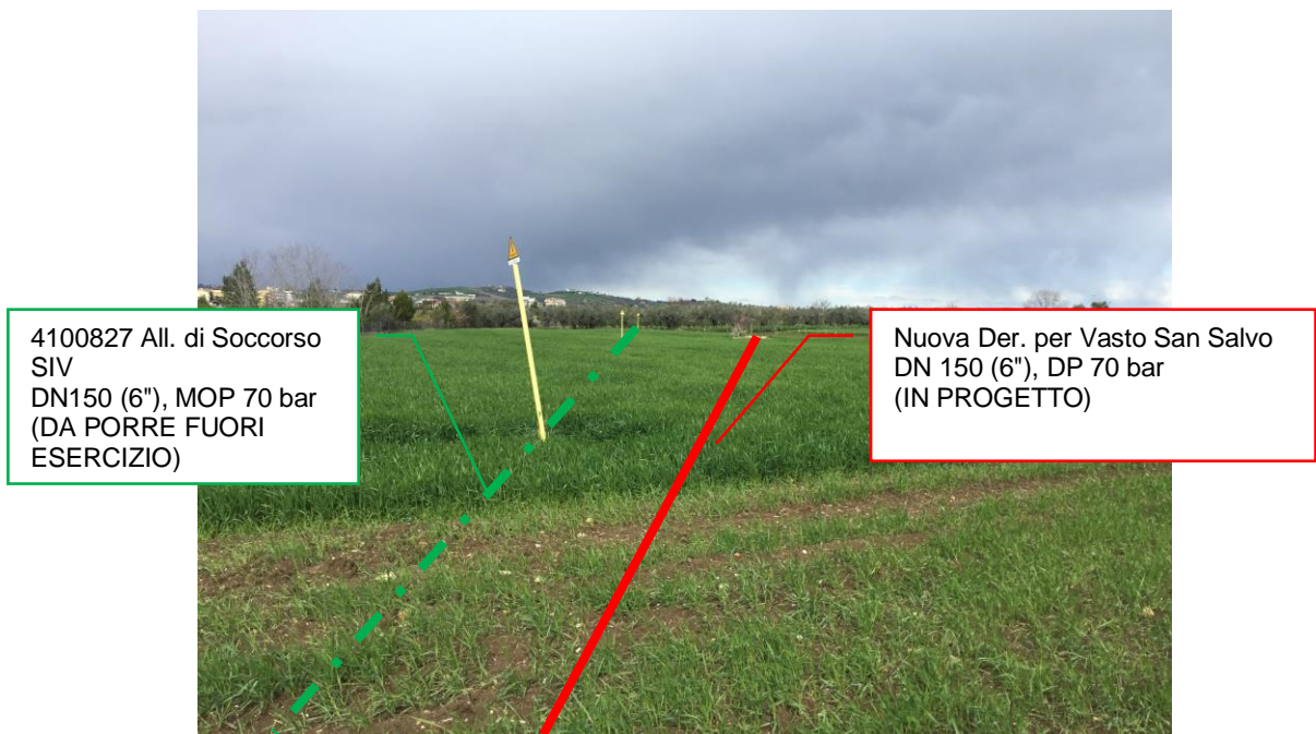
Foto n.22 – Km 7+870 - Panoramica metanodotti da porre fuori esercizio e in progetto
