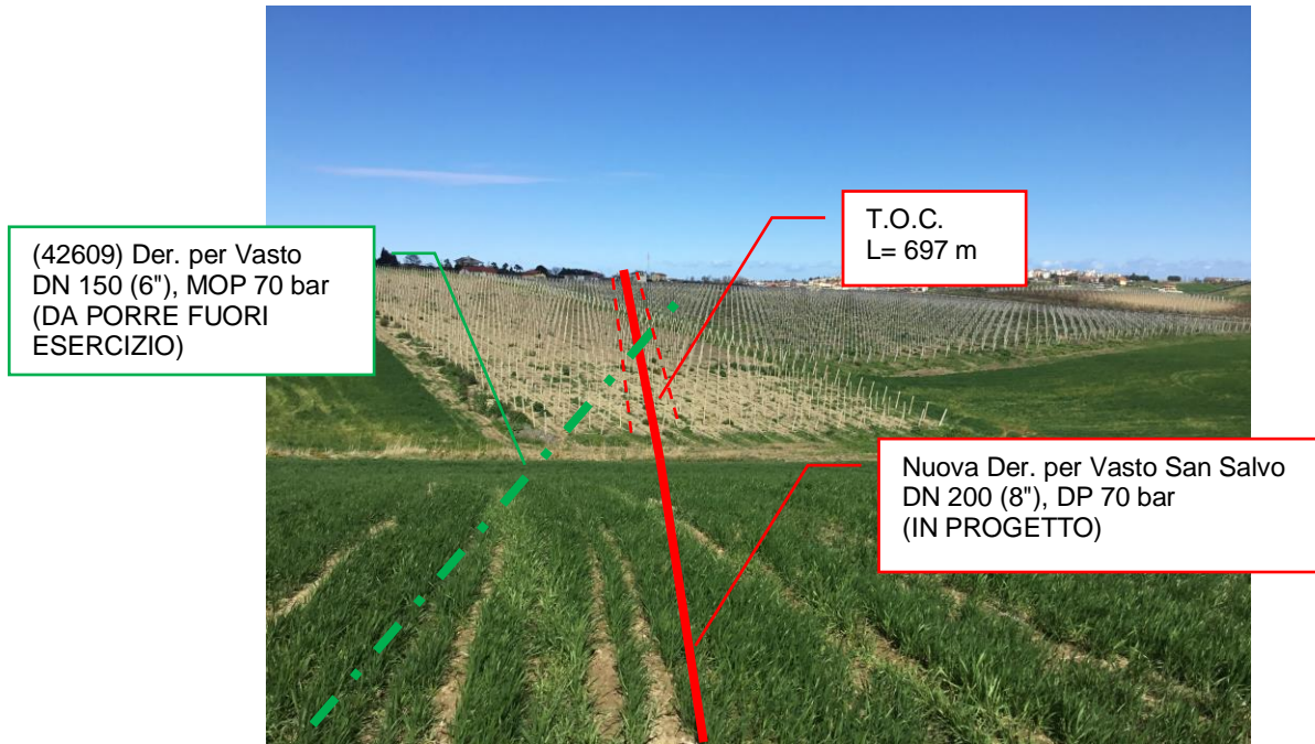
Foto n.9 – Km 1+506 - Metanodotto in progetto con vista T.O.C. e metanodotto da porre fuori esercizio
