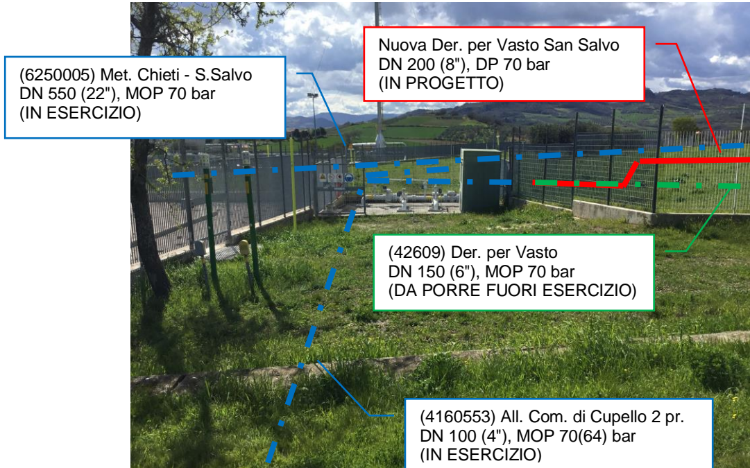
Foto n.1 – Km 0+000 - Metanodotti esistenti, da porre fuori esercizio e in progetto con vista area impianto
