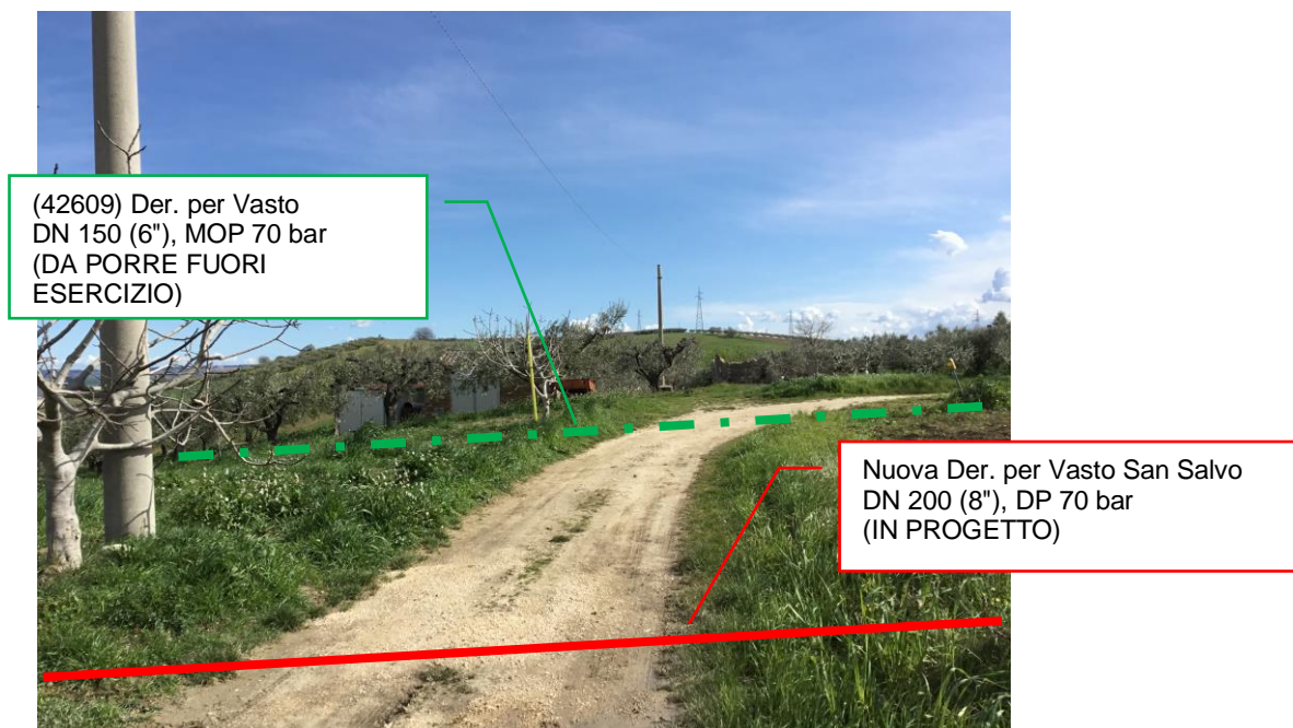
Foto n.10 – Km 2+355 - Vista attraversamento di metanodotti su strada
