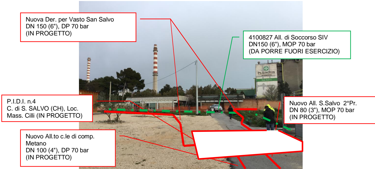
Foto n.27 – Km 8+700 - Vista Area impianti e metanodotti in progetto
