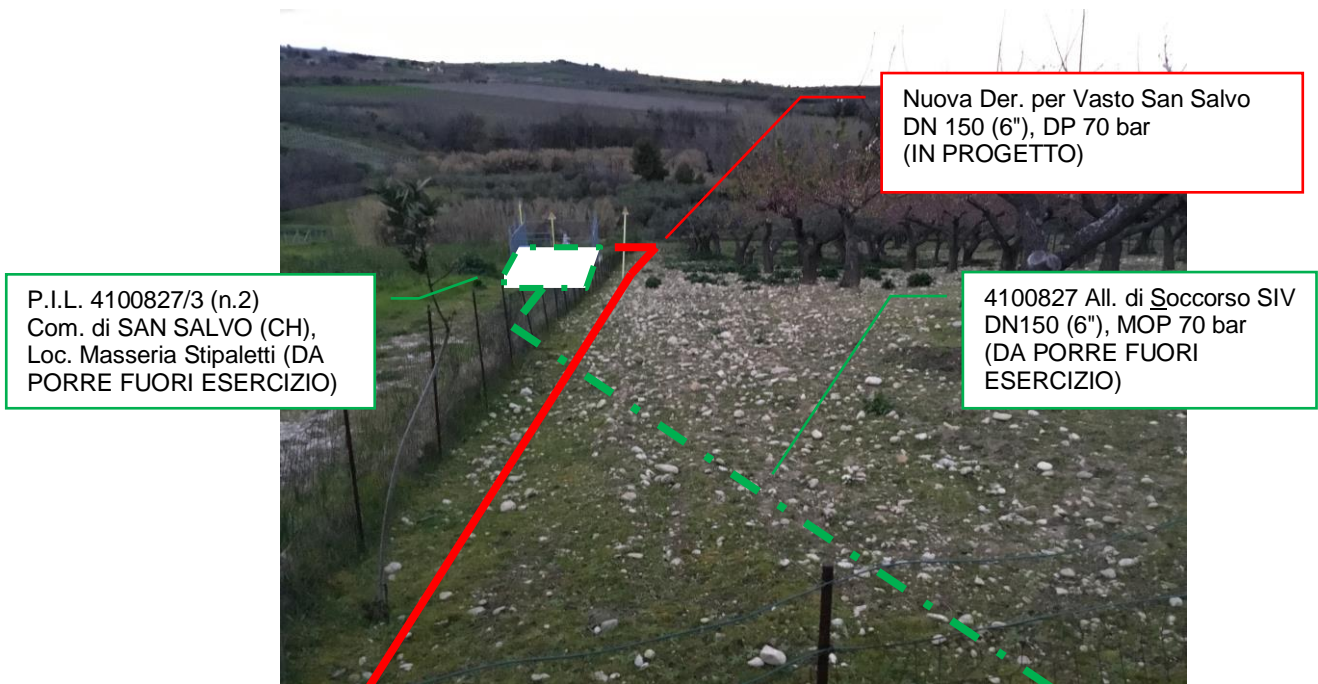
Foto n.20 – Km 6+970 - Vista met. da porre fuori esercizio, in progetto e impianto PIL da porre fuori esercizio
