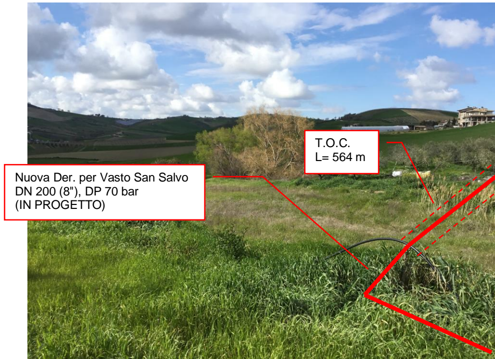
Foto n.5 – Km 0+320 -Nuova Der. per Vasto San Salvo DN 200 (8”), DP 70 bar (IN PROGETTO)
