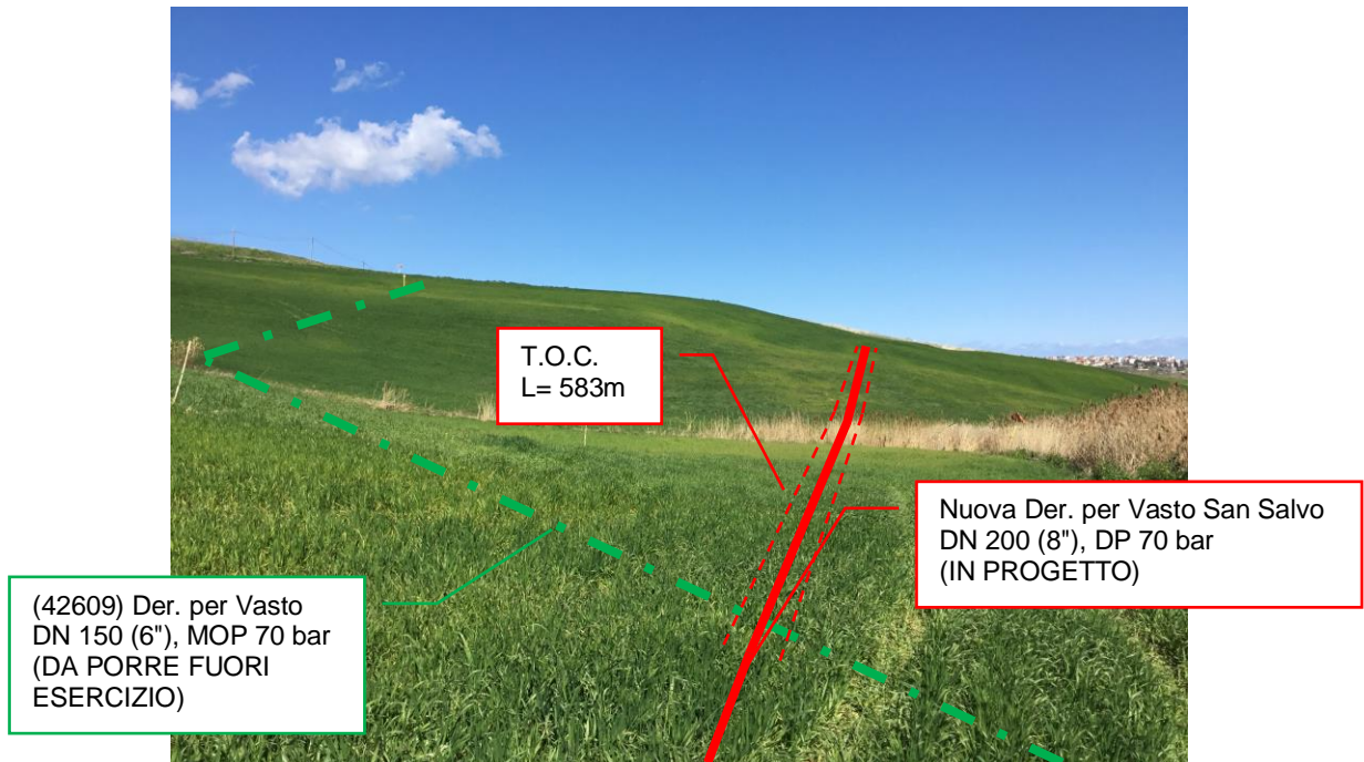
Foto n.8 – Km 0+915 - Metanodotto in progetto con vista T.O.C. e metanodotto da porre fuori esercizio
