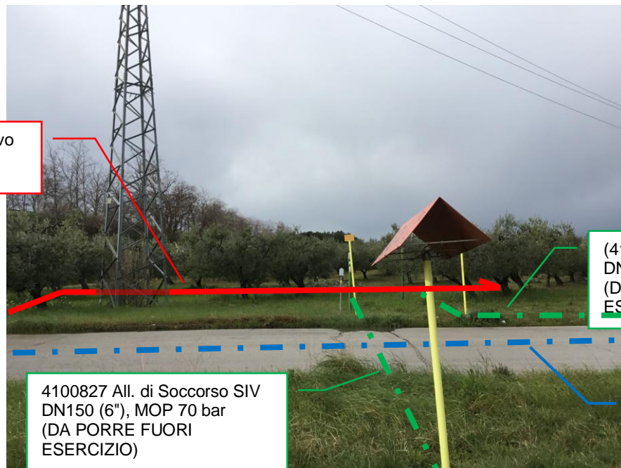
Foto n.24 – Km 8+125 - Percorrenza metanodotti su contrada Piane S. Angelo S.P. 200
