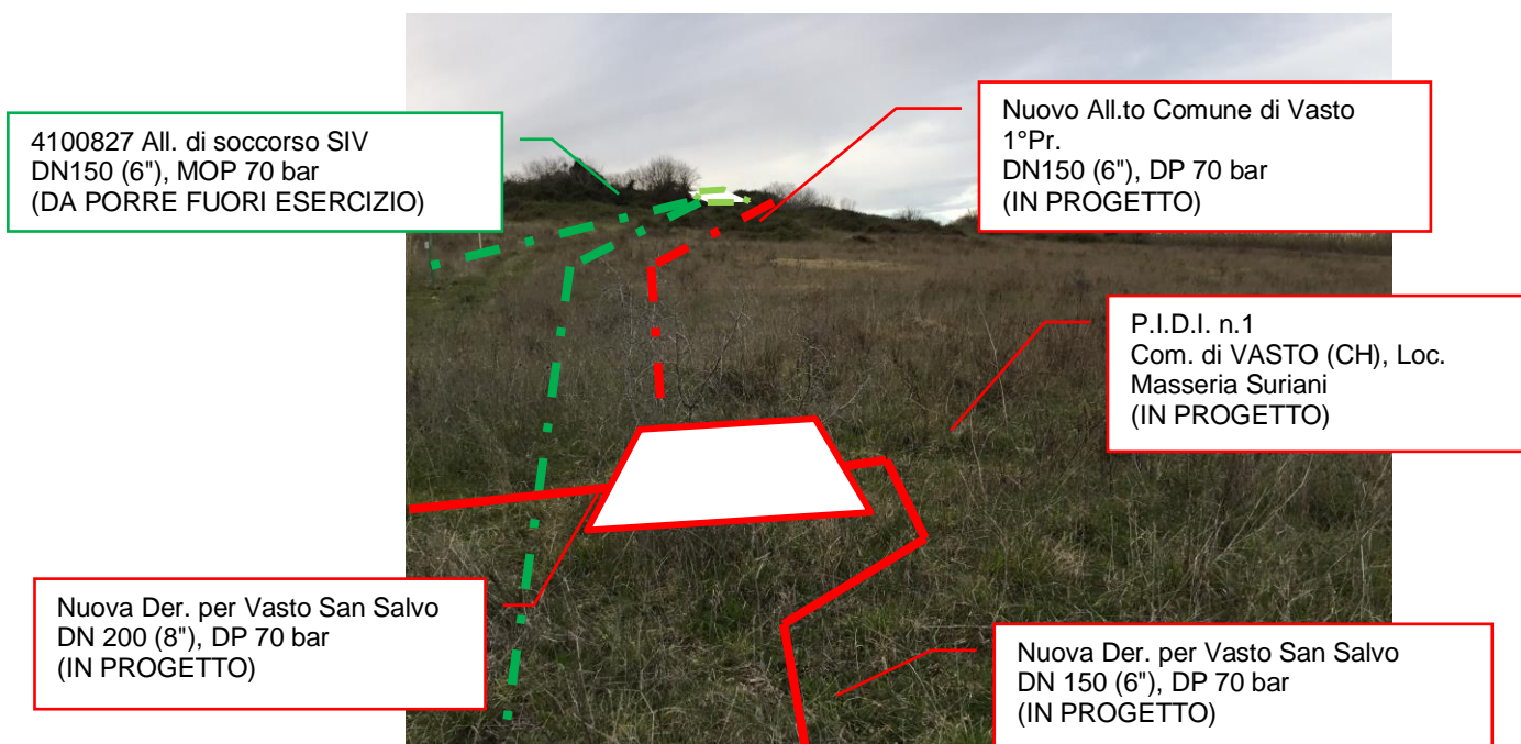
Foto n.18 – Km 6+200 - Met. in progetto con vista impianto PIDI n.1 in progetto e met. da porre fuori esercizio
