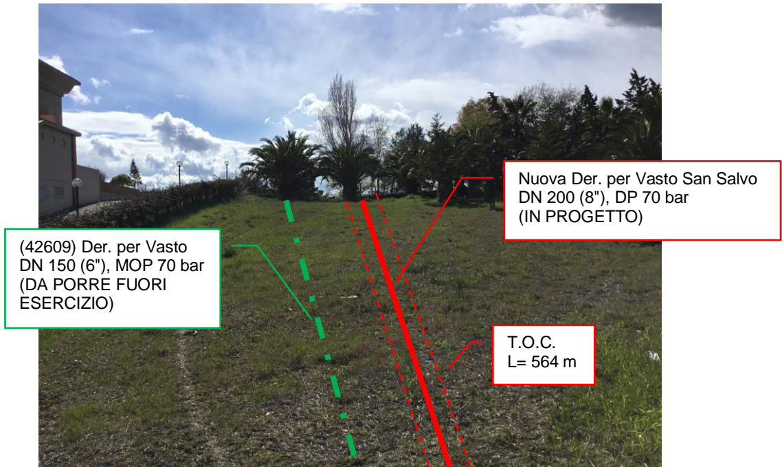
Foto n.7 – Km 0+730 - Metanodotti da porre fuori esercizio e in progetto
