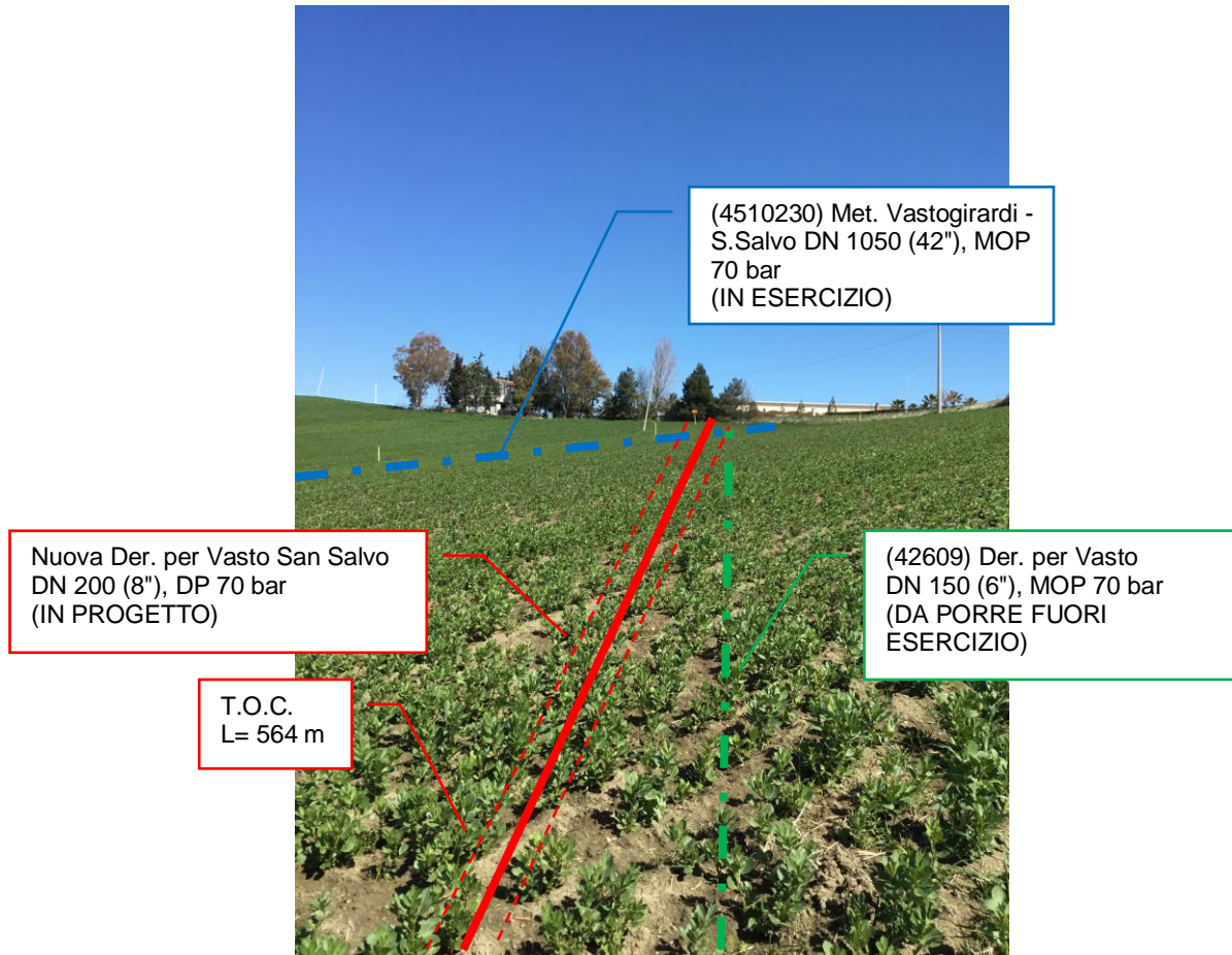
Foto n.6 – Km 0+400 - Panoramica metanodotti esistenti, da porre fuori esercizio e in progetto
