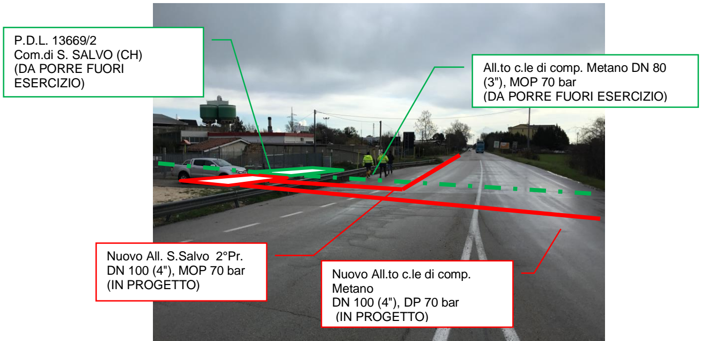
Foto n.28 – Km 8+700 - Vista Area impianti e metanodotti in progetto e da porre fuori esercizio
