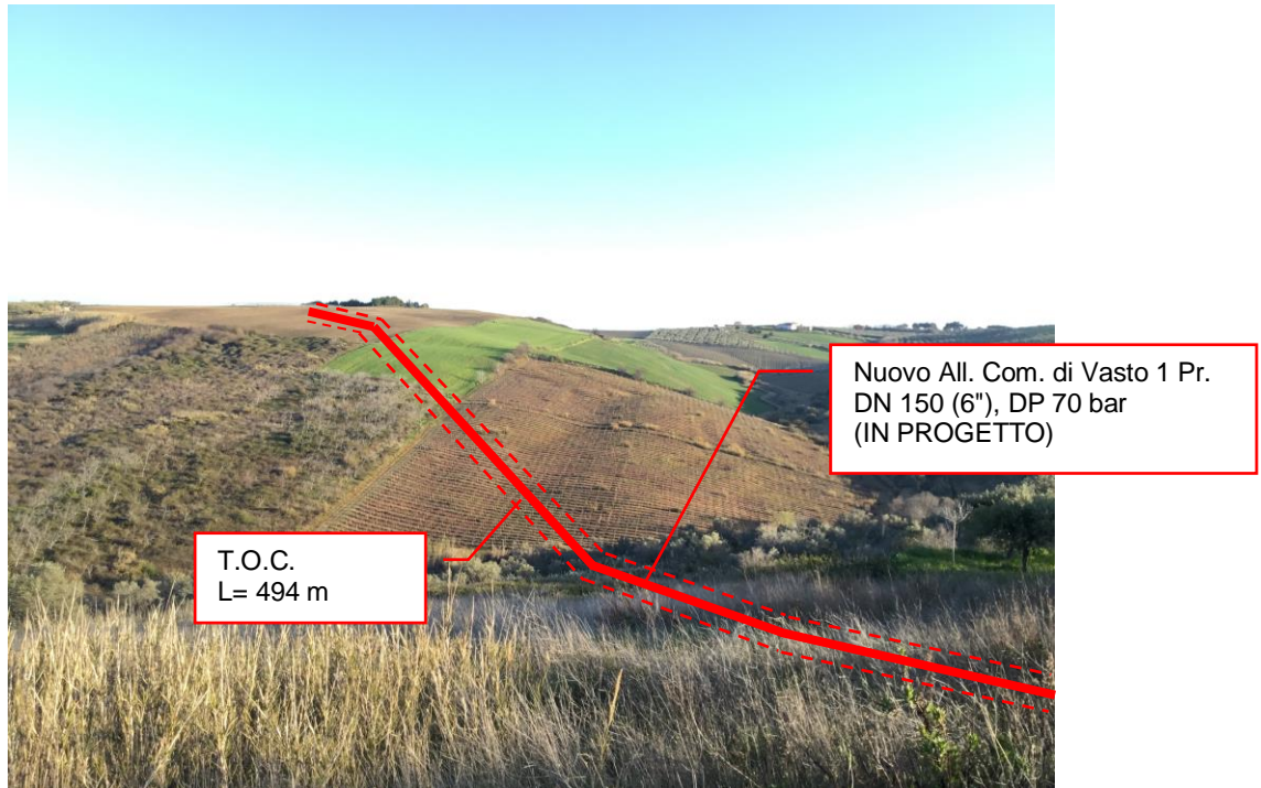
Foto n.7 – Km 3+210 - Nuovo All. Com. di Vasto 1 Pr. Dn 150 (6'') DP 70 bar (IN PROGETTO) con vista TOC
