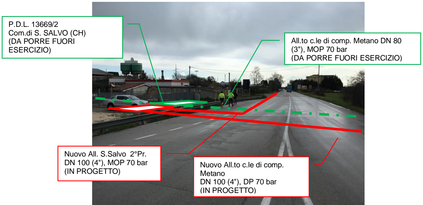
Foto n.21 – Km 2+716 - Vista Area impianti e metanodotti in progetto e da porre fuori esercizio
