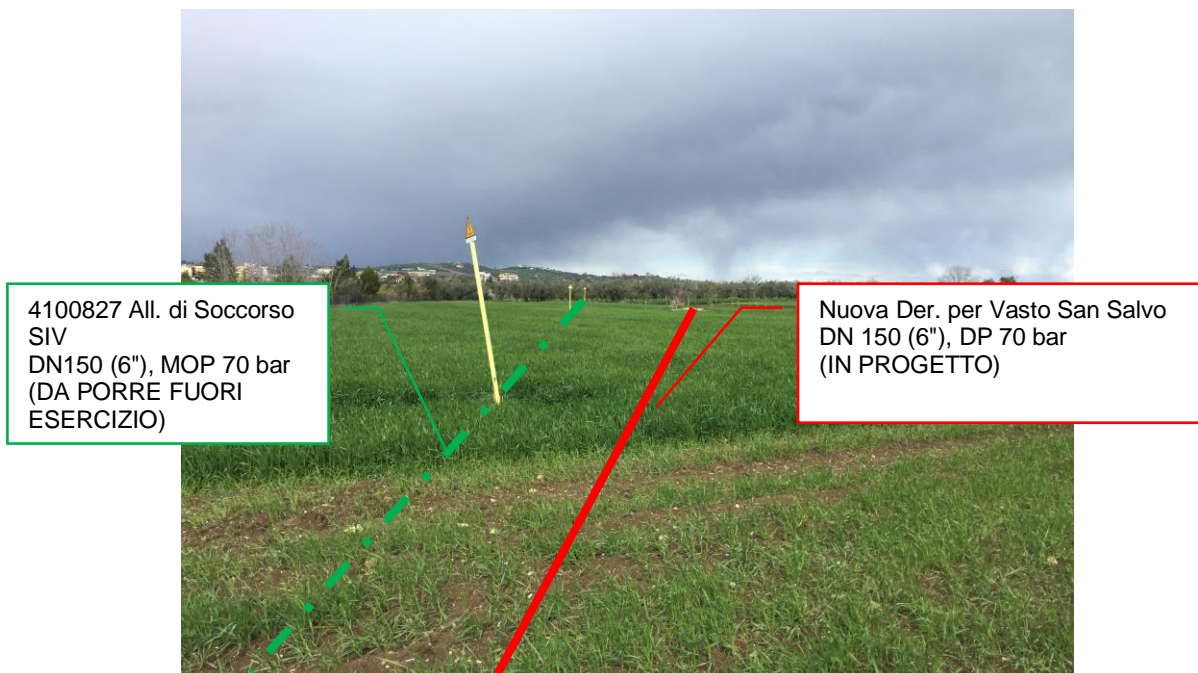
Foto n.15 – Km 1+870 - Panoramica metanodotti da porre fuori esercizio e in progetto
