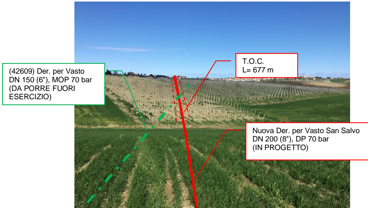
Foto n.8 – Km 1+511 - Metanodotto in progetto con vista T.O.C. e metanodotto da porre fuori esercizio
