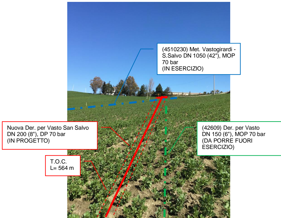
Foto n.5 – Km 0+360 -Panoramica metanodotti esistenti, da porre fuori esercizio e in progetto
