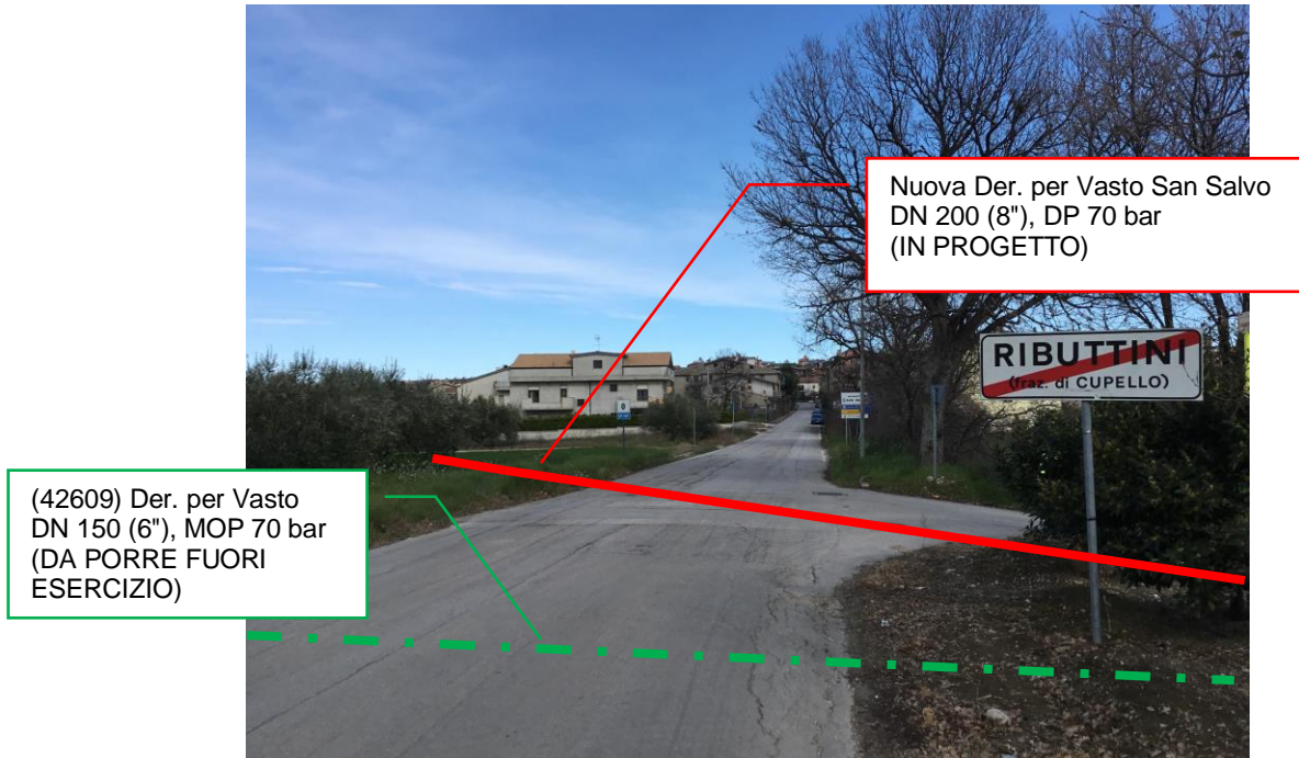
Foto n.10 – Km 2+742 - Attraversamento metanodotti su S.P. 182 (Via dei Palmoli)
