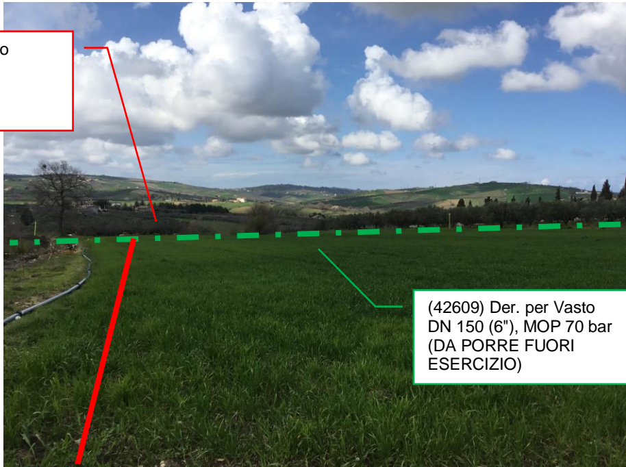
Foto n.26 – Km0+395 - Panoramica metanodotti in progetto e da porre fuori esercizio
