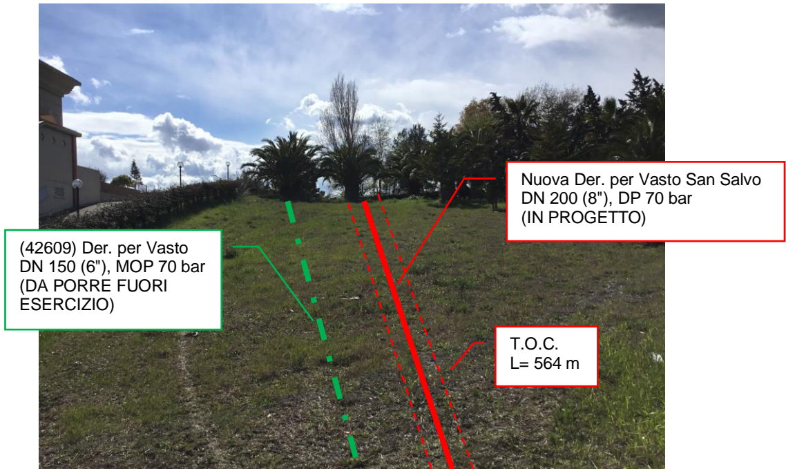
Foto n.6 – Km 0+700 - Metanodotti da porre fuori esercizio e in progetto
