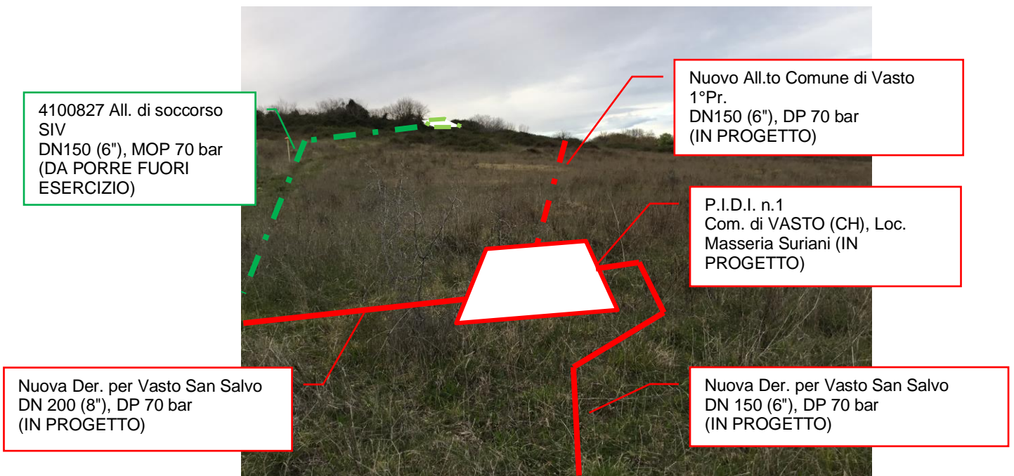
Foto n.11 – 0+222 - Met. in progetto con vista impianto PIDI n.1 in progetto e met. da porre fuori esercizio
