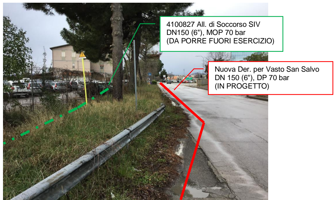
Foto n.19 – Km 2+502 - Percorrenza metanodotti su S.P. 200
