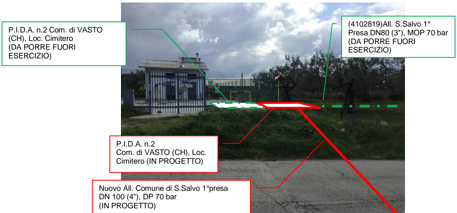
Foto n.25 – Km 0+475 - Area impianti e metanodotti da porre fuori esercizio e in progetto
