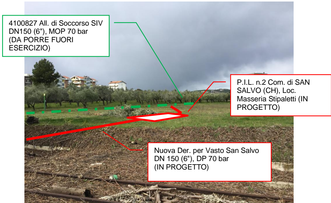
Foto n.14 – Km 1+194 - Met. in progetto con vista impianto PIL n.2 in progetto e met. da porre fuori esercizio
