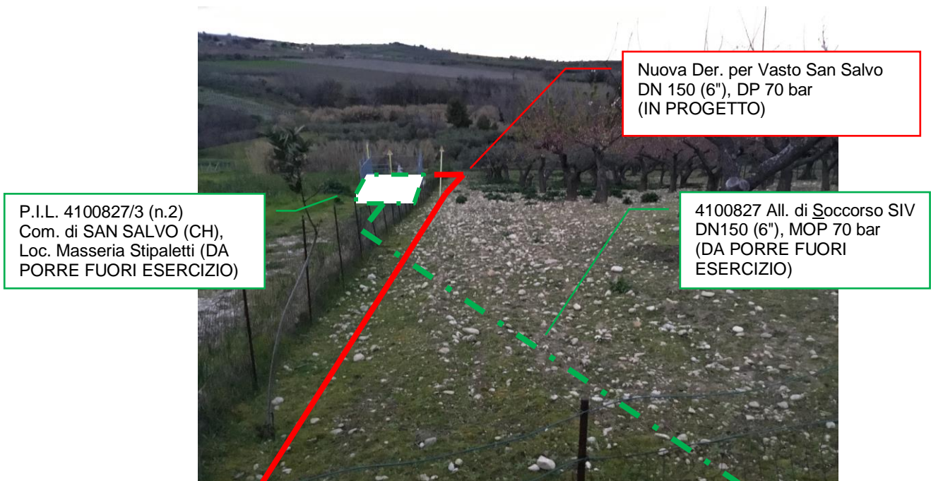
Foto n.13 – Km 0+970 - Vista met. da porre fuori esercizio, in progetto e impianto PIL da porre fuori esercizio
