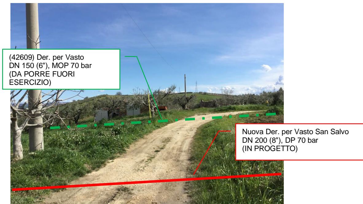
Foto n.9 – Km 2+731 - Vista attraversamento di metanodotti su strada
