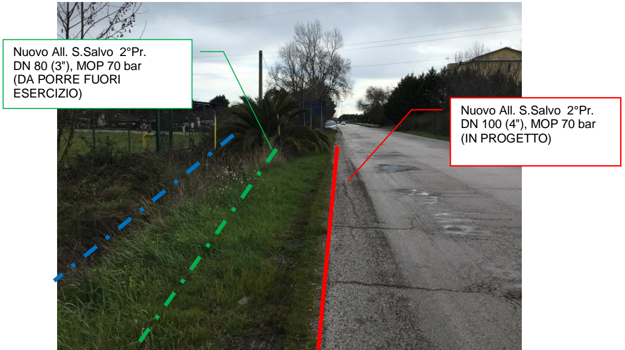
Foto n.24 – Km 2+716 - Panoramica metanodotti su S.P. 197 via Trignina (CH)
