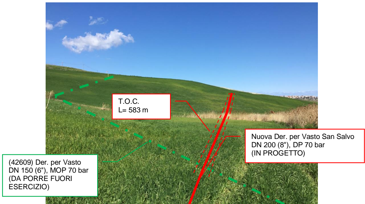
Foto n.7 – Km 0+860 - Metanodotto in progetto con vista T.O.C. e metanodotto da porre fuori esercizio
