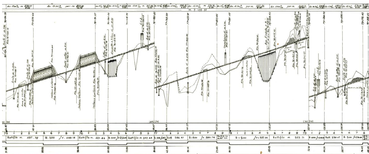
Estratto profilo longitudinale del progetto originale – progr. km 74+990 a 79+850
