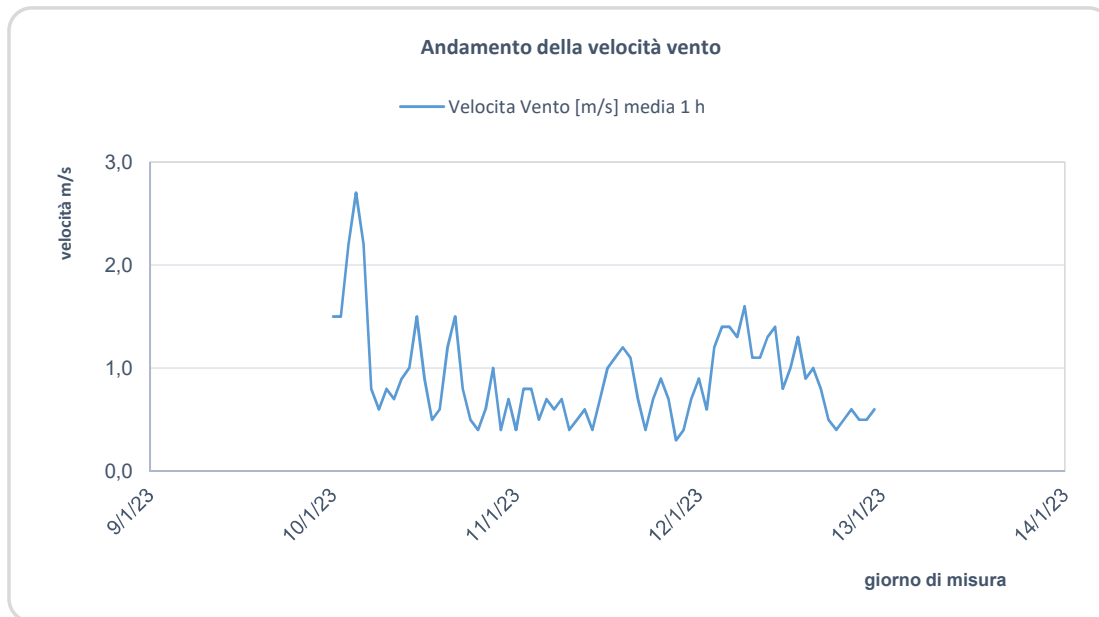
Grafico 8-4: Andamento della velocità del vento
