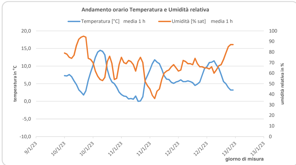
Grafico 8-1: Andamento della temperatura e dell'umidità relativa.
