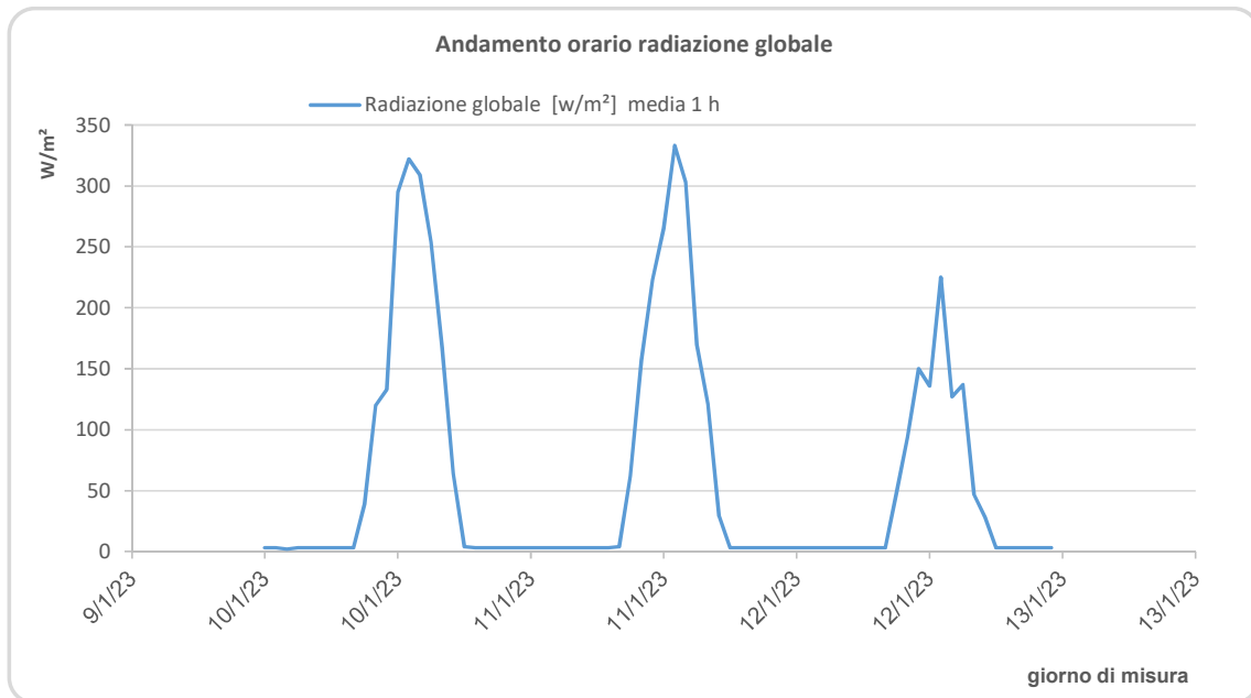
Grafico 8-2: Andamento della radiazione globale.
