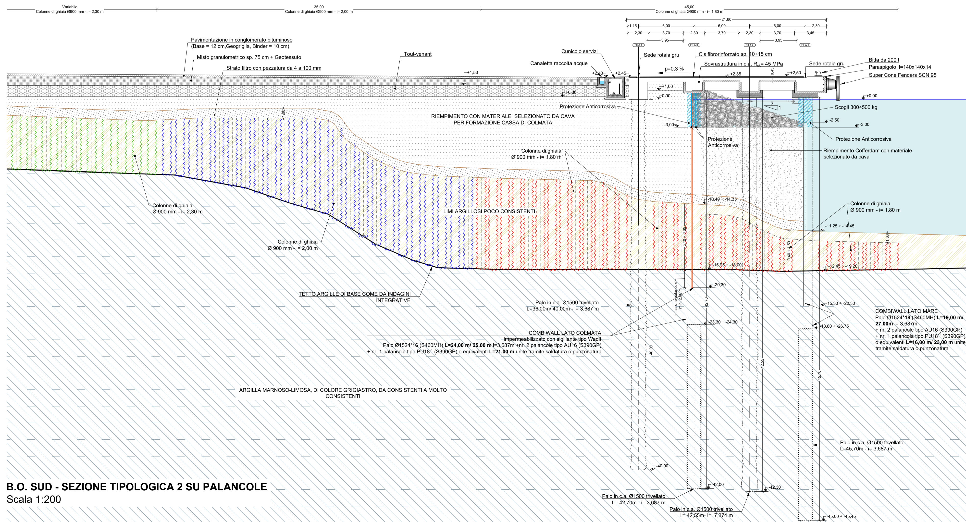
B.O. SUD - SEZIONE TIPOLOGICA 2 SU PALI Scala 1:200
