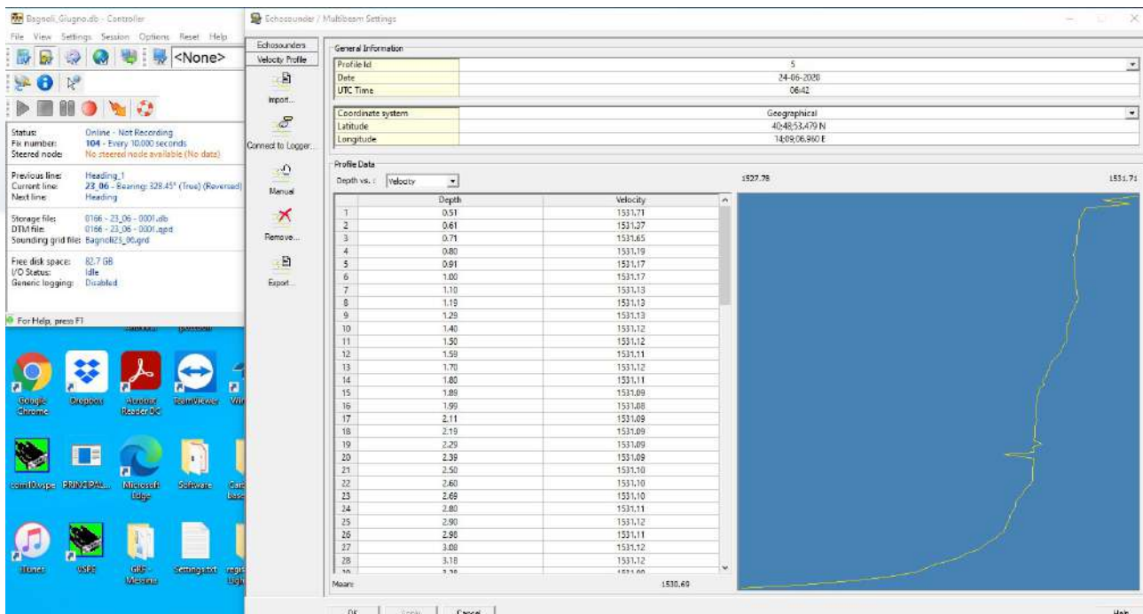
Fig. 7 Registrazione del profilo di velocità del suono in acqua ed inserimento dei dati nel software Idrografico Qinsky (QPS).
