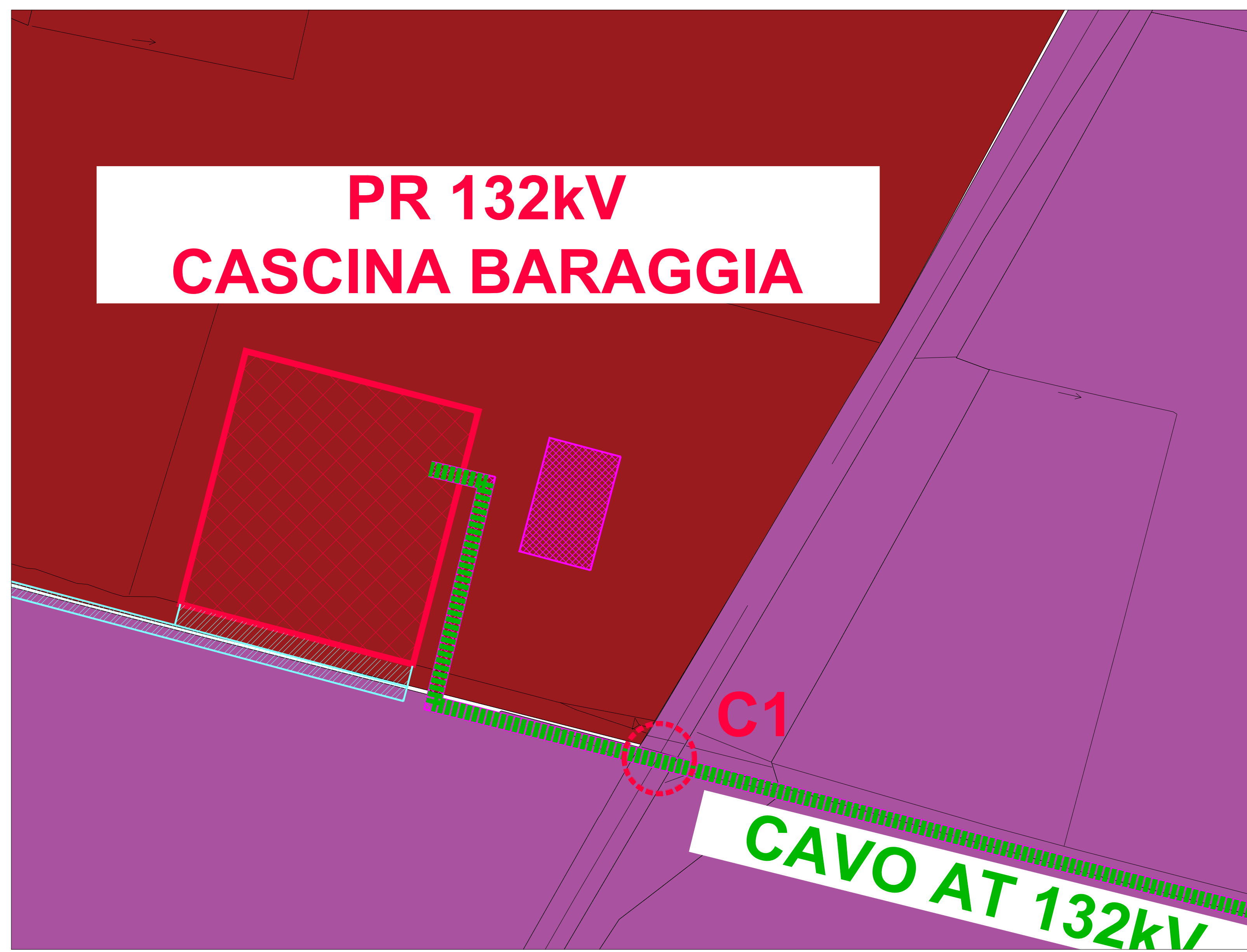
PLANIMETRIA CATASTALE 1:1.000
