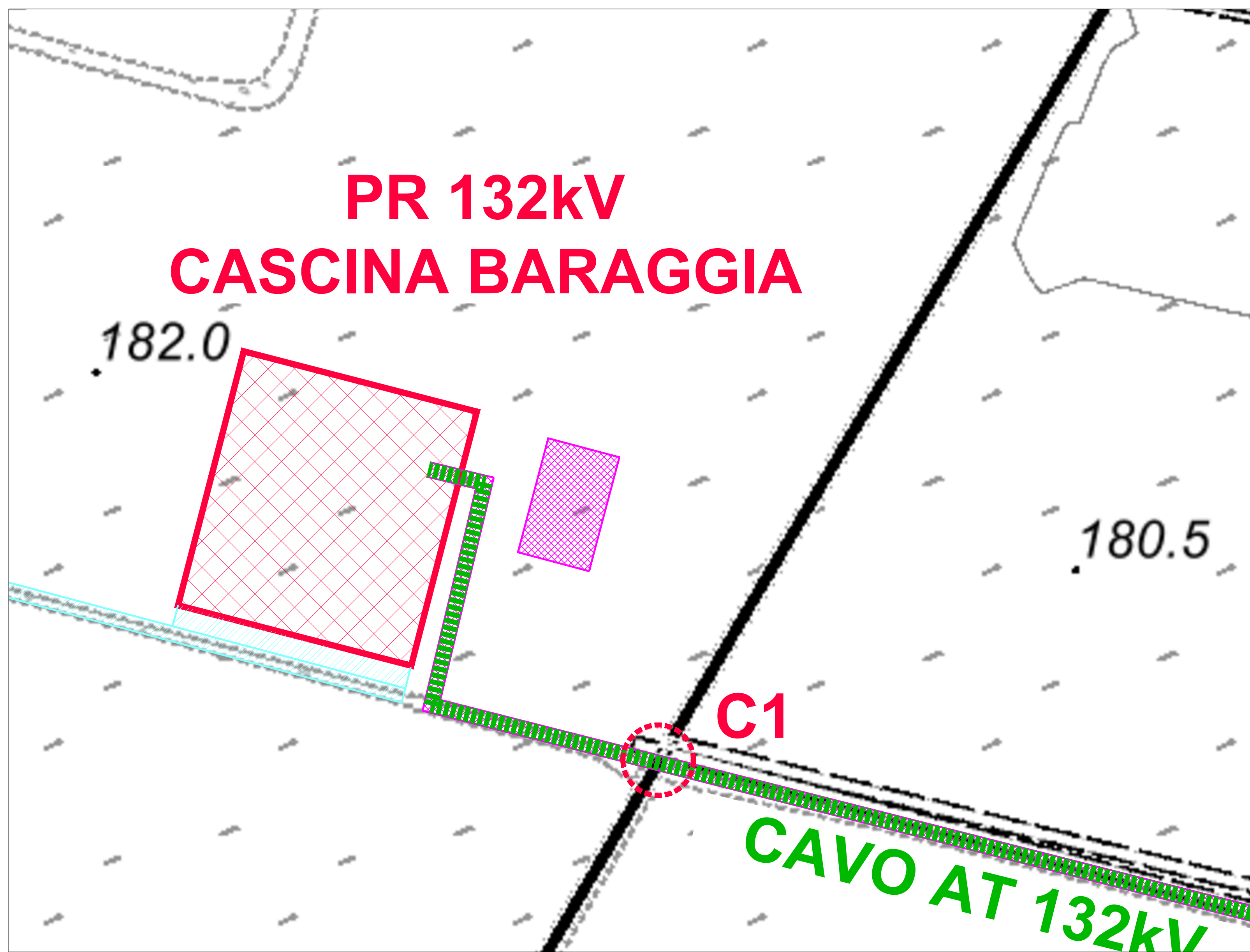
PLANIMETRIA CTR 1:1.000
