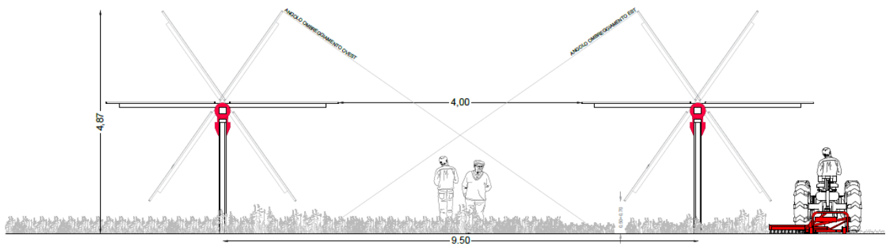
(Sezione tipo del campo agro-fotovoltaico, misure in m)
