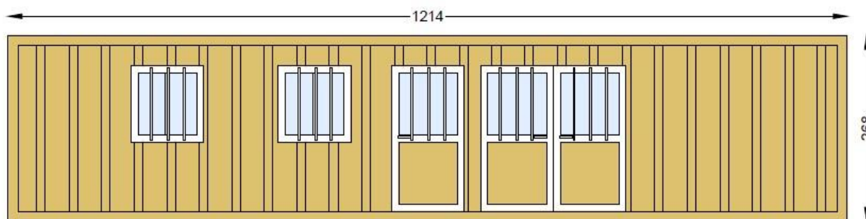
(Configurazione tipica della Control room, misure in cm)
