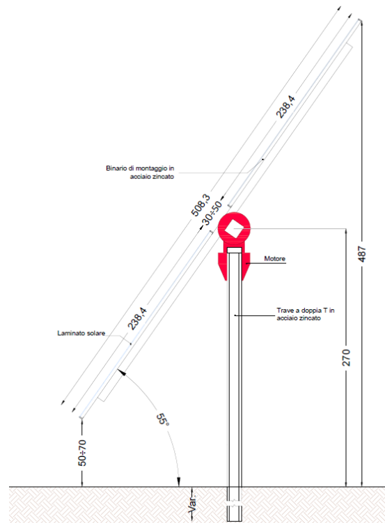
(Sezione tipo di tracker con inclinazione a 55°)
