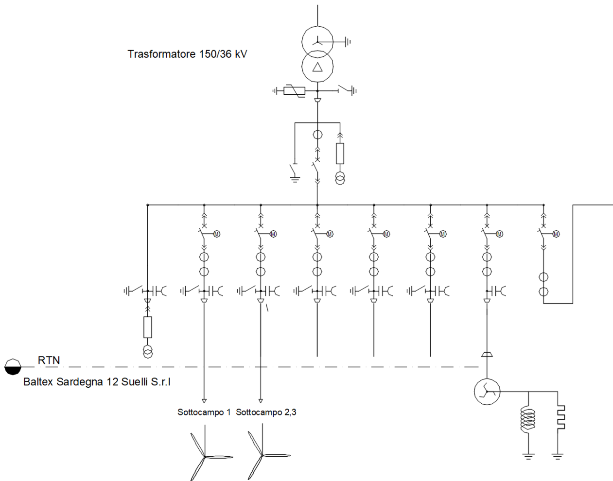
Figura 2-2 – Schema connessione agli stalli di consegna TERNA
