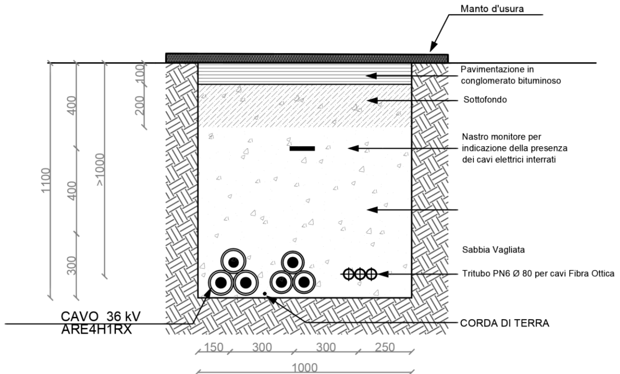
Figura 3-2 – Tipico modalità di posa Cavo 36 kV
