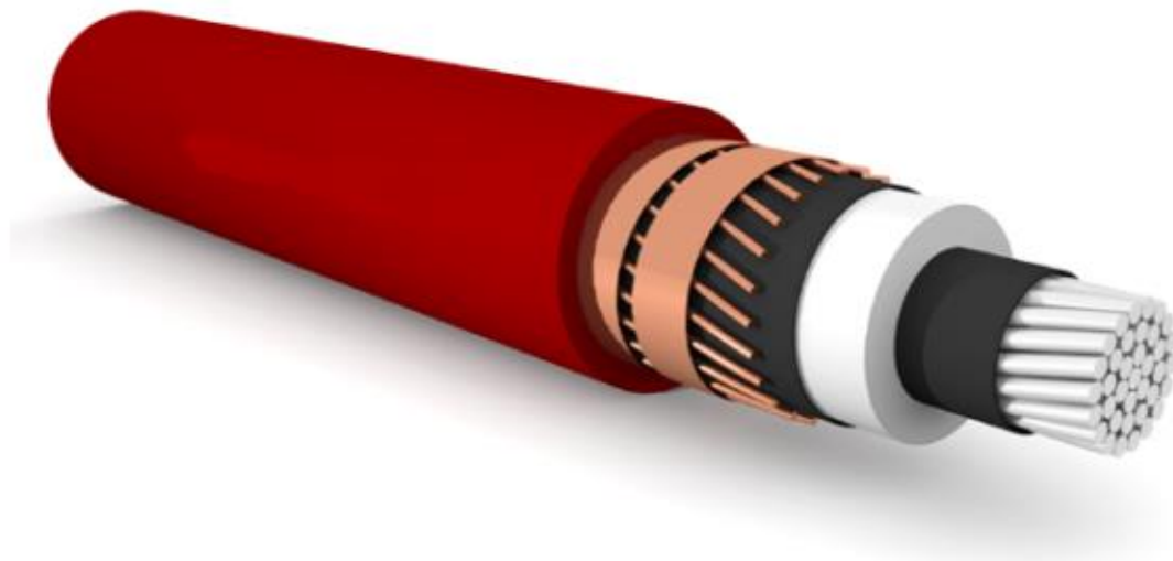
Figura 3-1 - Cavi unipolari del tipo ARE4H1R - 36kV
