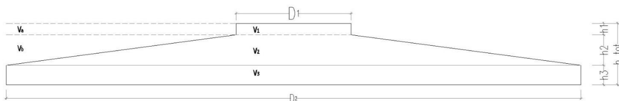
Figura 6.2 - Schema in sezione basamento di fondazione
