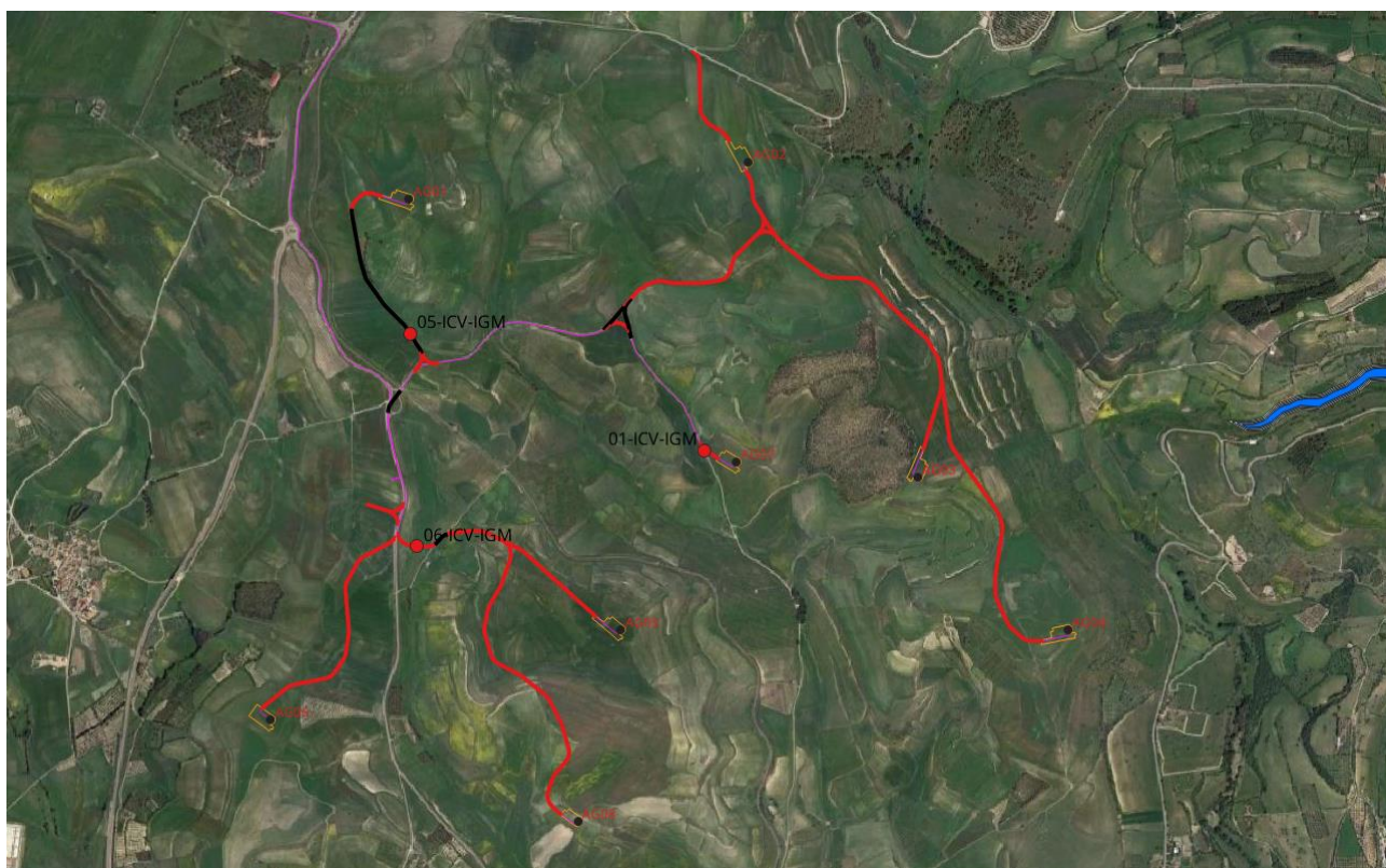
Figura 1.1: Planimetria di progetto su ortofoto con individuazione del reticolo idrografico della Regione (in rosso la viabilità di progetto da realizzare, in nero la viabilità da adeguare)
