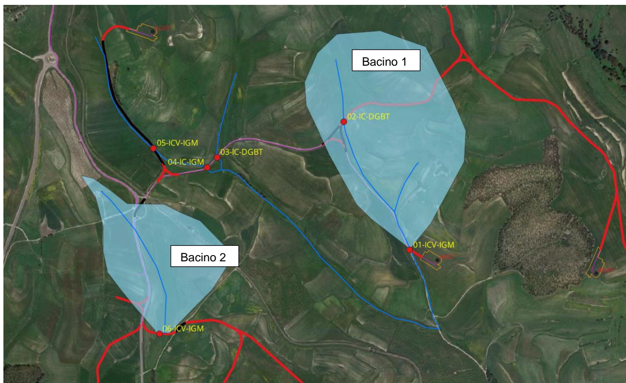
Figura 4.1: Planimetria con individuazione del bacino idrografico dell'attraversamento 01-ICV-IGM e 06-ICV-IGM
