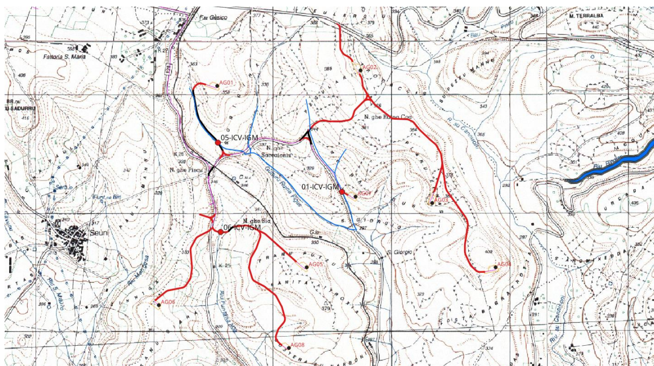
Figura 1.2: Planimetria di progetto su IGM con individuazione del reticolo idrografico della Regione Sardegna (in rosso la viabilità di progetto da realizzare, in nero la viabilità da adeguare)
