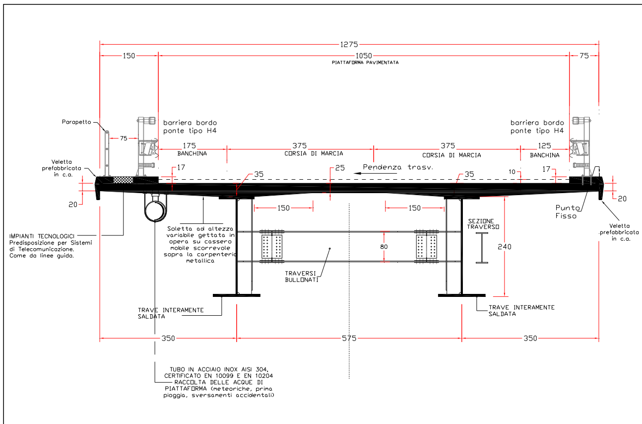
Sezione trasversale d'impalcato (carreggiata sx).
