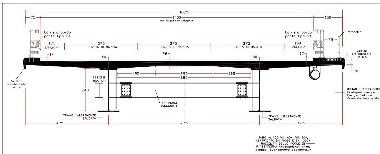
Sezione trasversale d'impalcato (carreggiata dx).
