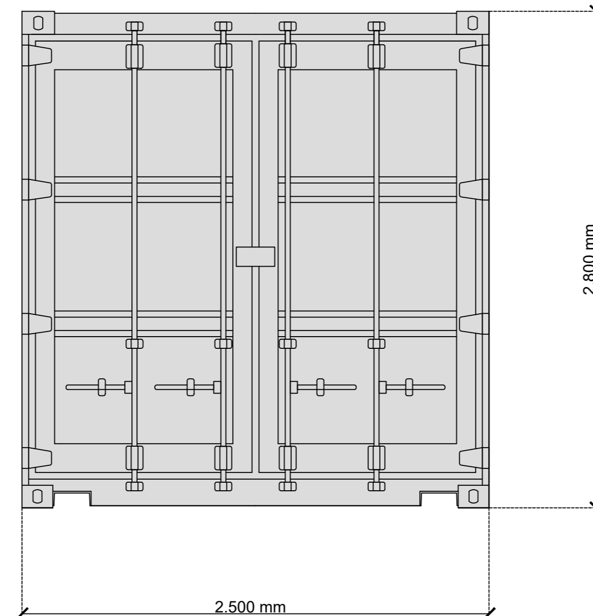
PROSPETTO FRONTALE SC - SCALA 1:20
