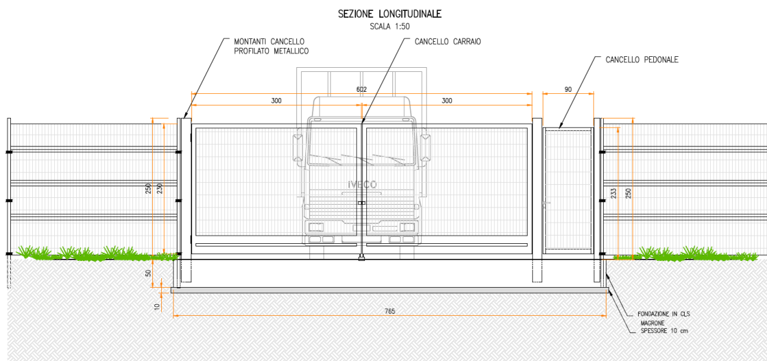
Figura 12.6: Particolare accesso
