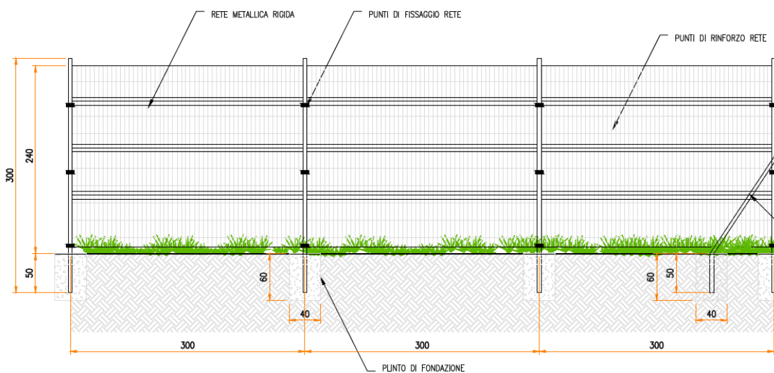
Figura 12.5: Particolare recinzione
