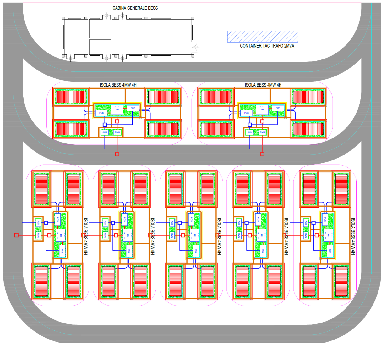
Figura 2.4: Layout del Sistema BESS 25 MW – 4h
