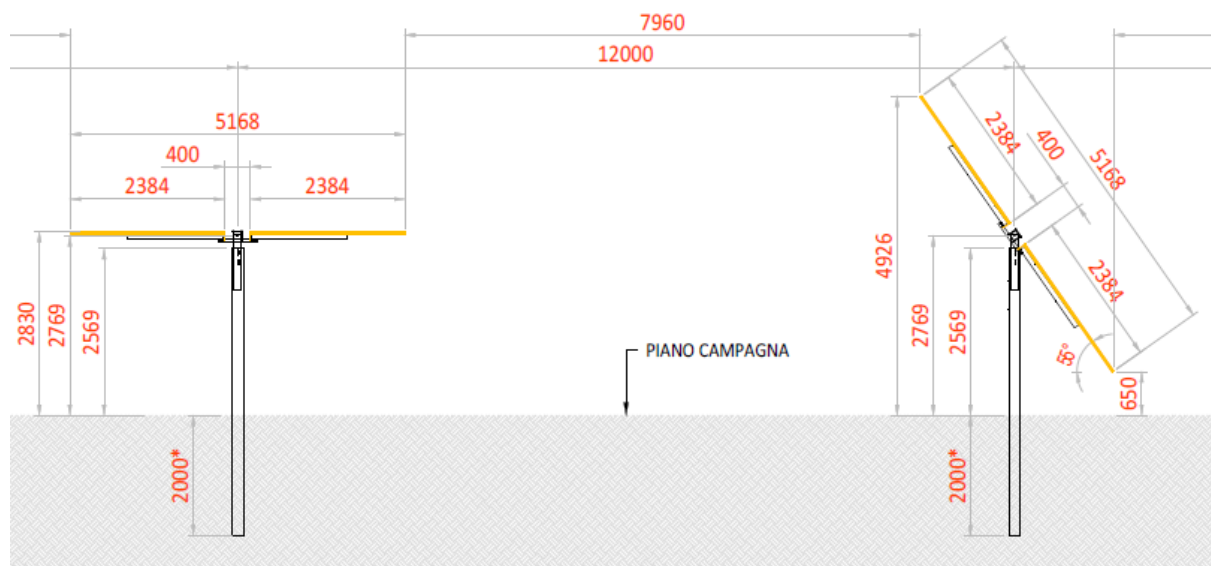
Figura 12.2: Particolare costruttivo strutture mobili (tracker)
