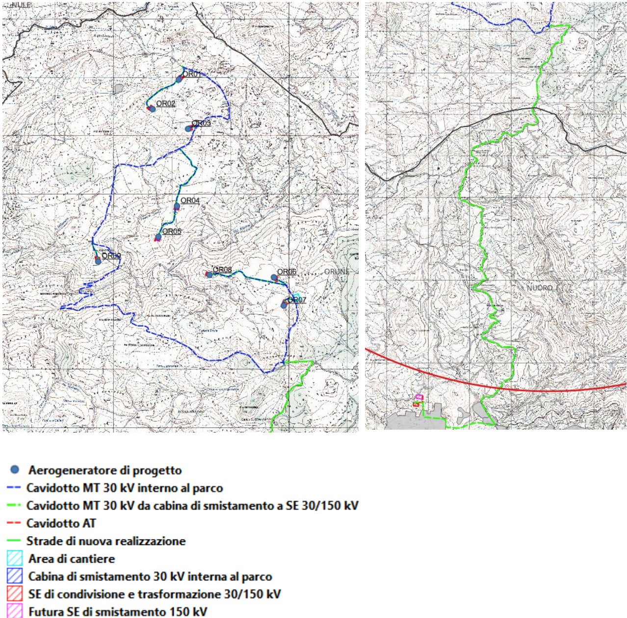
Figura 1: Layout dell'impianto e localizzazione
