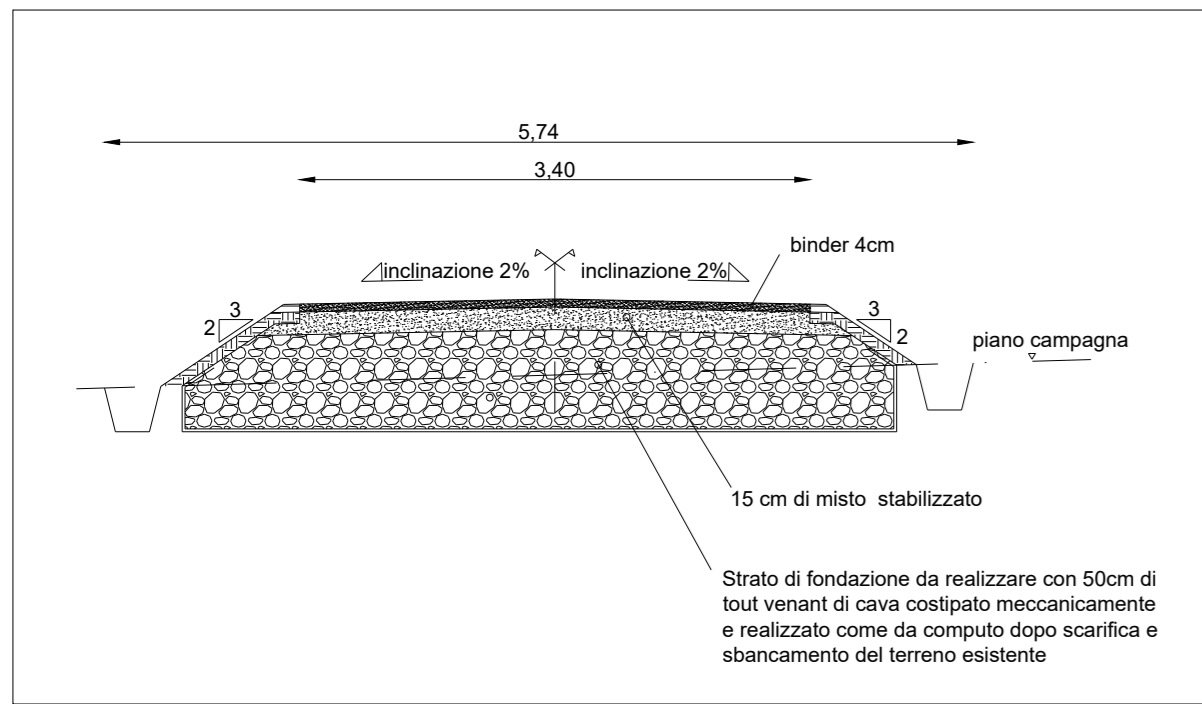
Sezione pacchetto stradale scala 1:50
