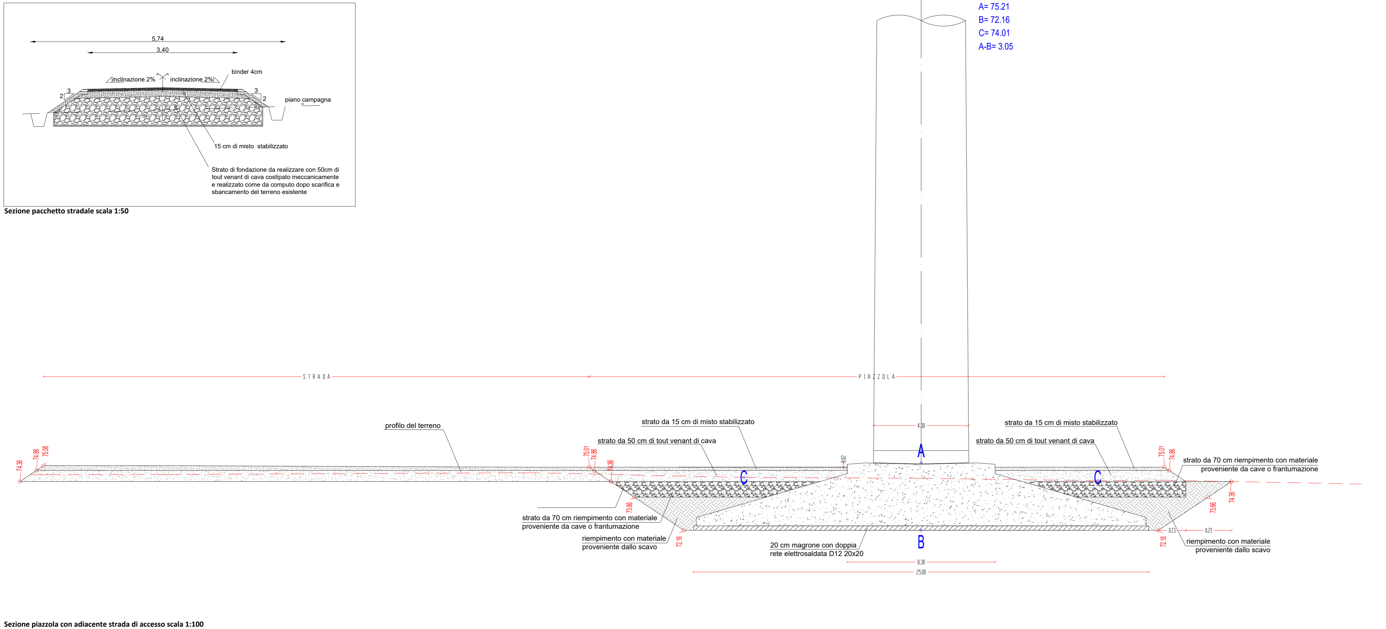
Sezione piazzola con adiacente strada di accesso scala 1:100
